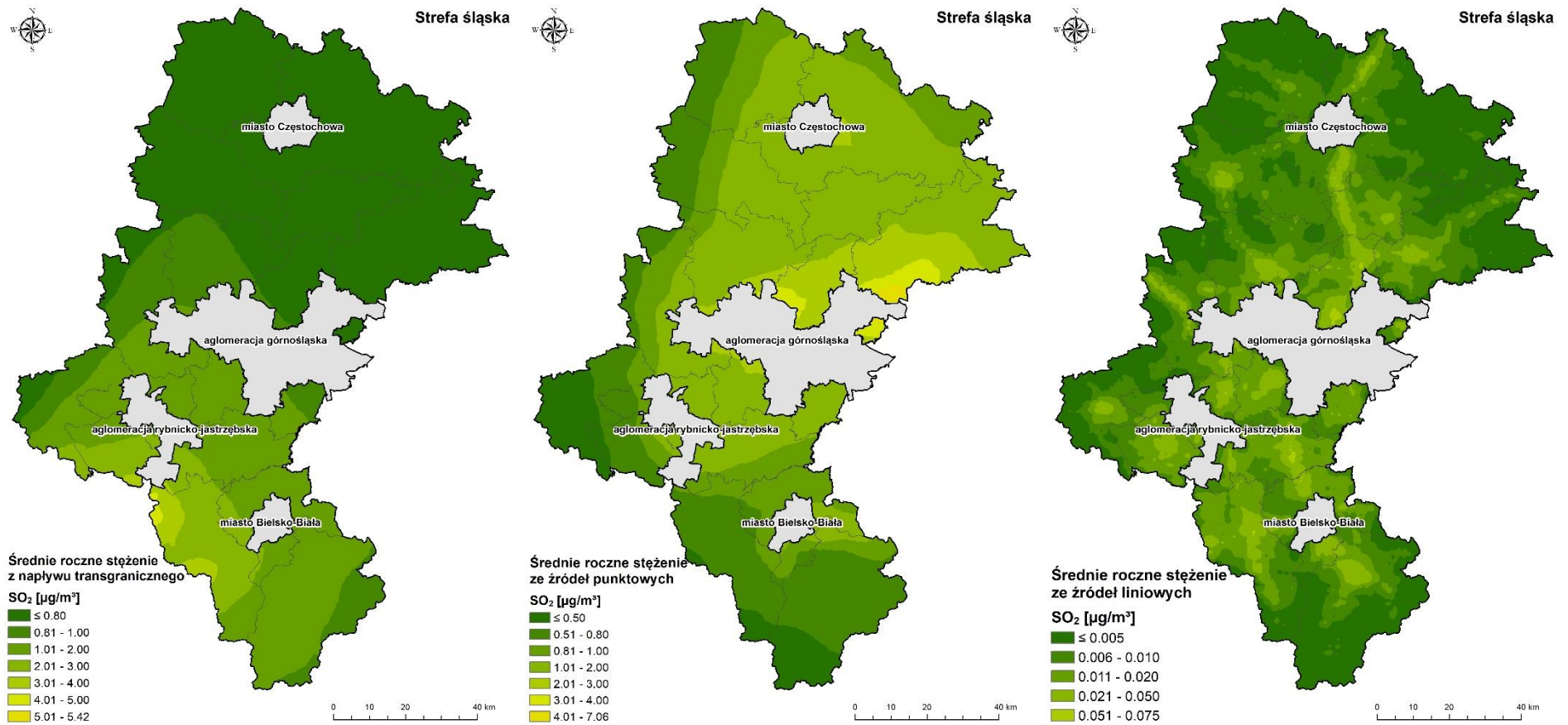
Rysunek 22. Rozkład stężeń średniorocznych SO 2 generowanych przez napływ transgraniczny, napływ z innych stref województwa śląskiego ze źródeł liniowych w strefie śląskiej 61
