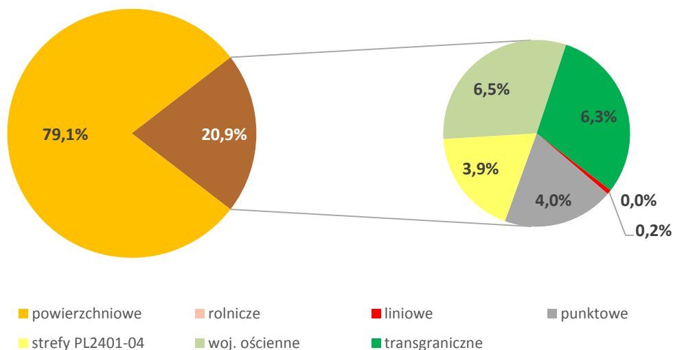
Rysunek 19. Udziały poszczególnych rodzajów źródeł emisji w wielkości stężeń średniorocznych dwutlenku siarki w obszarze przekroczeń stężeń dobowych na terenie strefy śląskiej 59
