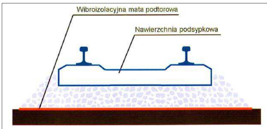
Rysunek 7. Schemat zastosowania maty wibroizolacyjnej [Źródło: www.tines.pl ].
