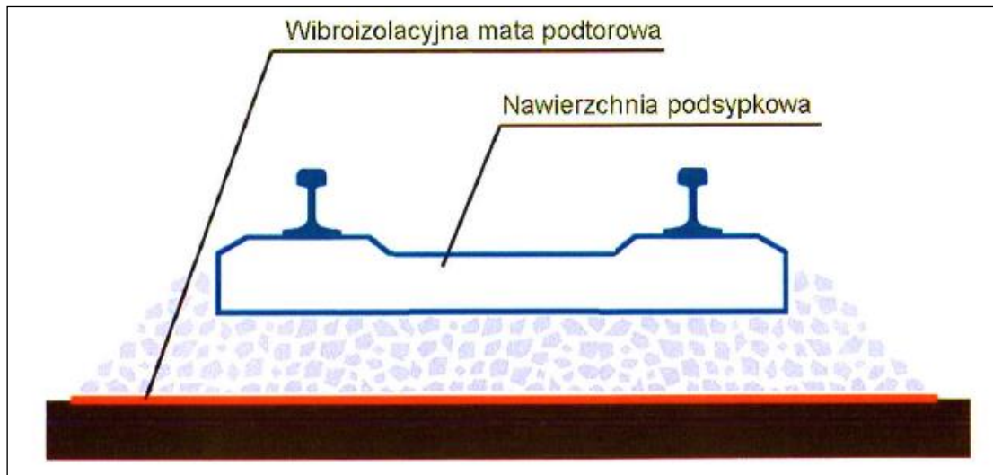
Rysunek 7. Schemat zastosowania maty wibroizolacyjnej
