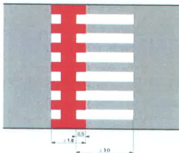
Rys. 4.2.2.3. Przykład sposobu połączenia znaku P-10 ze znakiem P-11",
