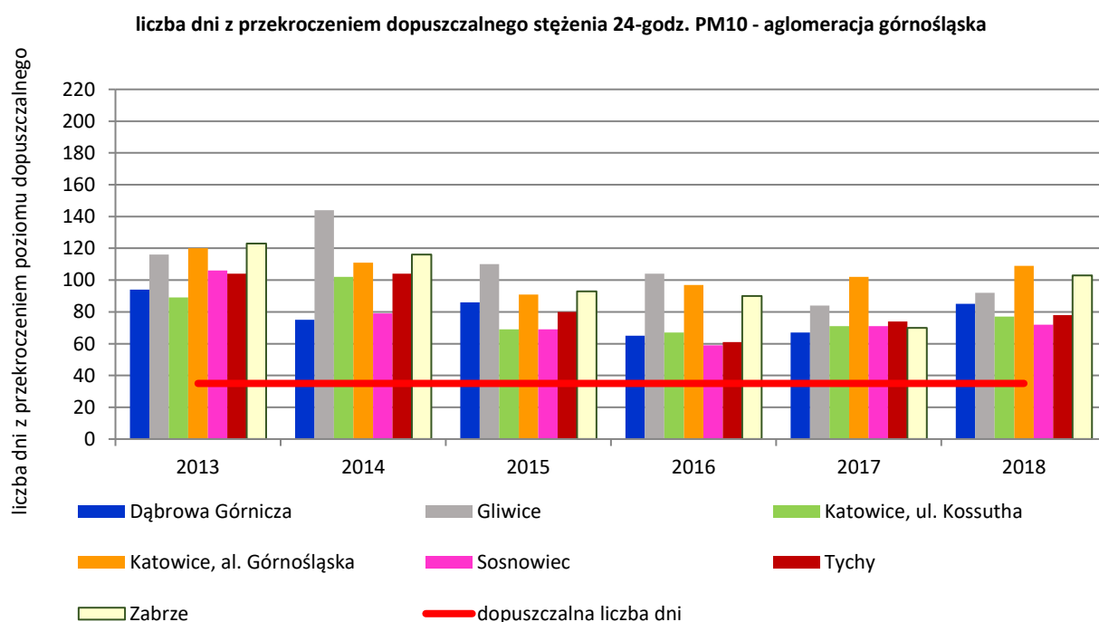
Rysunek 16. Liczba dni z przekroczeniem poziomu dopuszczalnego 24-godzinnego pyłu zawieszonego PM10 w latach 2013-2018 w punktach pomiarowych w strefie aglomeracja górnośląska 76
