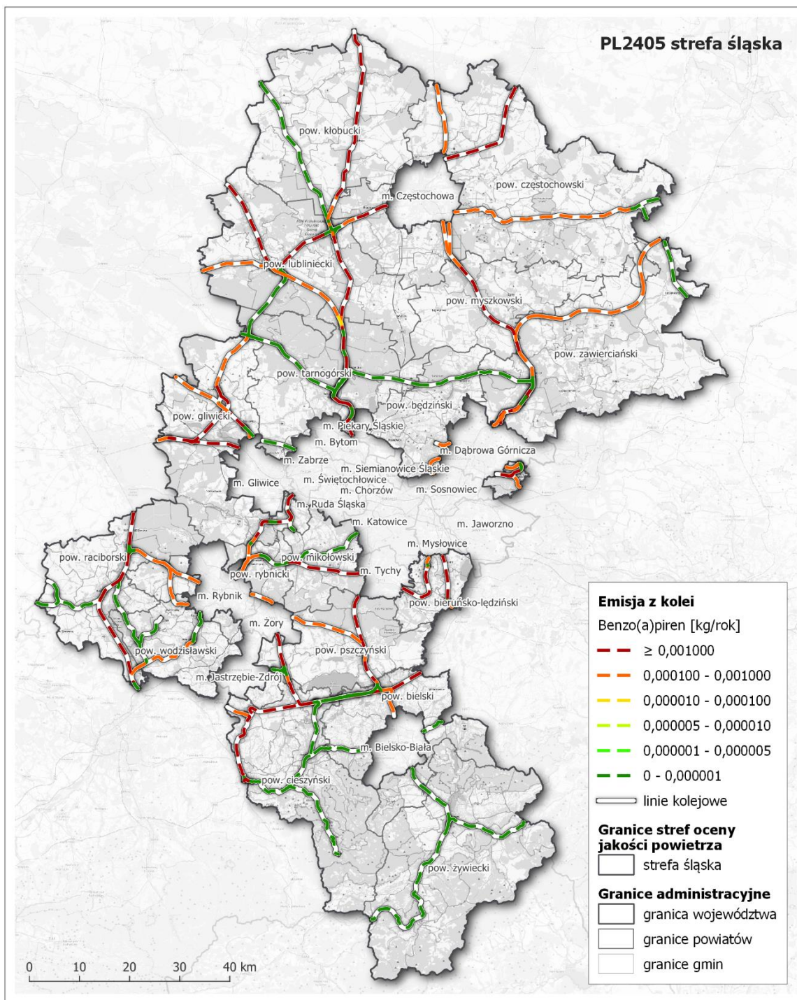
Rysunek 195. Lokalizacja i wielkość emisji B(a)P z kolei w strefie śląskiej w roku bazowym 2018 356
