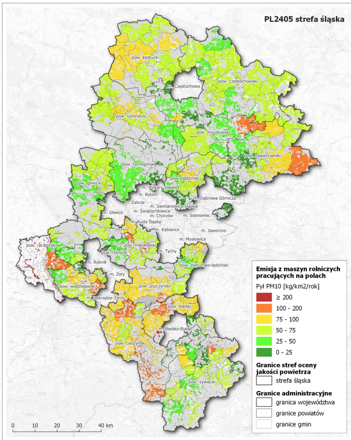
Rysunek 198. Lokalizacja i wielkość emisji pyłu PM10 z maszyn rolniczych w strefie śląskiej w roku bazowym 2018 359
