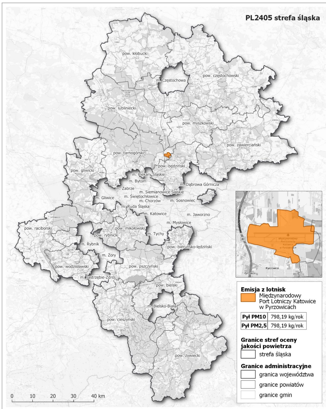
Rysunek 203. Lokalizacja i wielkość emisji pyłu PM 2,5 z lotnisk w strefie śląskiej w roku bazowym 2018 364
