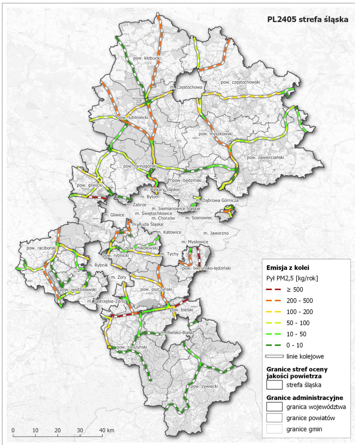
Rysunek 194. Lokalizacja i wielkość emisji pyłu PM 2,5 z kolei w strefie śląskiej w roku bazowym 2018 355
