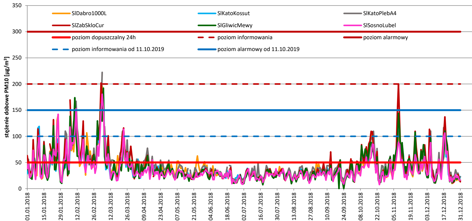
przebieg zmienności stężeń 24-godz. PM10 w 2018 r. - aglomeracja górnośląska
