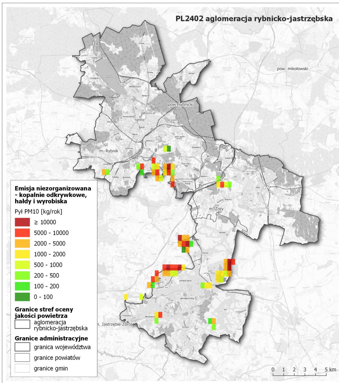
Rysunek 143. Lokalizacja i wielkość emisji pyłu PM10 ze źródeł niezorganizowanych (kopalnie odkrywkowe, haldy i wyrobiska) w aglomeracji rybnicko-jastrzębskiej w roku bazowym 2018 304
