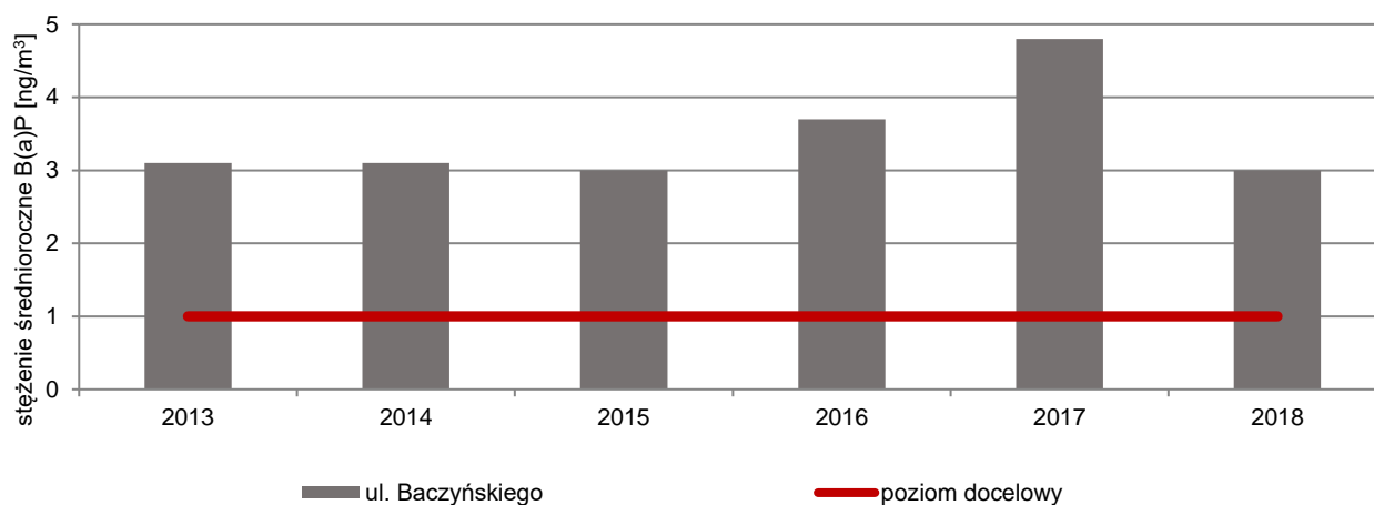
Rysunek 39. Wyniki pomiarów stężeń średniorocznych benzo(a)pirenu w latach 2013-2018 w strefie miasto Częstochowa 127
