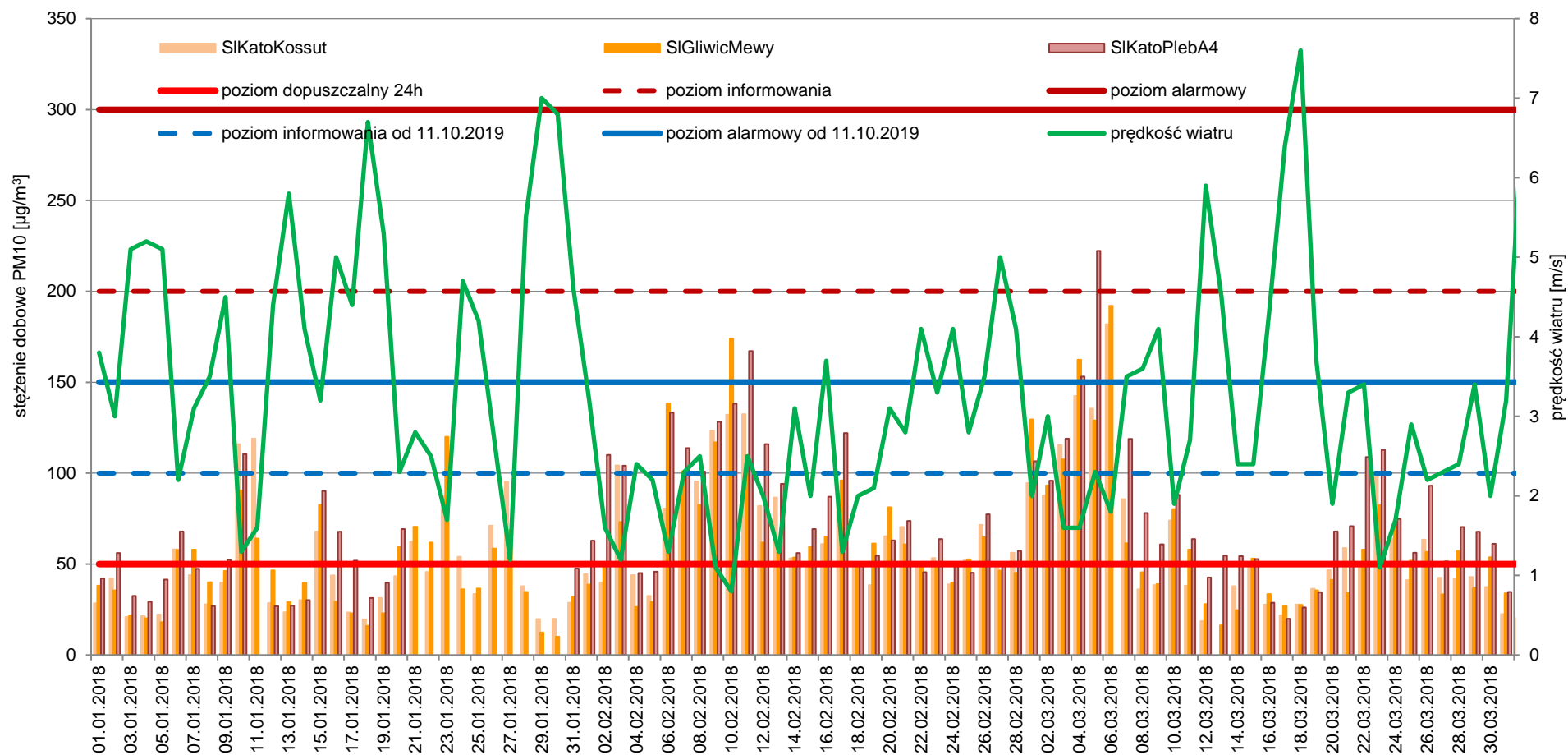
porównanie przebiegu zmienności stężeń 24-godz. PM10 w 2018 r. w aglomeracji górnośląskiej z prędkością wiatru
