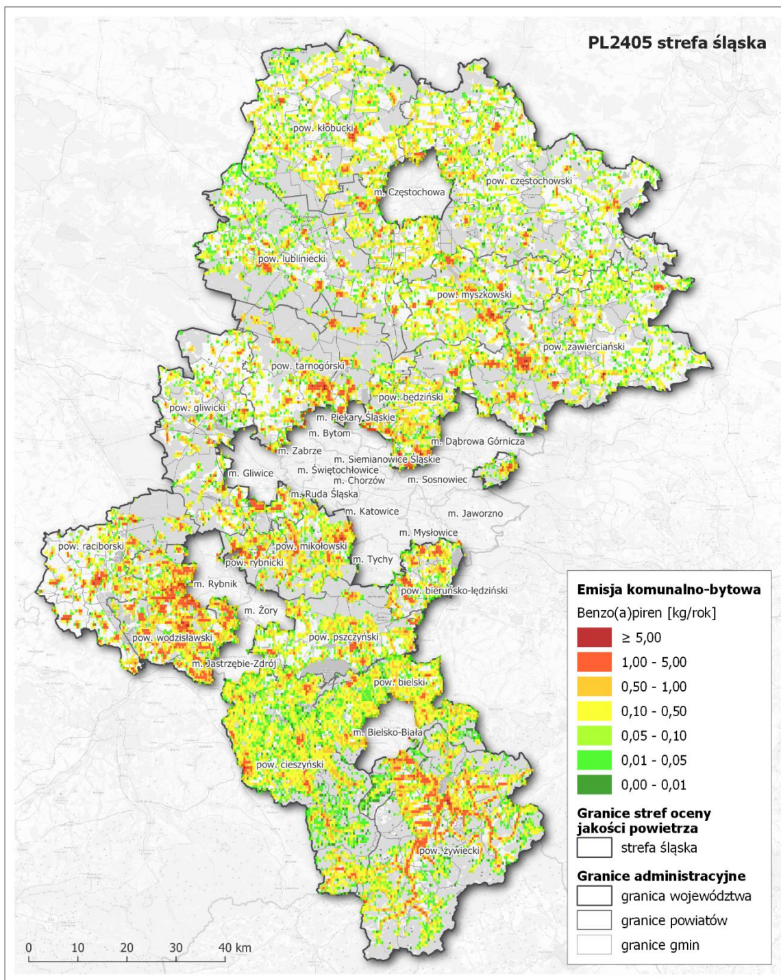
Rysunek 226. Lokalizacja i wielkość emisji B(a)P ze źródeł z sektora komunalno-bytowego w strefie śląskiej w roku bazowym 2018 387
