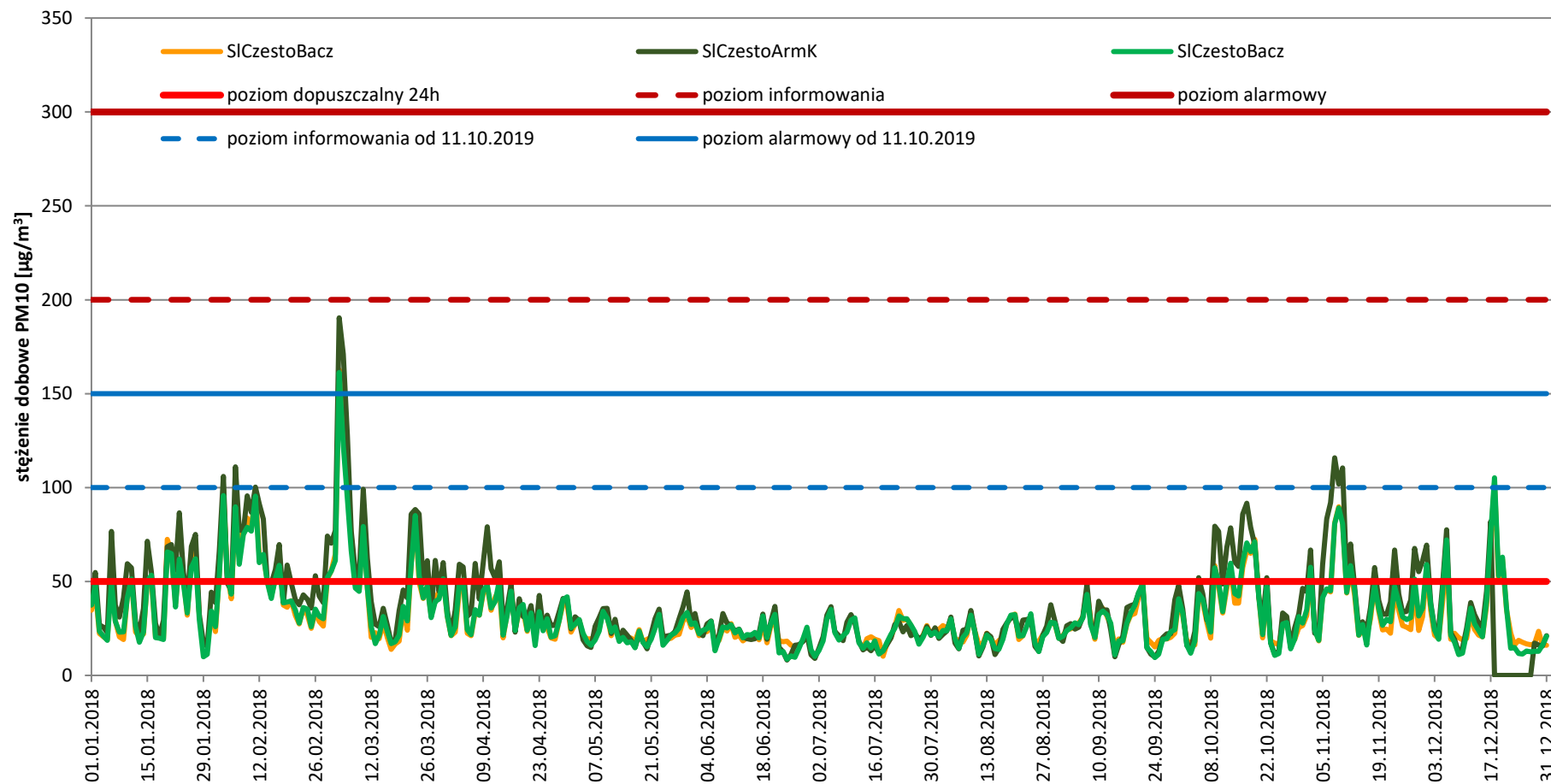
przebieg zmienności stężeń 24-godz. PM10 w 2018 r. - Częstochowa
