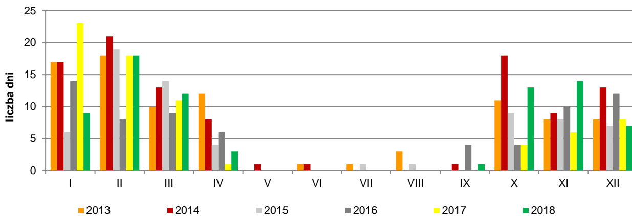
liczba dni z przekroczeniem dopuszczalnego stężenia 24-godz. dla PM10 w Katowicach ul. Kossutha
