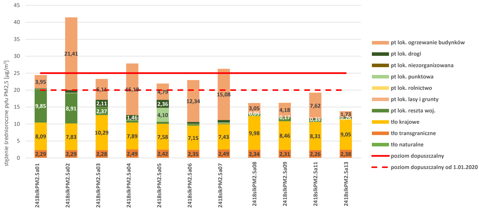
Rysunek 89. Prezentacja poziomów tła regionalnego oraz lokalnego przyrostu stężeń na terenie obszarów przekroczeń pyłu PM 2,5 w strefie śląskiej w 2018 roku 194
