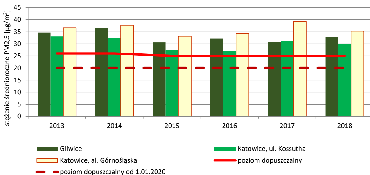
stężenie średnioroczne PM2,5 w strefie aglomeracja górnośląska
