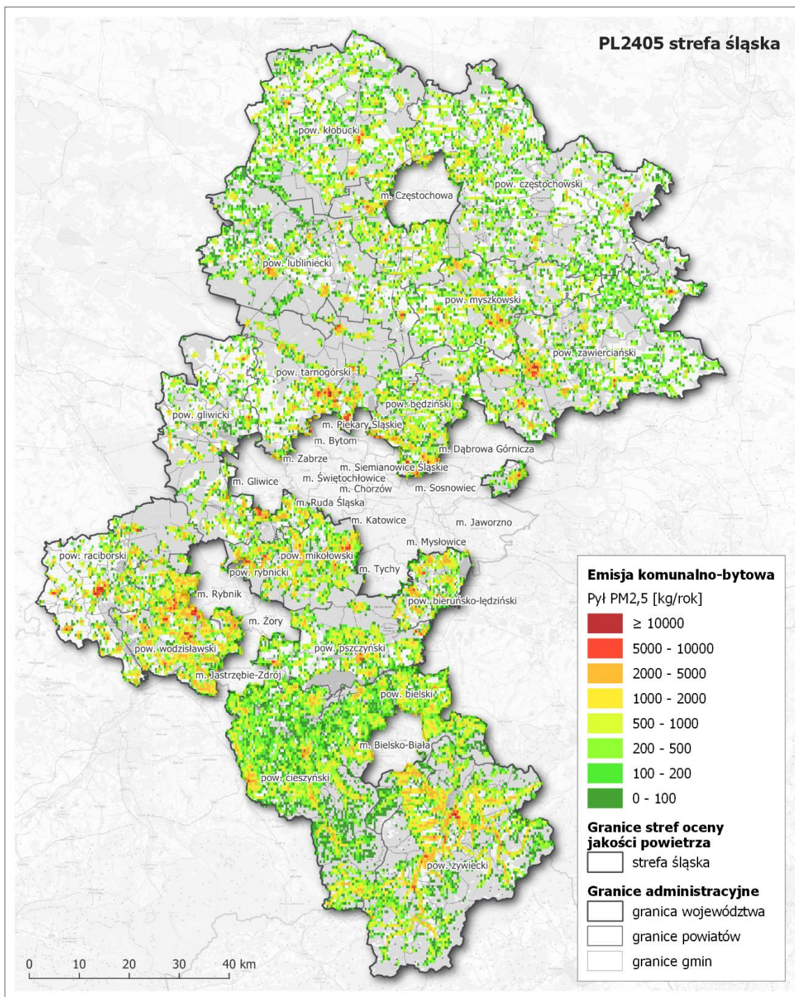
Rysunek 225. Lokalizacja i wielkość emisji pyłu PM 2,5 ze źródeł z sektora komunalno-bytowego w strefie śląskiej w roku bazowym 2018 386
