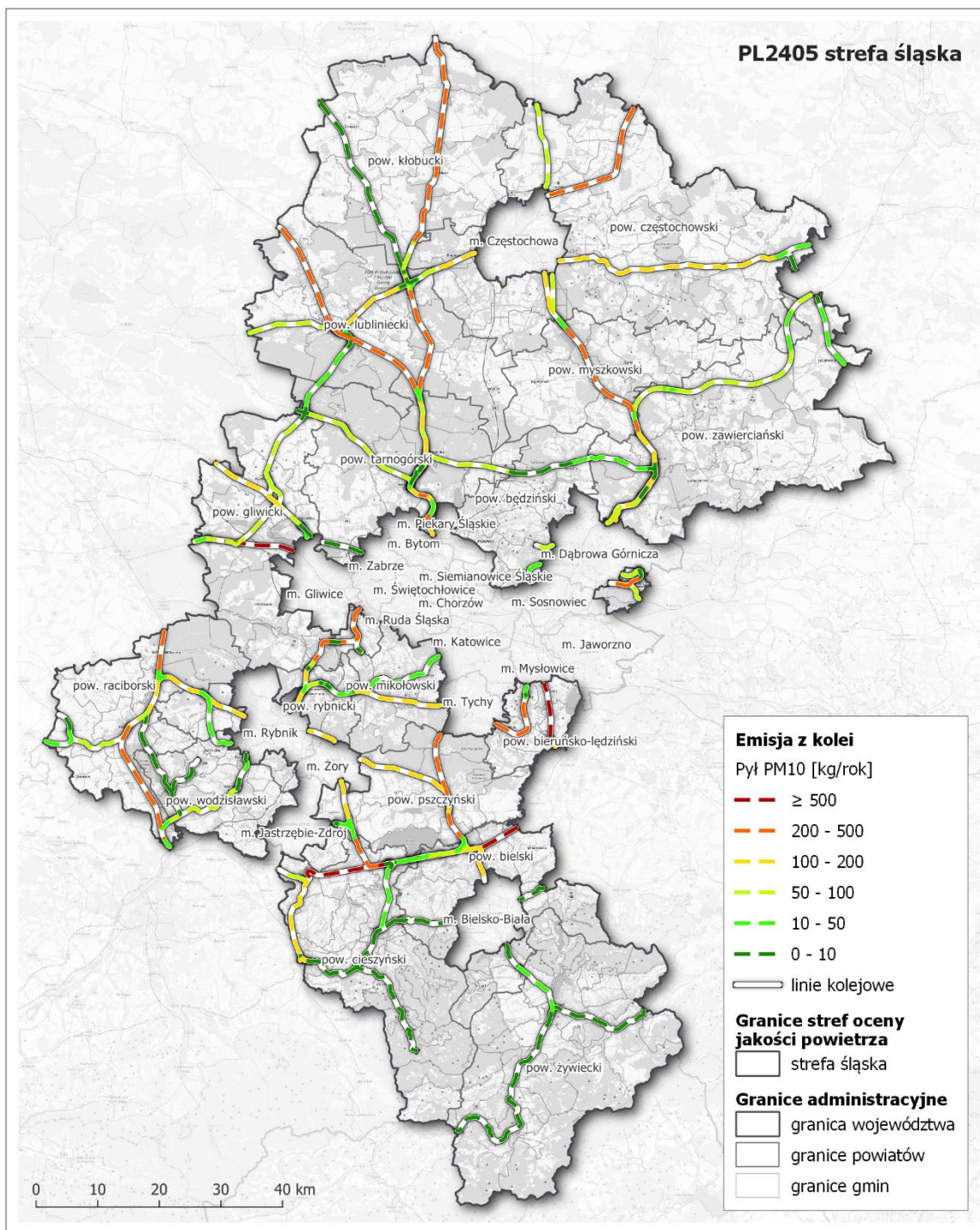
Rysunek 193. Lokalizacja i wielkość emisji pyłu PM10 z kolei w strefie śląskiej w roku bazowym 2018 354
