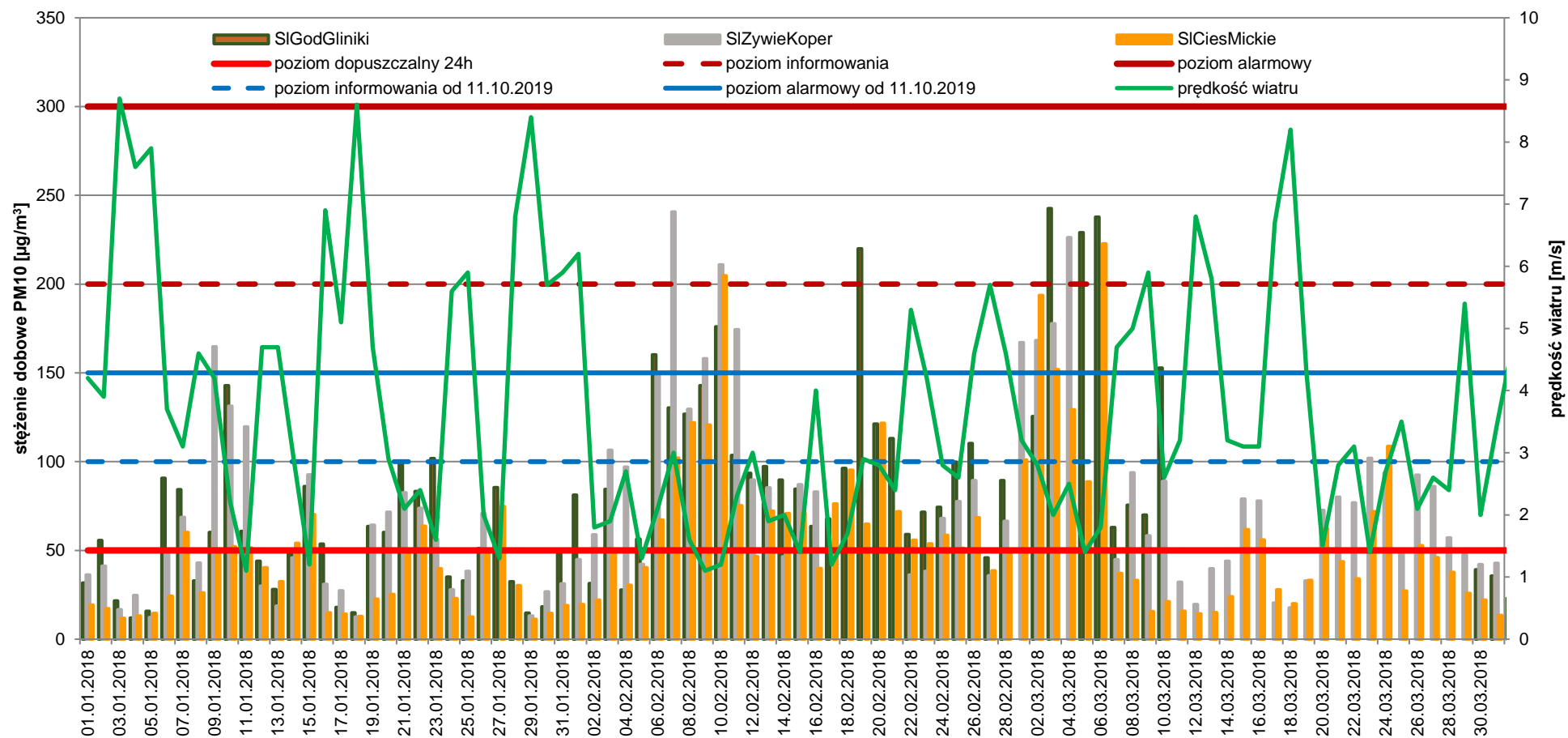
porównanie przebiegu zmienności stężeń 24-godz. PM10 w 2018 r. w strefie śląskiej z prędkością wiatru
