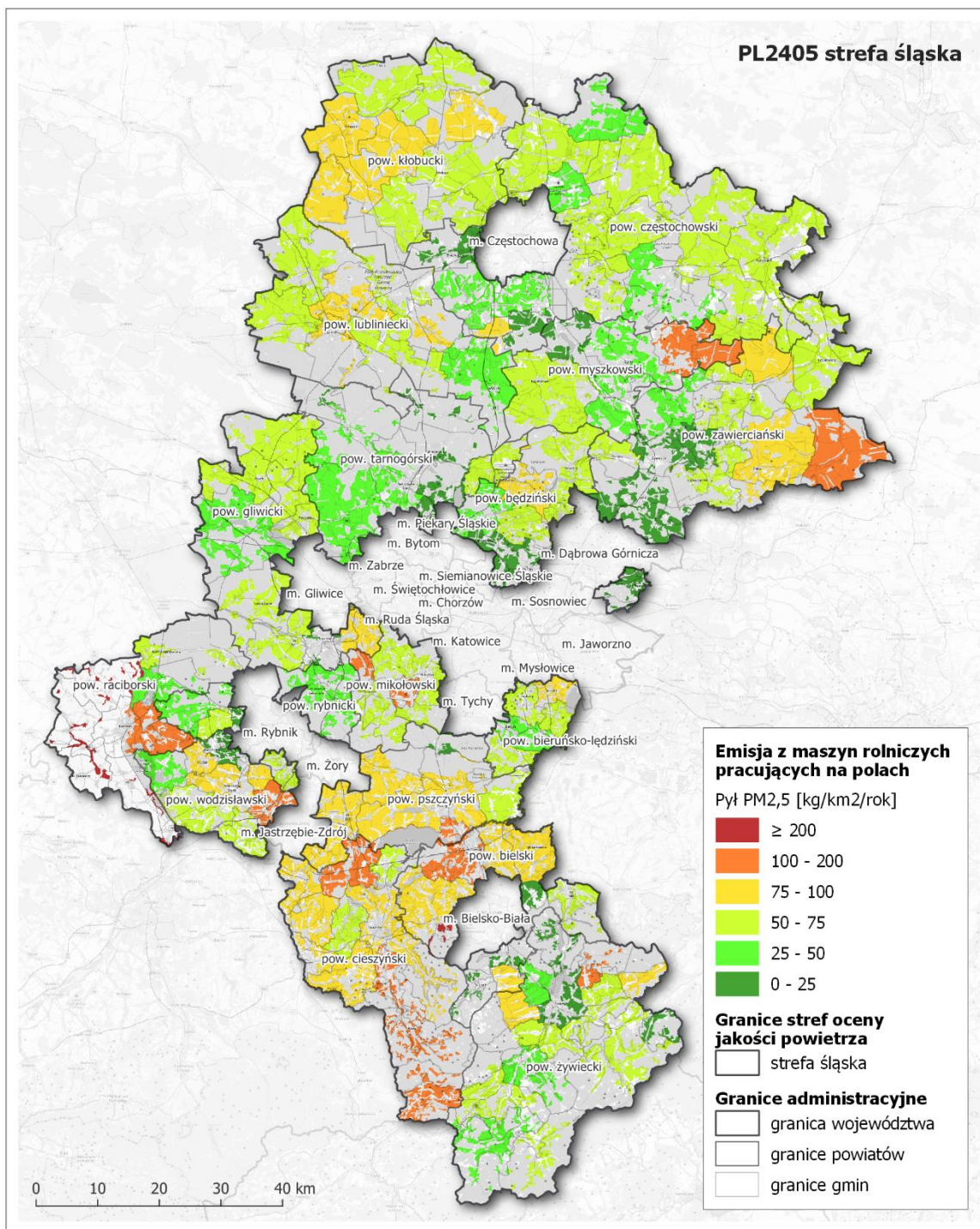
Rysunek 199. Lokalizacja i wielkość emisji pyłu PM 2,5 z maszyn rolniczych w strefie śląskiej w roku bazowym 2018 360
