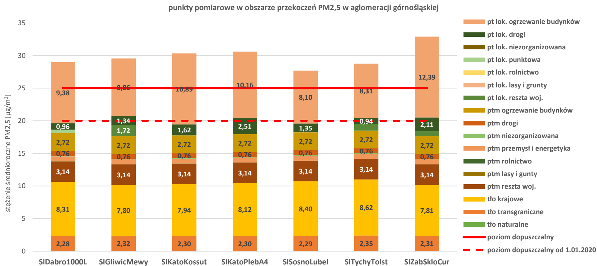
Rysunek 74. Prezentacja poziomów tła regionalnego, przyrostu tła miejskiego oraz lokalnego przyrostu stężeń w punktach pomiarowych na terenie obszaru przekroczeń pyłu PM2,5 w aglomeracji górnośląskiej w 2018 roku 179
