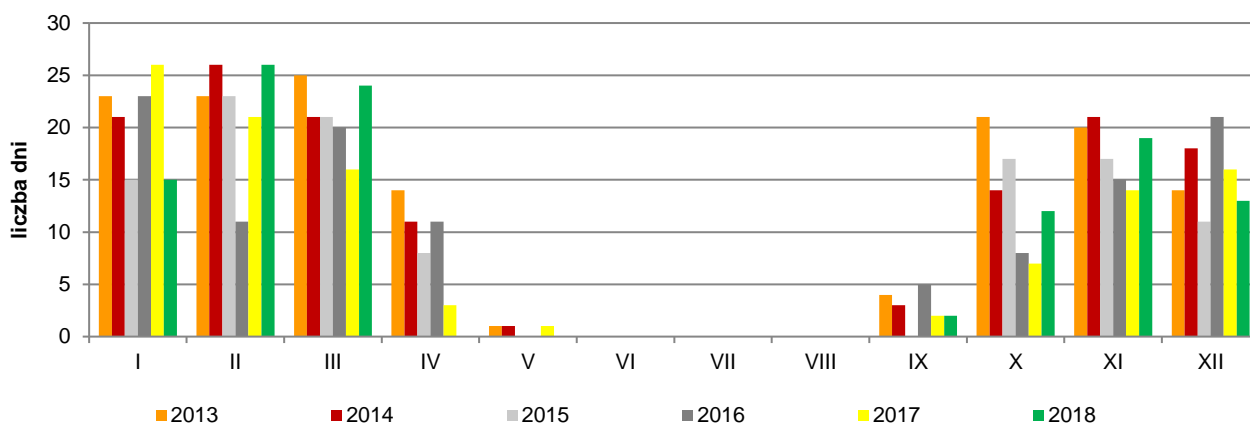
liczba dni z przekroczeniem dopuszczalnego stężenia 24-godz. dla PM10 w Wodzisławiu Śląskim
