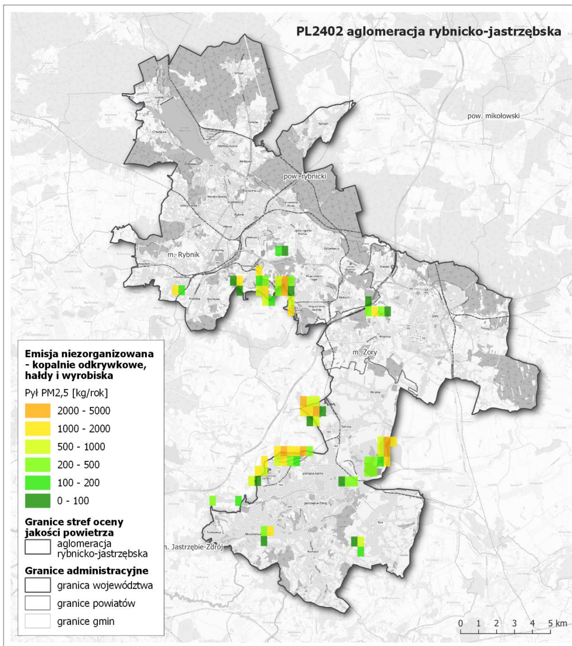
Rysunek 144. Lokalizacja i wielkość emisji pyłu PM 2,5 ze źródeł niezorganizowanych (kopalnie odkrywkowe, haldy i wyrobiska) w aglomeracji rybnicko-jastrzębskiej w roku bazowym 2018 305
