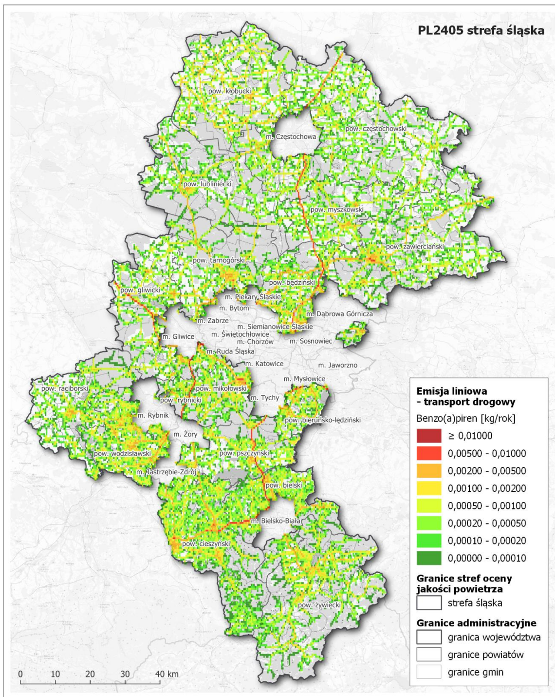
Rysunek 187. Lokalizacja i wielkość emisji B(a)P z sektora transportu drogowego w strefie śląskiej w roku bazowym 2018 348
