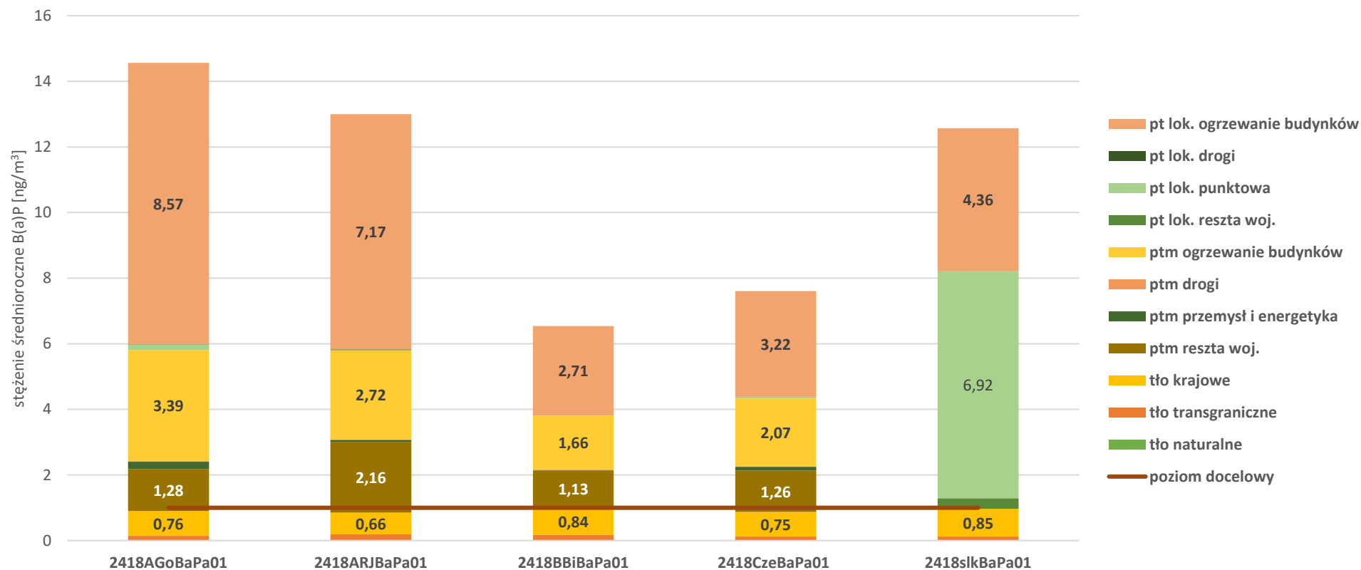
Rysunek 75. Prezentacja poziomów tła regionalnego, przyrostu tła miejskiego oraz lokalnego przyrostu stężeń na terenie obszarów przekroczeń benzo(a)pirenu w województwie śląskim w 2018 roku 180
