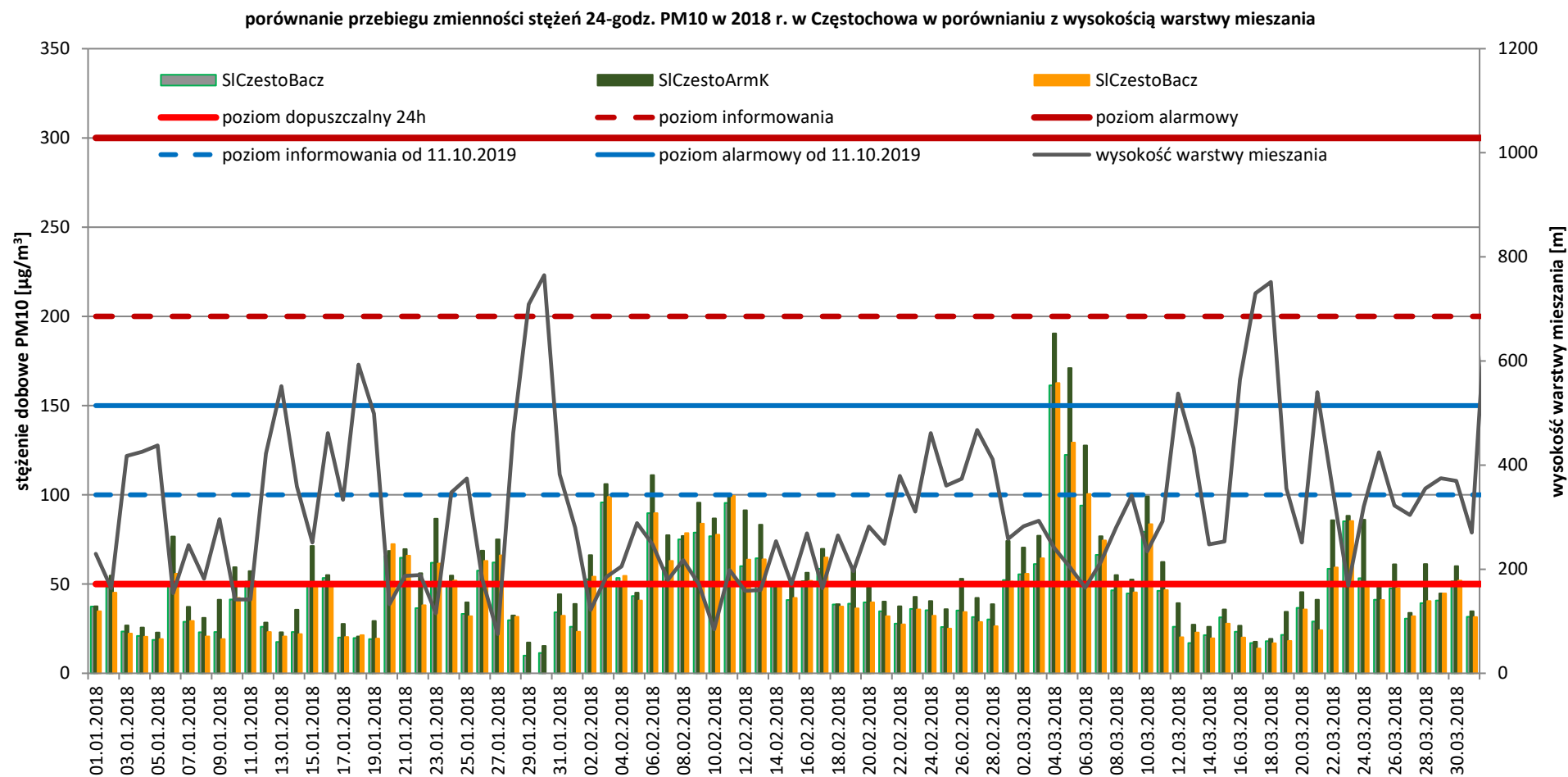
Rysunek 104. Porównanie przebiegu zmienności stężeń 24-godz. PM10 w I kwartale 2018 r. notowanych na stacjach pomiarowych w strefie miasto Częstochowa z wysokością warstwy mieszanania 246
