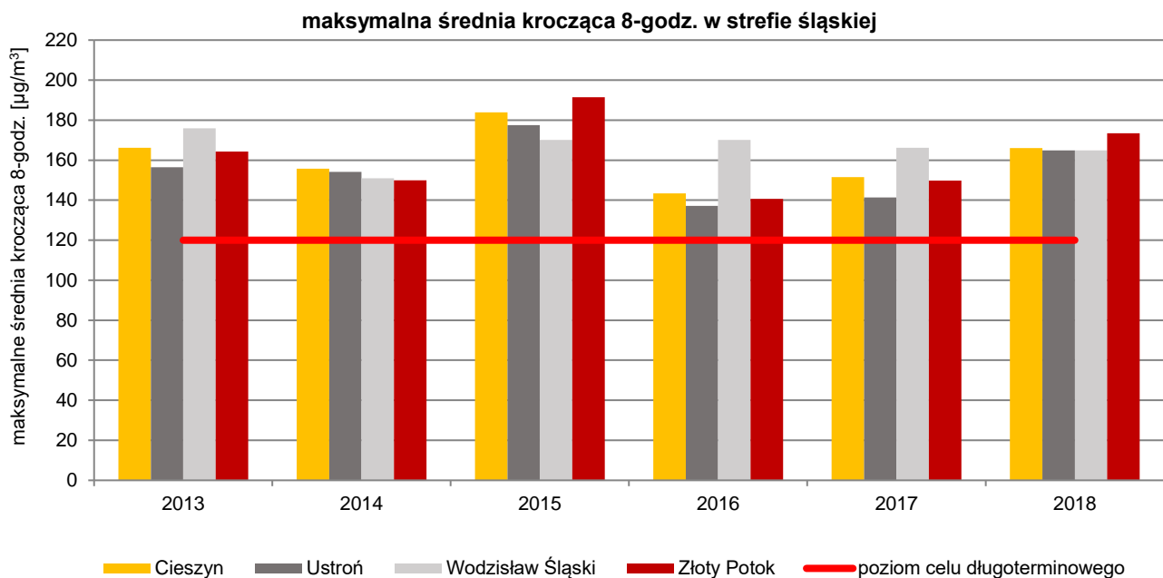
Rysunek 48. Maksymalne ośmiogodzinne średnie kroczące dla ozonu w punktach pomiarowych w latach 2013-2018 w strefie śląskiej 145
