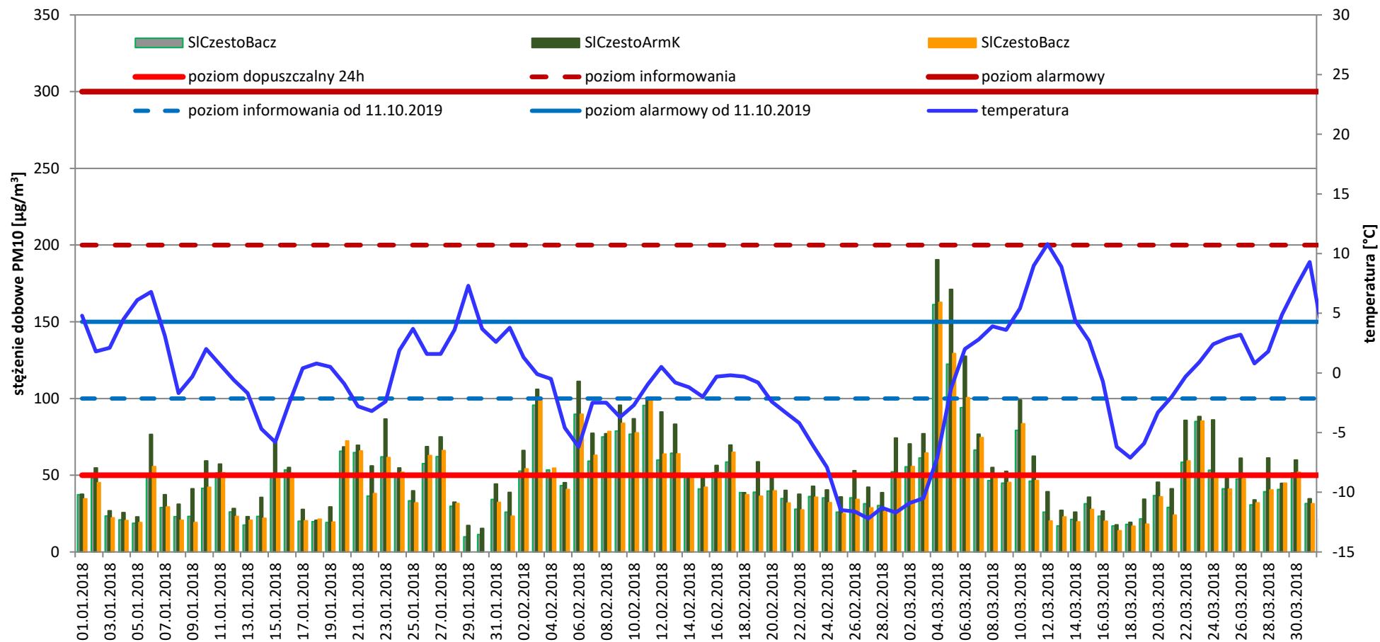
porównanie przebiegu zmienności stężeń 24-godz. PM10 w 2018 r. w Częstochowa w porównaniu z temperaturą
