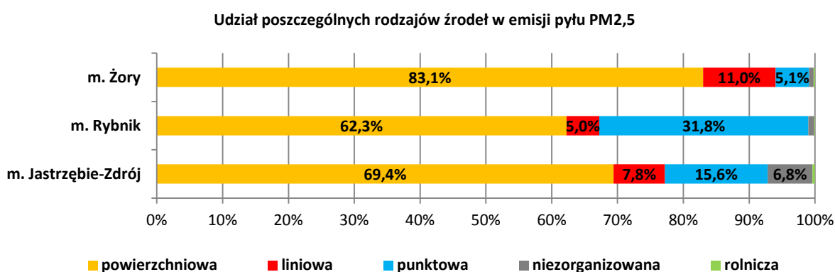
Rysunek 107. Procentowy udział poszczególnych rodzajów źródeł w sumarycznej emisji pyłu PM2,5 w miastach strefy aglomeracja rybnicko-jastrzębska w roku bazowym 2015 211
