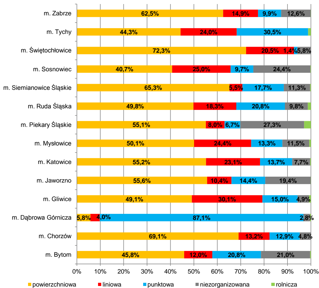
udział poszczególnych rodzajów źródeł w emisji pyłu zawieszzonego PM10
