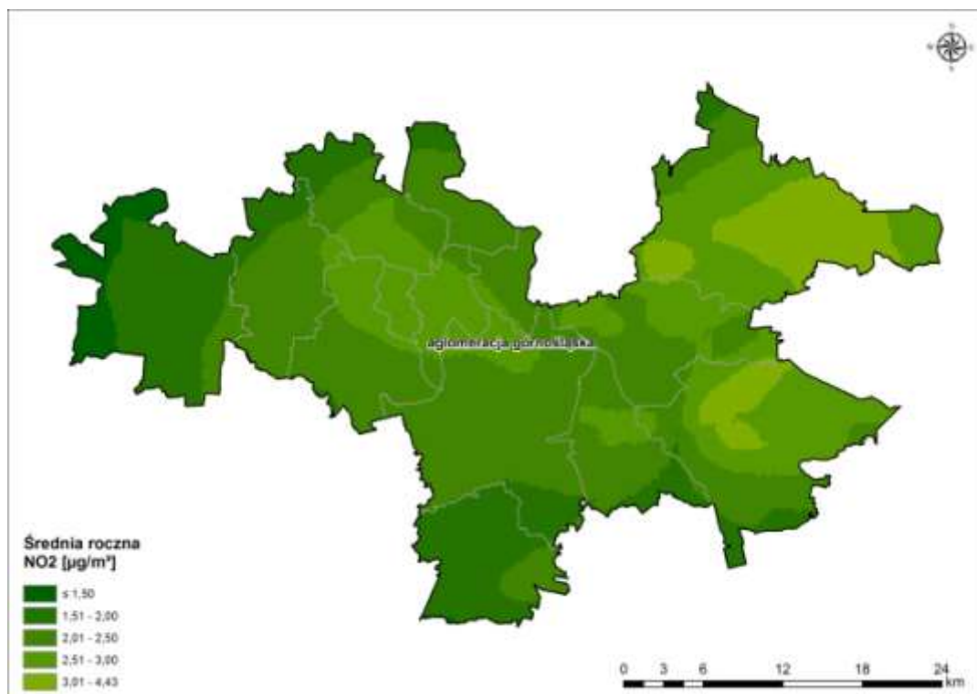
Rysunek 69. Rozkład stężeń średniorocznych \text{NO}_2 generowanych przez źródła punktowe w aglomeracji górnośląskiej 159
