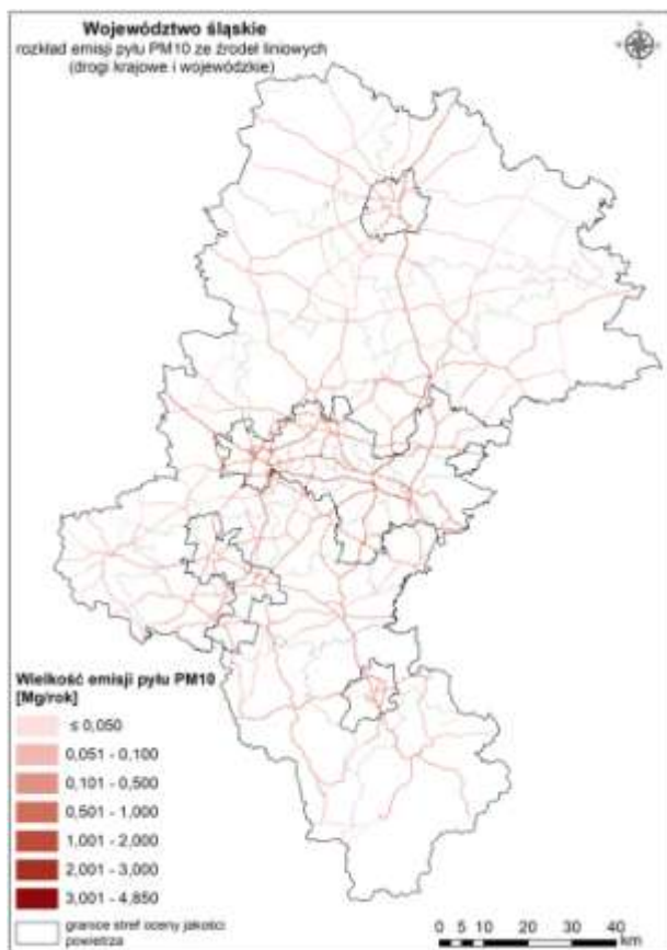
Rysunek 91. Rozkład przestrzenny emisji pyłu PM10, PM2,5 oraz tlenków azotu z dróg krajowych i wojewódzkich w województwie śląskim w roku bazowym 2015
