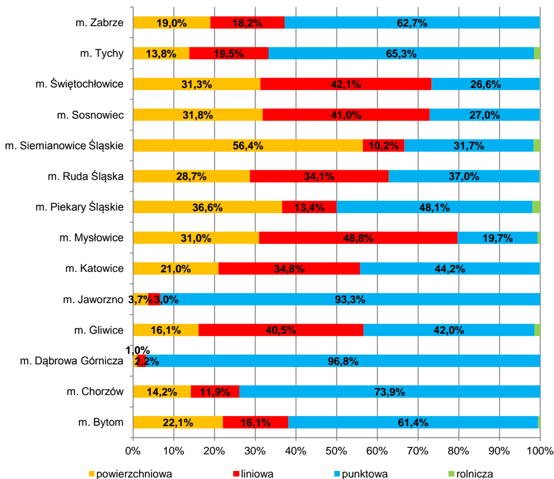
udział poszczególnych rodzajów źródeł w emisji tlenków azotu
