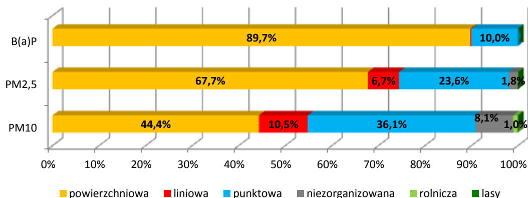
Rysunek 105. Procentowy udział poszczególnych rodzajów źródeł w sumarycznej emisji pyłu PM10, PM2,5 i B(a)P dla strefy aglomeracja rybnicko-jastrzębska w roku bazowym 2015 208
