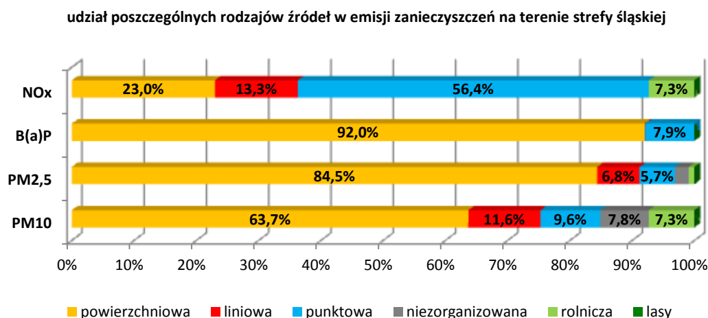
Rysunek 114. Procentowy udział poszczególnych rodzajów źródeł w sumarycznej emisji pyłu PM10, PM2,5, B(a)P i NOx dla strefy śląskiej w roku bazowym 2015 221
