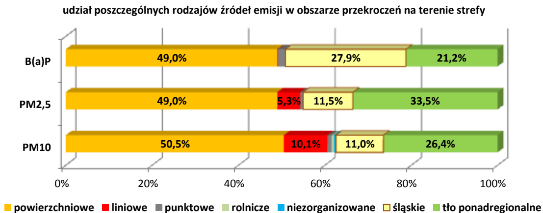
Rysunek 60. Udziały poszczególnych rodzajów źródeł emisji w wielkości stężeń analizowanych zanieczyszczeń w obszarze przekroczeń na terenie strefy miasto Częstochowa w roku bazowym 2015
