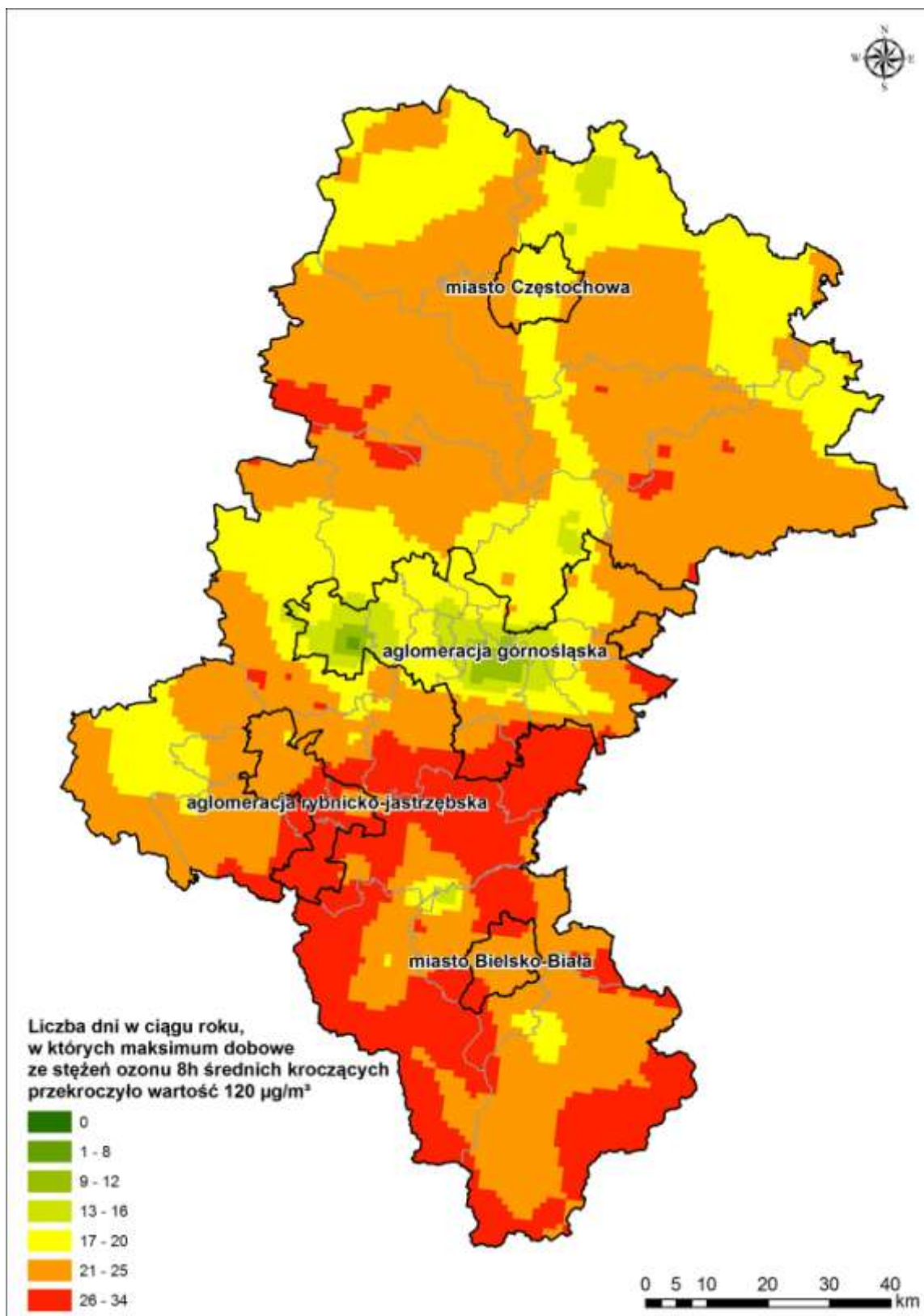
Rysunek 175. Rozkład liczby dni, w których maksymalne stężenie z ośmiogodzinnych średnich kroczących dla ozonu przekracza wartość 120 [µg/m 3 ] w województwie śląskim w roku bazowym 2015
