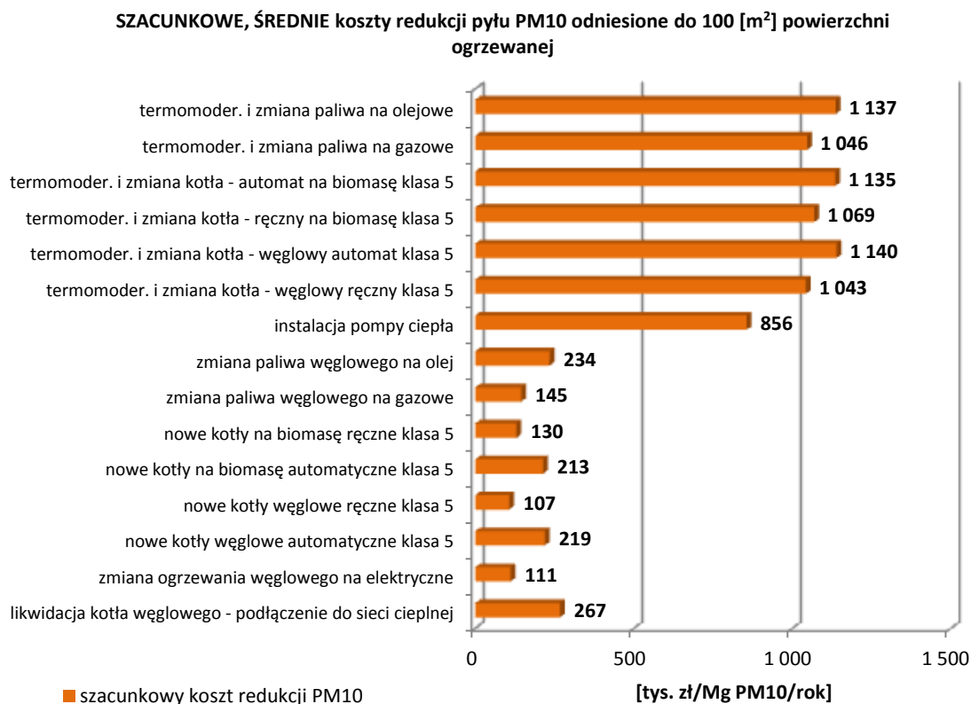
Rysunek 72. Porównanie szacunkowych, średnich wskaźników kosztów redukcji pyłu zawieszony PM10 z indywidualnych systemów grzewczych
