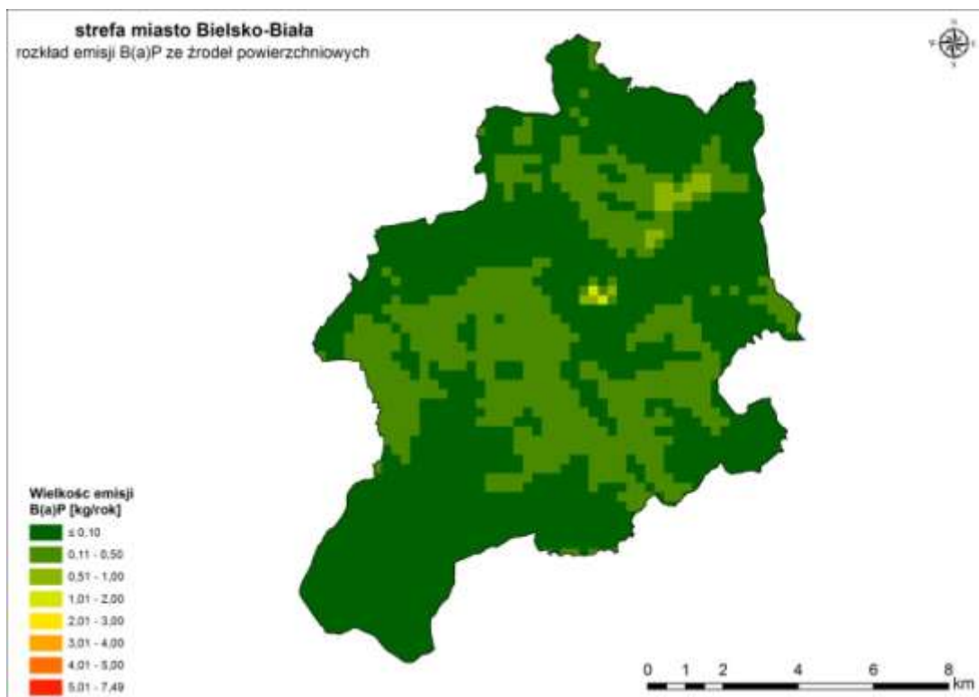
Rysunek 142. Lokalizacja i wielkość emisji B(a)P ze źródeł powierzchniowych w strefie miasto Bielsko-Biala w roku bazowym 2015 275
