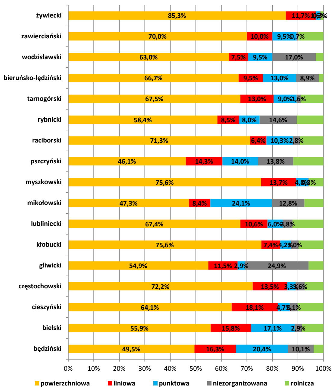
udział poszczególnych rodzajów źródeł w emisji pyłu PM10
