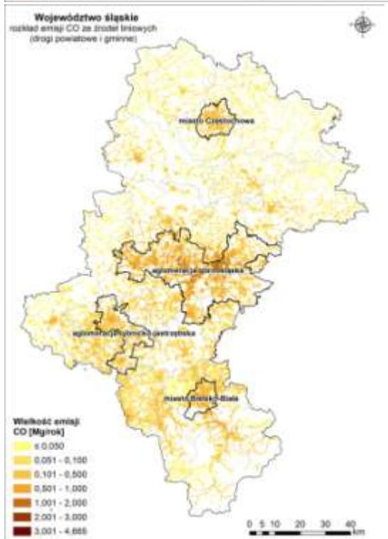
Rysunek 93. Rozkład przestrzenny emisji prekursorów pyłu i ozonu ze źródeł liniowych w siatce obliczeniowej w województwie śląskim w roku bazowym 2015
