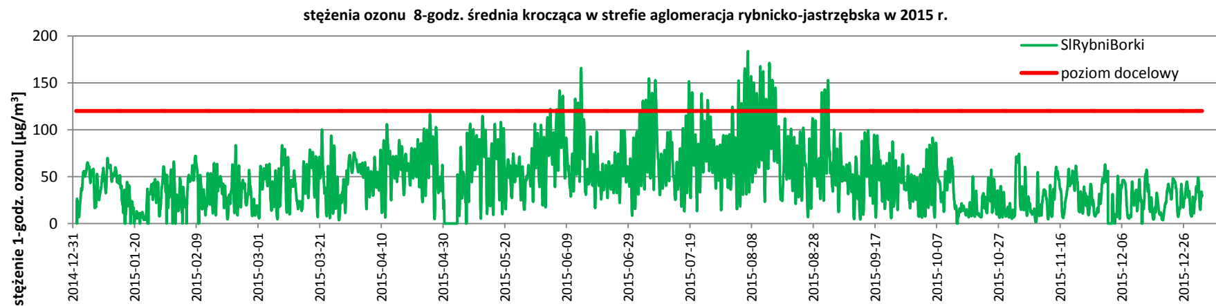
Rysunek 25. Przebieg zmienności ośmiogodzinnej średniej kroczącej dla ozonu w strefie aglomeracja rybnicko-jastrzębska w 2015 roku 96
