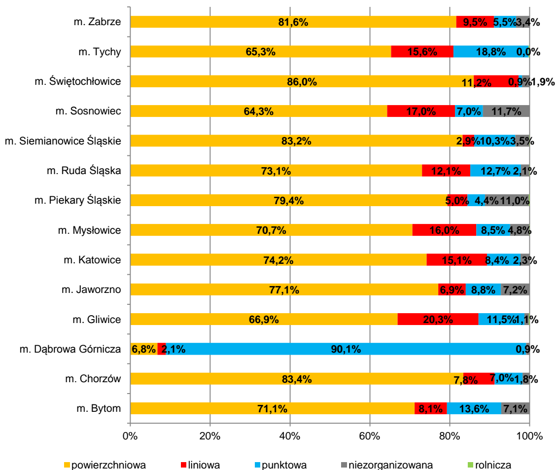
udział poszczególnych rodzajów źródeł w emisji pyłu zawieszonego PM2,5
