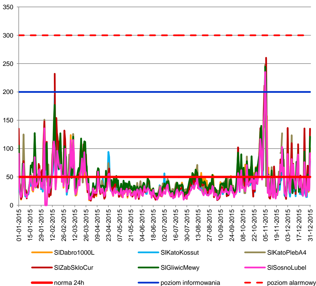
przebieg zmienności stężeń 24-godz. PM10 w 2015 r. - aglomeracja górnośląska
