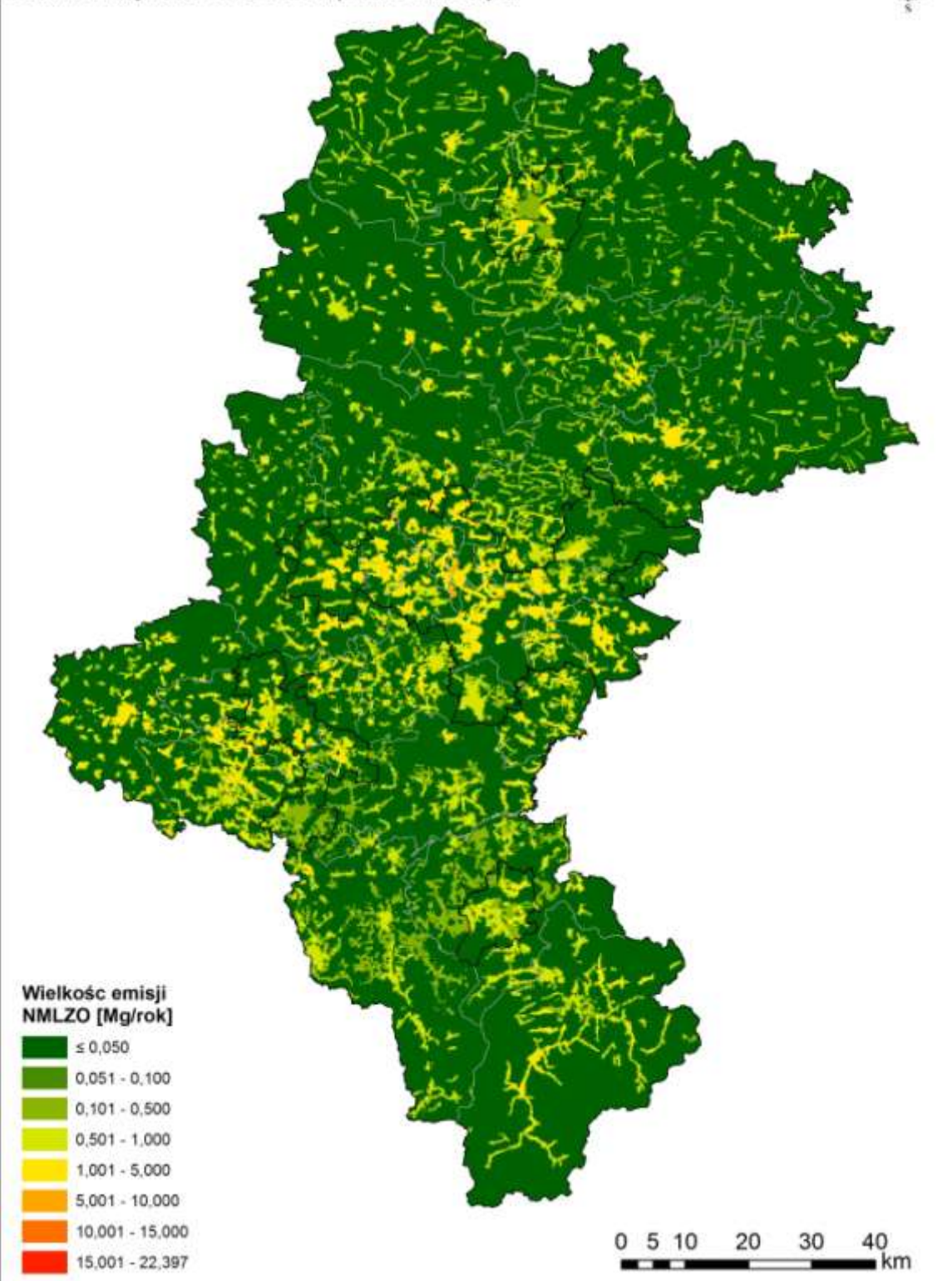
Rysunek 89. Lokalizacja i wielkość emisji NMLZO ze źródeł powierzchniowych w siatce obliczeniowej w województwie śląskim w roku bazowym 2015 roku 199
