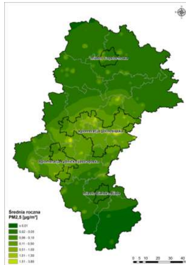
Rysunek 65. Rozkład stężeń średniorocznych pyłu PM10 i PM2,5 generowanych przez źródła nieorganizowane w województwie śląskim 155
