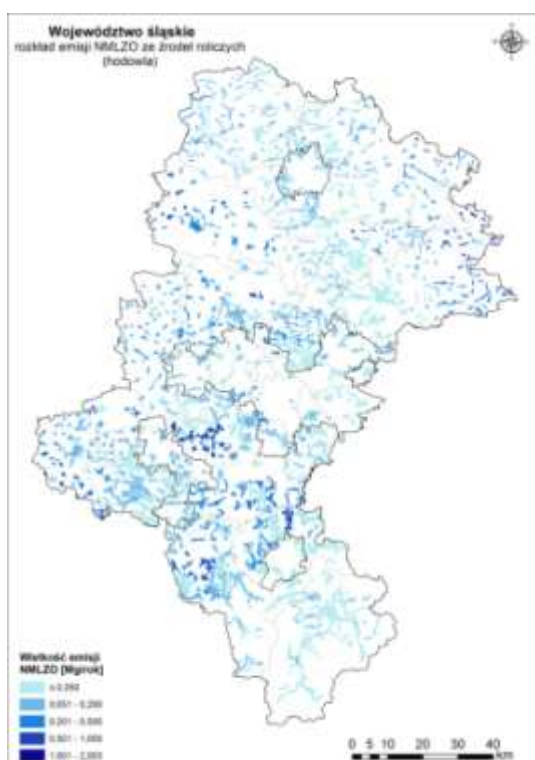
Rysunek 96. Rozkład przestrzenny emisji prekursorów pyłu i ozonu z hodowli w siatce obliczeniowej na terenie województwa śląskiego w roku bazowym 2015
