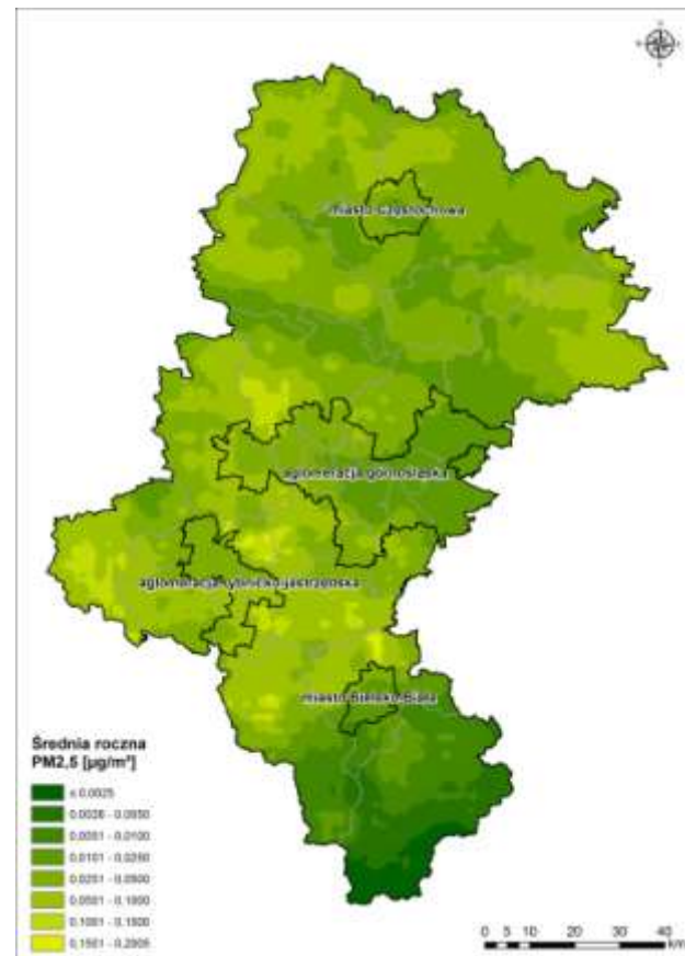
Rysunek 66. Rozkład stężeń średniorocznych pyłu PM10, PM2,5 oraz B(a)P generowanych przez źródła rolnicze w województwie śląskim 156
