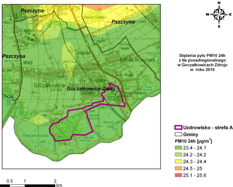
Rysunek 47. Stężenia PM10 o okresie uśredniania wyników 24h w Goczałkowicach - Zdroju pochodzące z tła ponadregionalnego w 2010 r.
