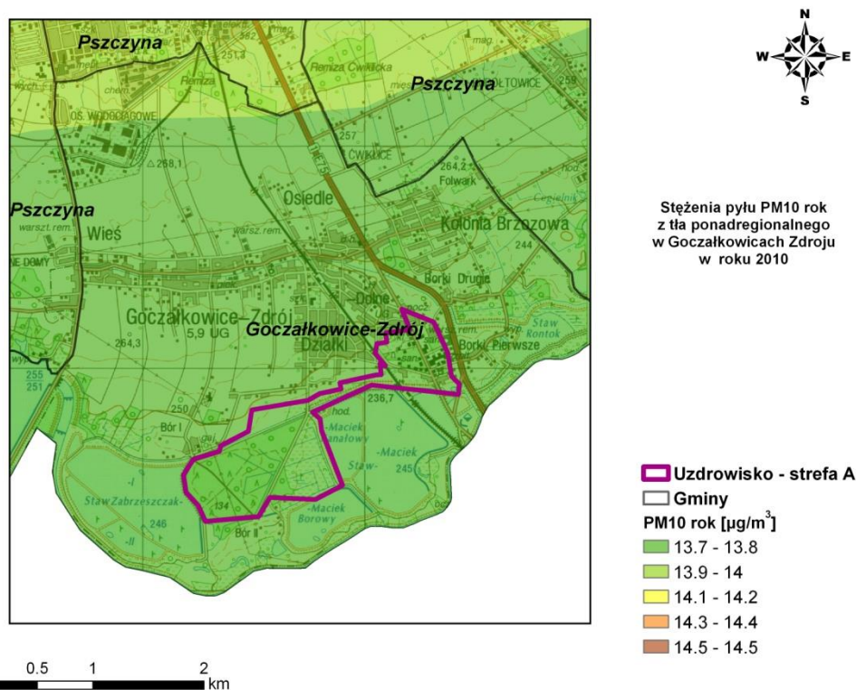
Rysunek 49. Stężenia PM10 o okresie uśredniania wyników rok w Goczałkowicach - Zdroju pochodzące z tła ponadregionalnego w 2010 r.
