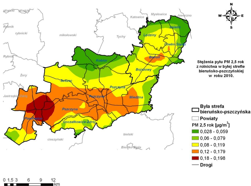
Rysunek 90. Stężenia pyłu zawieszono PM 2,5 o okresie uśredniania wyników rok w byłej strefie bieruńsko-pszczyńskiej pochodzące z emisji z rolnictwa w 2010 r.
