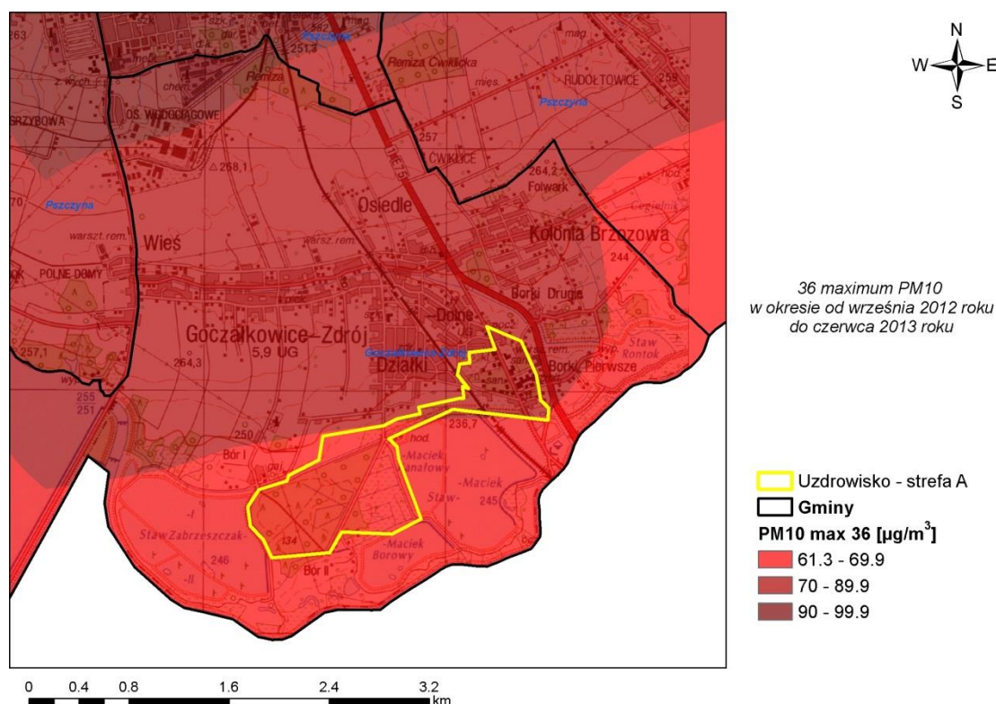
Rysunek 144. Stężenia pyłu zawieszonego PM10 o okresie uśredniania wyników 24h w byłej strefie bieruńsko-pszczyńskiej pochodzące z łącznej emisji wszystkich typów w okresie od września 2012 r. do czerwca 2013 r.
