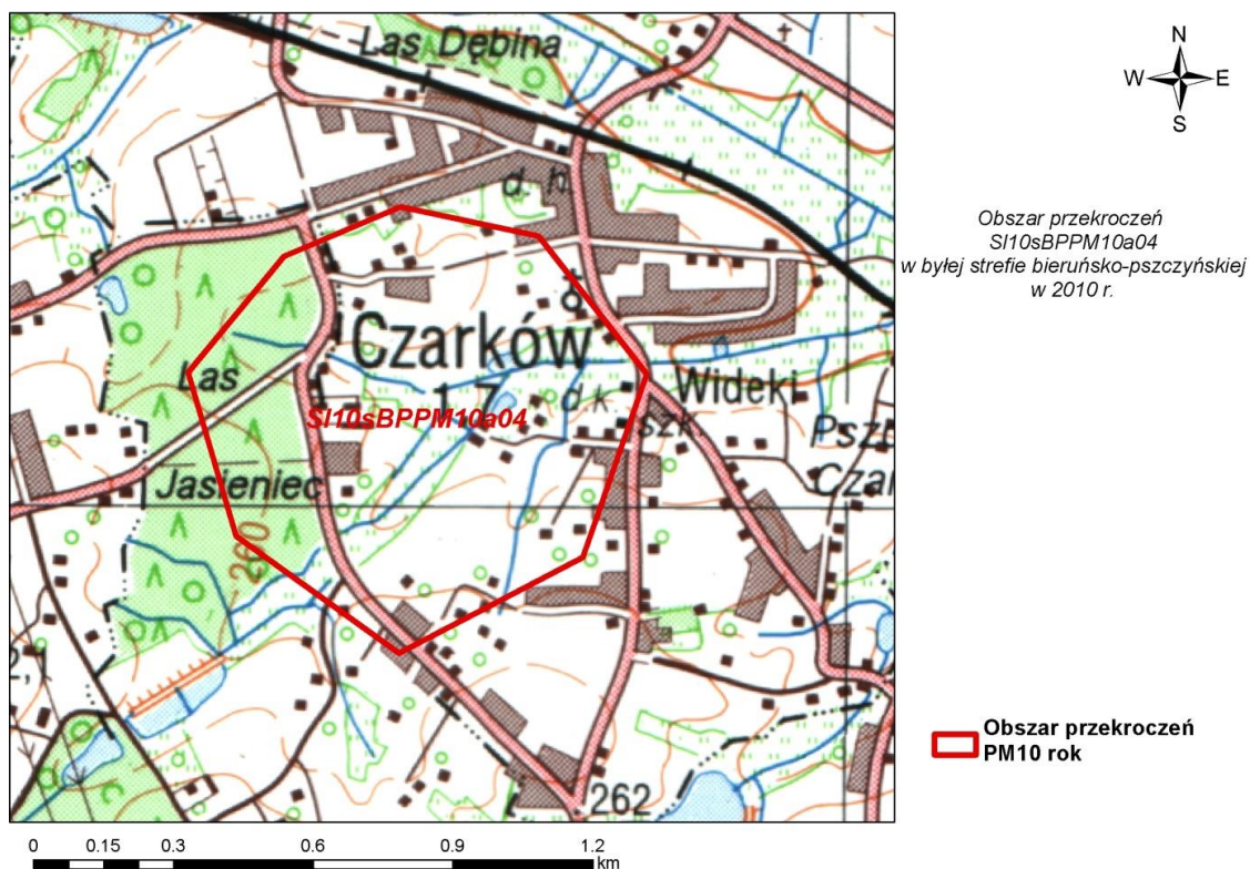
Rysunek 102. Obszar przekroczeń poziomu dopuszczalnego PM10 rok SI10sBPPM10a04 w byłej strefie bieruńsko-pszczyńskiej w 2010 r.
