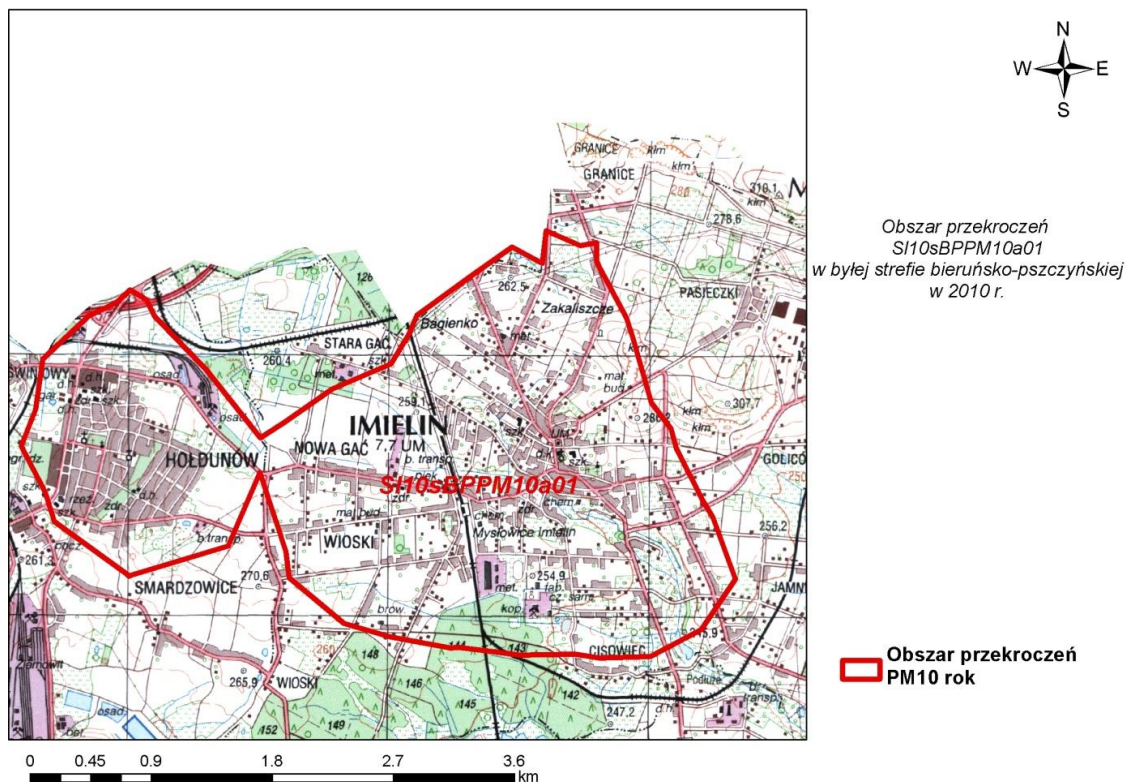
Rysunek 96. Obszar przekroczeń poziomu dopuszczalnego PM10 rok SI10sBPPM10a01 w byłej strefie bieruńsko-pszczyńskiej w 2010 r.
