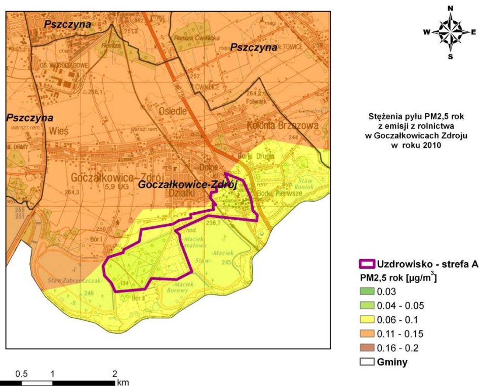
Rysunek 91. Stężenia pyłu zawieszono PM 2,5 o okresie uśredniania wyników rok w strefie bieruńsko-pszczyńskiej pochodzące z emisji z rolnictwa w 2010 r.
