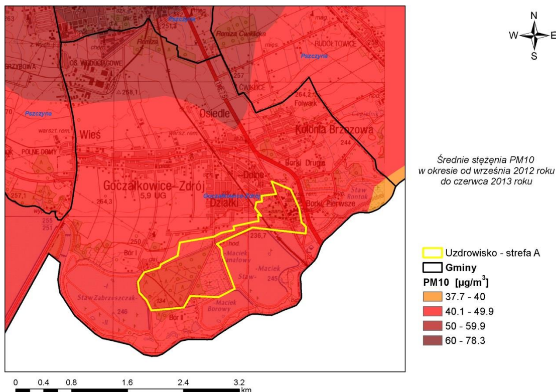
Rysunek 145. Stężenia pyłu zawieszonego PM10 w byłej strefie bieruńsko-pszczyńskiej pochodzące z łącznej emisji wszystkich typów w okresie od września 2012 r. do czerwca 2013 r.
