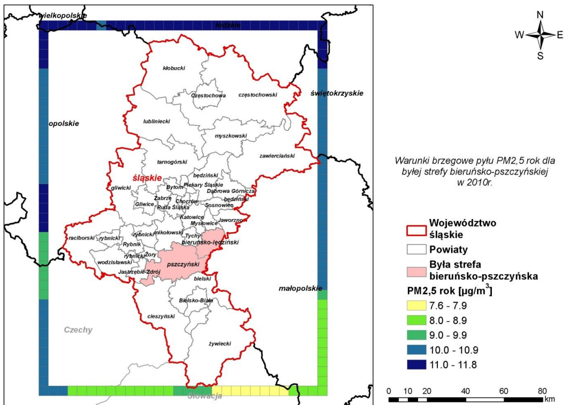
Rysunek 11. Warunki brzegowe pyłu zawieszono PM2,5 dla byłej strefy bieruńsko-pszczyńskiej w 2010 r.
