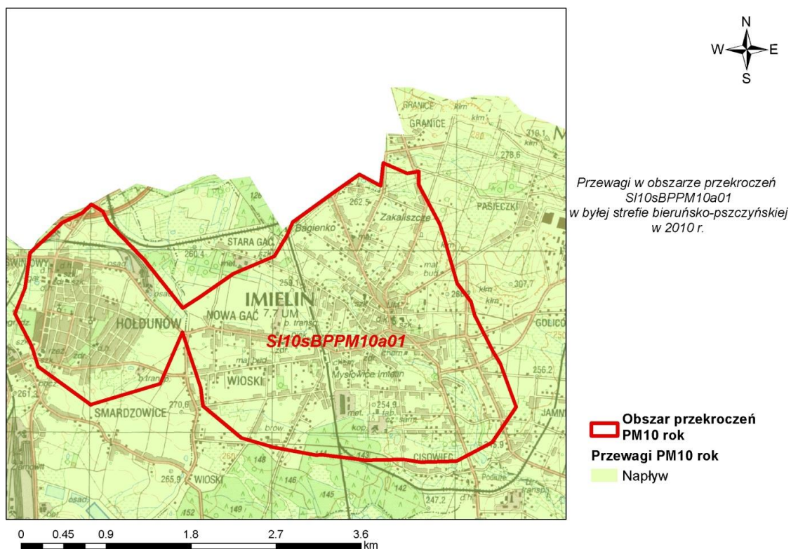
Rysunek 97. Przewagi typów emisji w stężeniach PM10 rok w obszarze przekroczeń SI10sBPPM10a01 w byłej strefie bieruńsko-pszczyńskiej w 2010 r.
