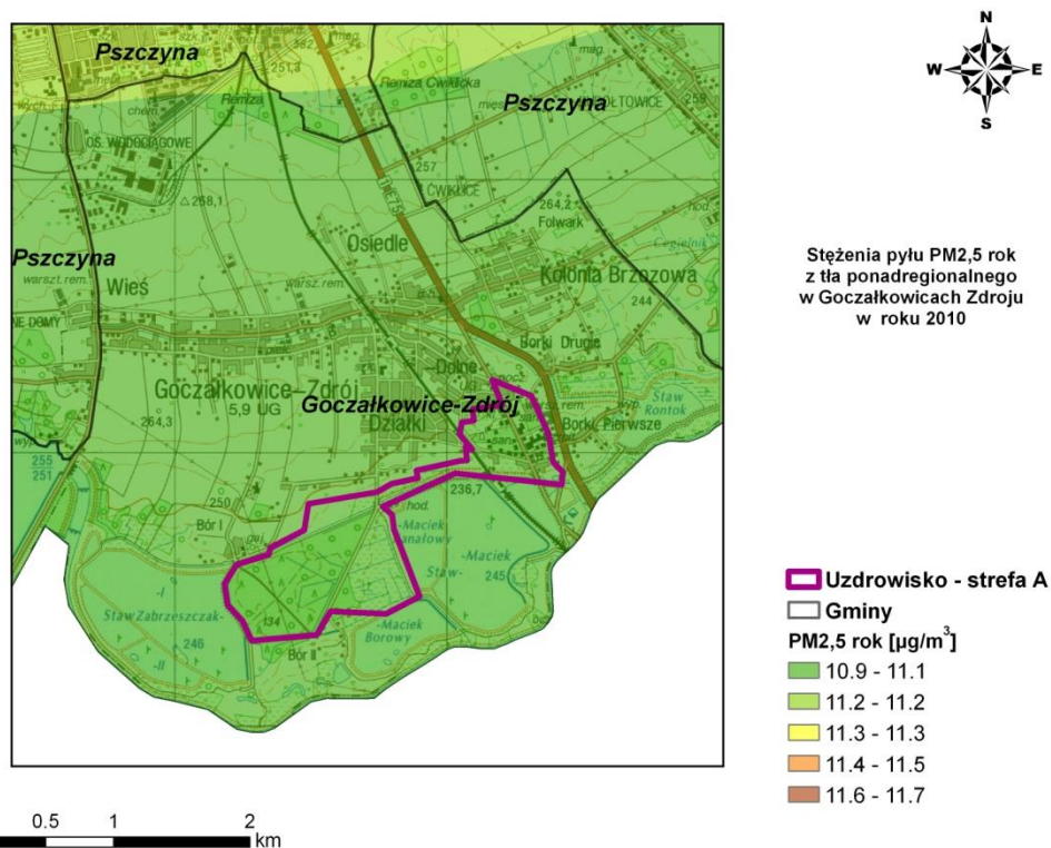
Rysunek 79. Stężenia PM 2,5 o okresie uśredniania wyników rok w Goczałkowicach - Zdroju z tła ponadregionalnego w 2010 r.
