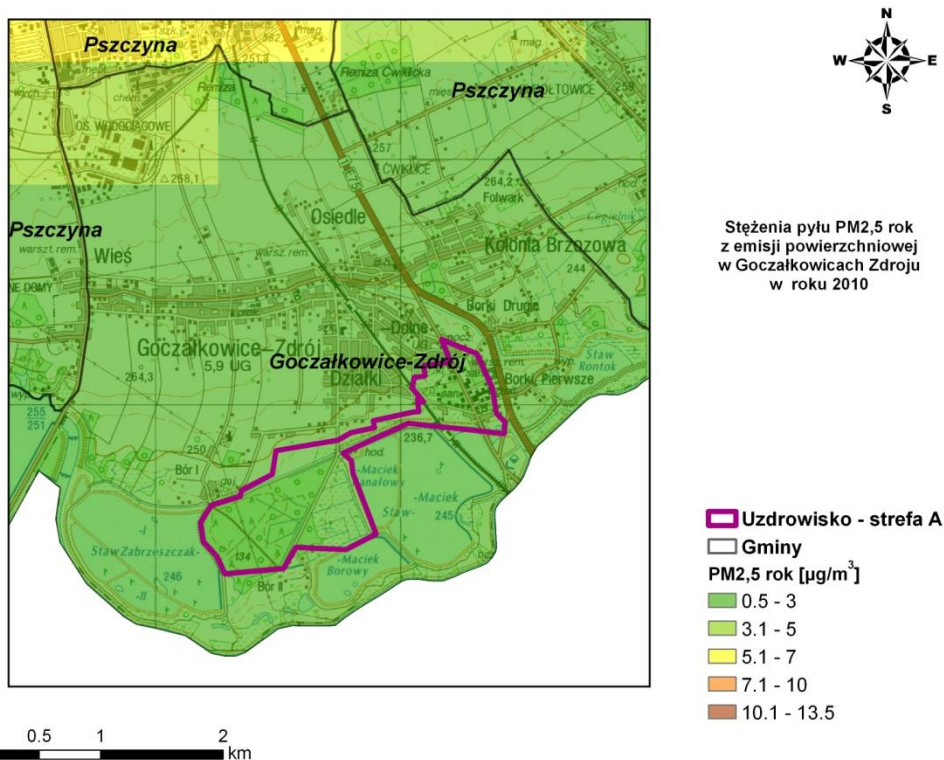
Rysunek 87. Stężenia pyłu zawieszonego PM 2,5 o okresie uśredniania wyników rok w Goczałkowicach – Zdroju pochodzące z emisji komunalnej w 2010 r.
