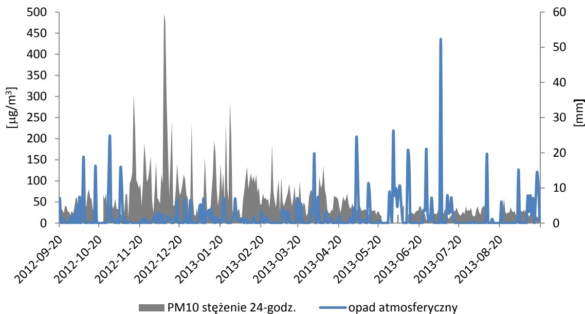
Rysunek 134. Średnie dobowe stężenie PM10 na tle sumy dobowego opadu atmosferycznego na stacji Katowice-Muchowiec od 20 września 2012 r. do 19 września 2013 r. dla Goczałkowic-Zdroju.
