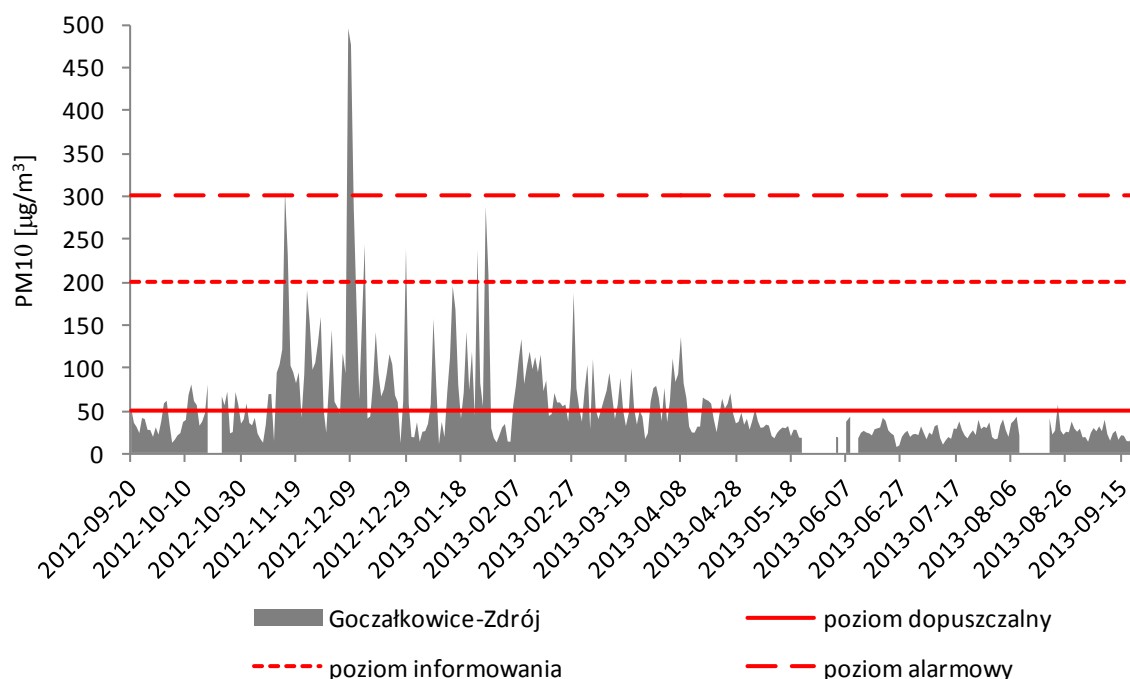
Rysunek 129. Stężenie średnie dobowe PM10 w okresie od 20.09.2012 r. do 19.09.2013 r. na tle poziomu dopuszczalnego, poziomu informowania i alarmowego dla Goczałkowice-Zdroju.
