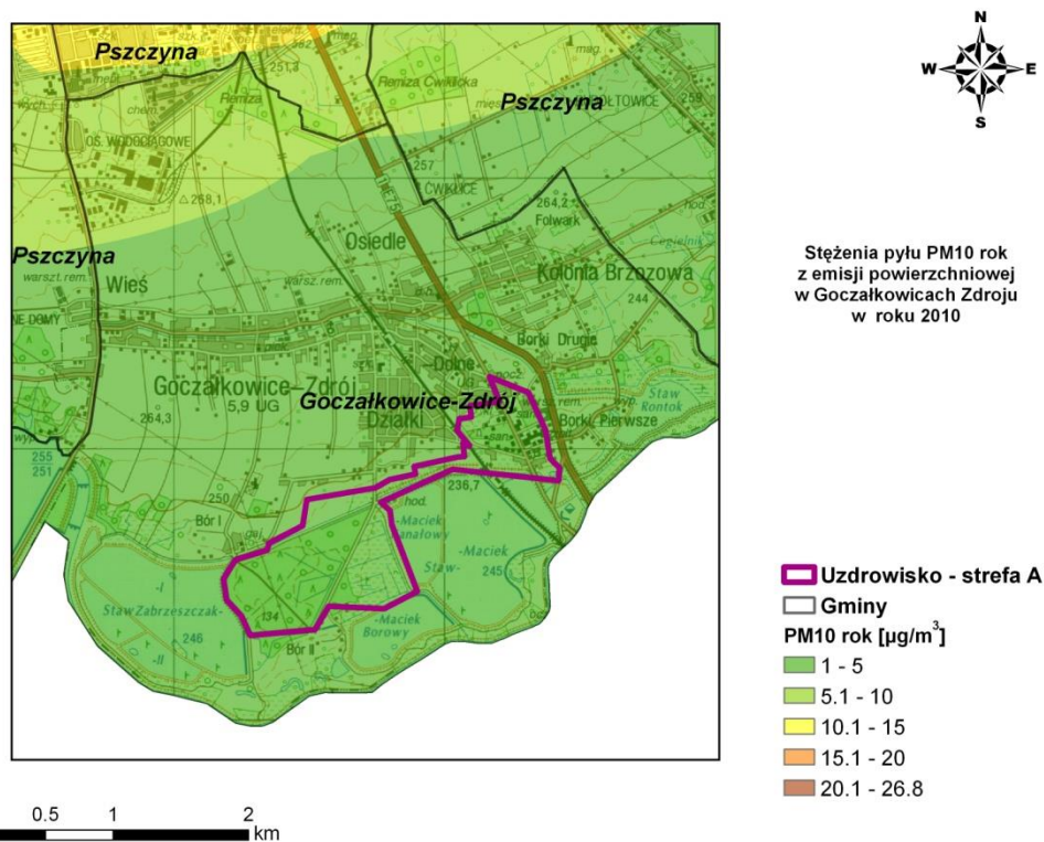
Rysunek 65. Stężenia pyłu zawieszonego PM10 o okresie uśredniania wyników rok w Goczałkowicach – Zdroju pochodzące z emisji komunalnej w 2010 r.
