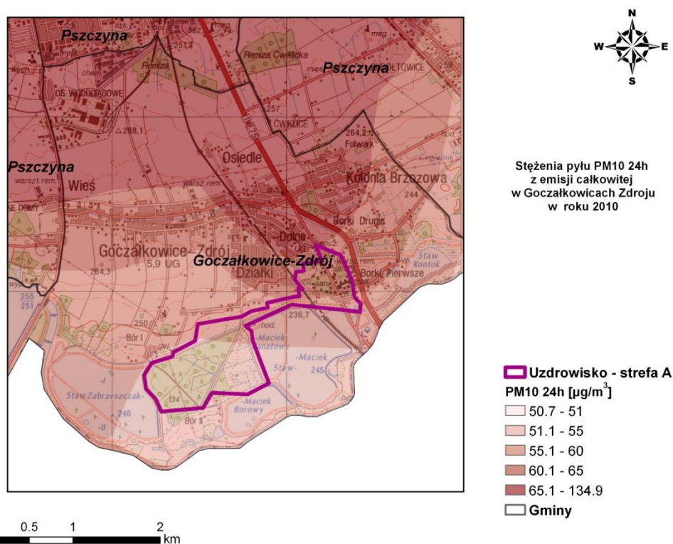
Rysunek 75. Stężenia pyłu zawieszonego PM10 o okresie uśredniania wyników 24h w Goczałkowicach - Zdroju pochodzące z łącznej emisji wszystkich typów w 2010 r.
