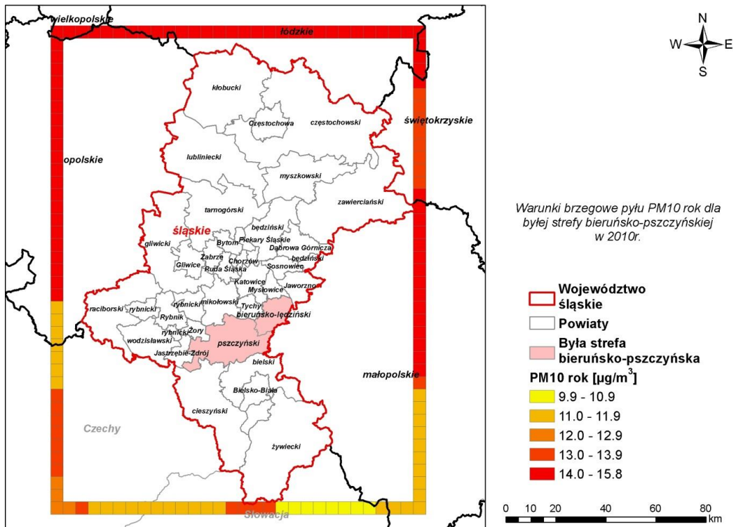
Rysunek 10. Warunki brzegowe pyłu zawieszono PM10 dla byłej strefy bieruńsko-pszczyńskiej w 2010r.
