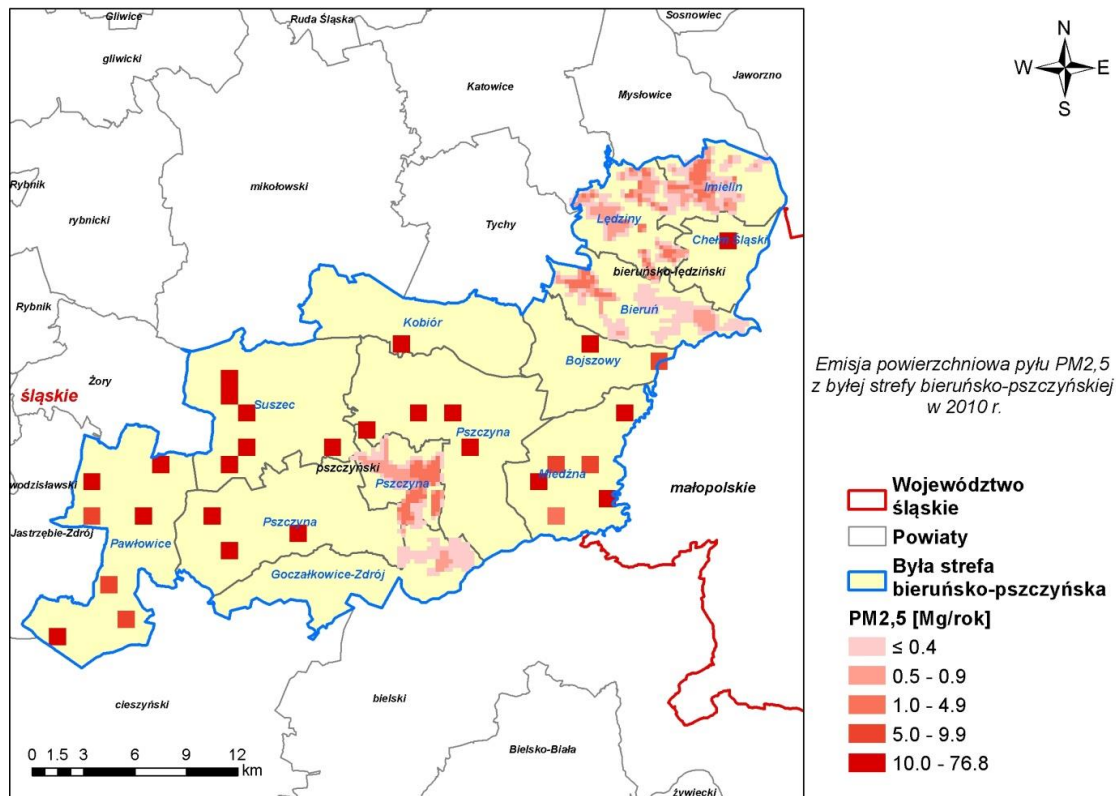
Rysunek 22. Emisja powierzchniowa pyłu zawieszonego PM 2,5 w byłej strefie bieruńsko-pszczyńskiej w 2010 r.
