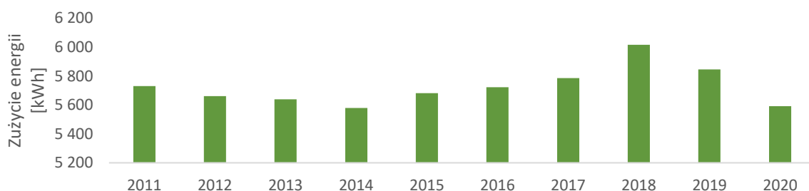
Wykres 31. Zużycie energii elektrycznej w przeliczeniu na 1 mieszkańca w województwie śląskim w latach 2011-2020.
