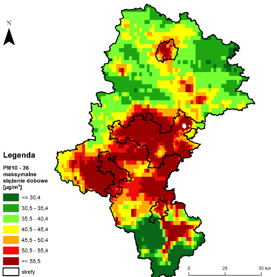
Rysunek 4-13 Rozkład przestrzenny 36. Maksymalnej wartości stężenia 24-godzinnego pyłu zawieszonego PM10 w województwie śląskim w 2021 roku, opracowany z wykorzystaniem metody szacowania w oparciu o wyniki modelowania jakości powietrza dla roku 2021, wykonanego przez IOŚ-PIB. Źródło: GIOŚ, 2022
