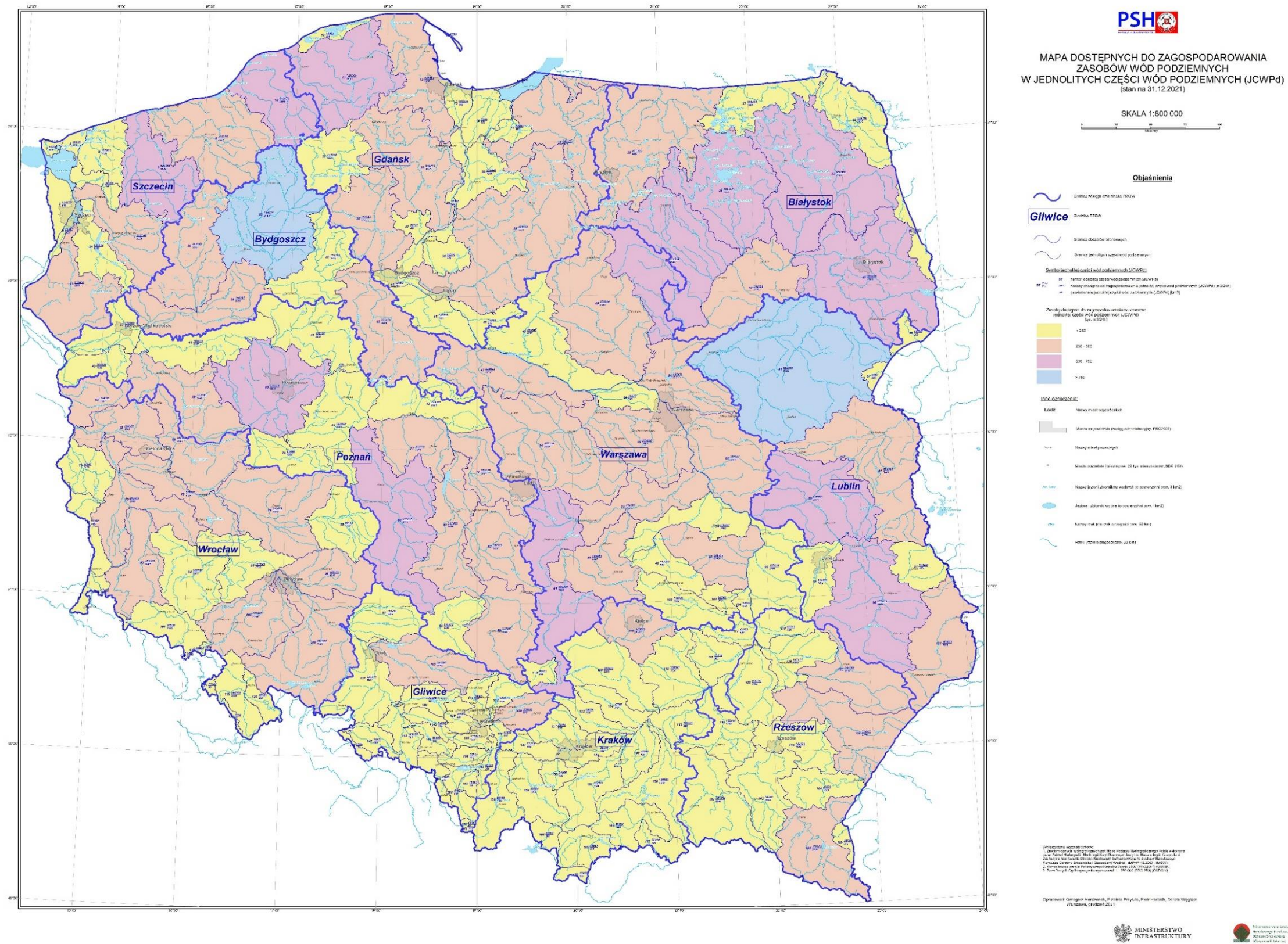
Rysunek 4-24 Mapa zasobów dyspozycyjnych według jednolitych części wód podziemnych, źródło [47].
