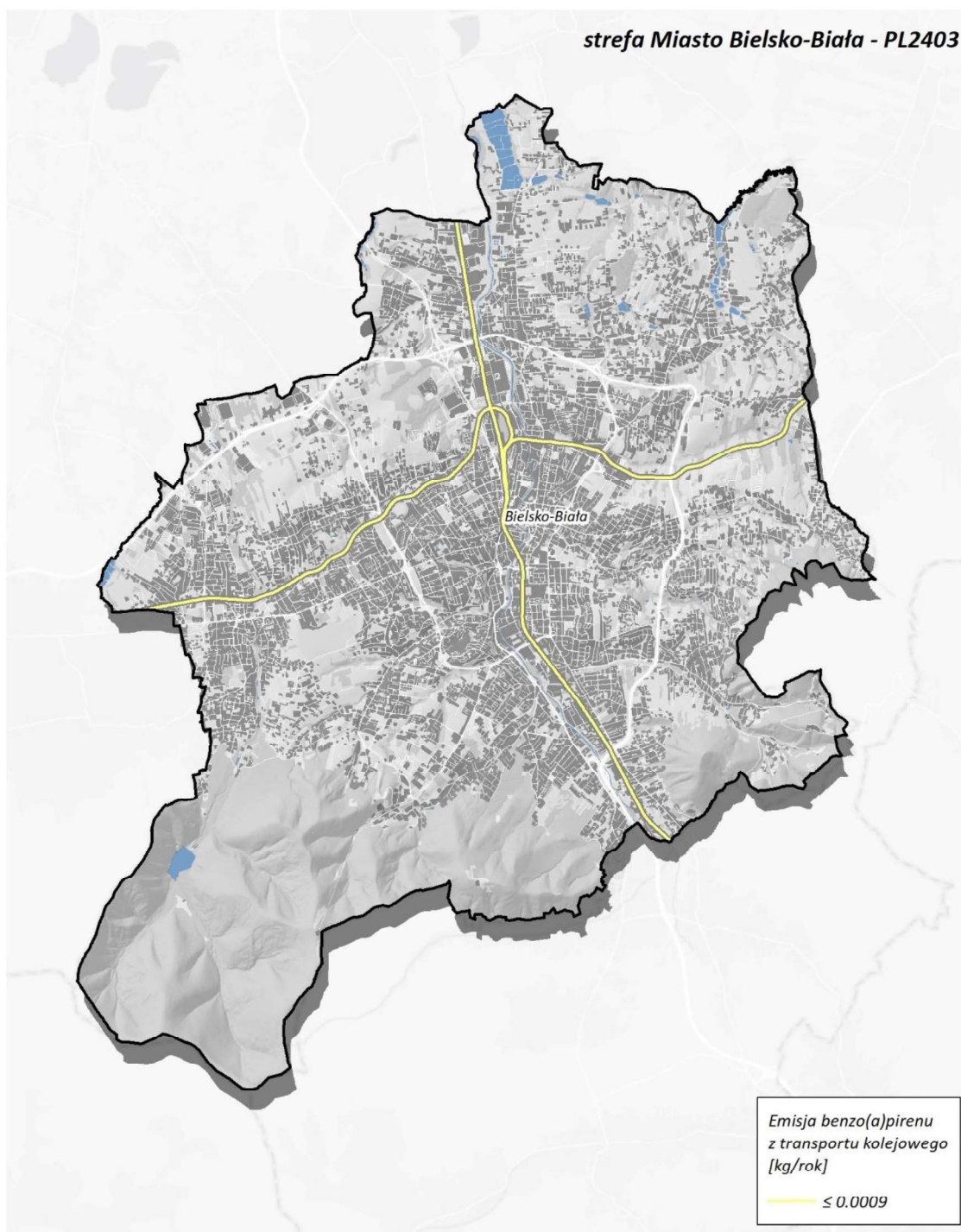
Rysunek 150. Lokalizacja i wielkość emisji B(a)P z kolei w Bielsku-Białej w roku bazowym 2022 322
