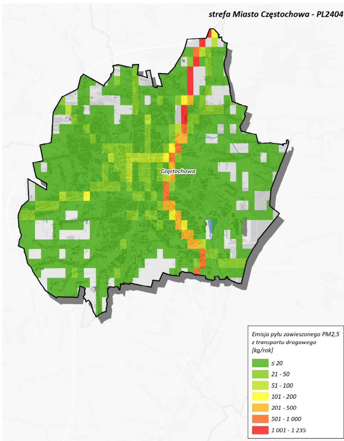
Rysunek 156. Lokalizacja i wielkość emisji pyłu PM 2,5 z sektora transportu drogowego w Częstochowie w roku bazowym 2022 328
