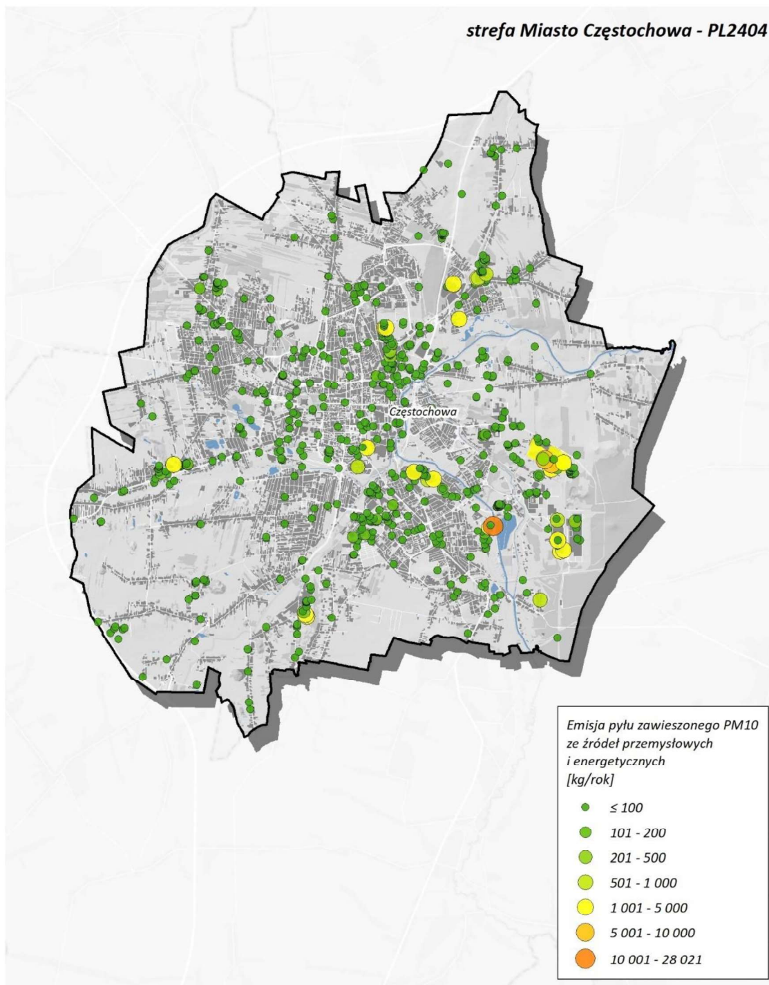
Rysunek 158. Lokalizacja i wielkość emisji pyłu PM10 z przemysłu i energetyki w Częstochowie w roku bazowym 2022 330
