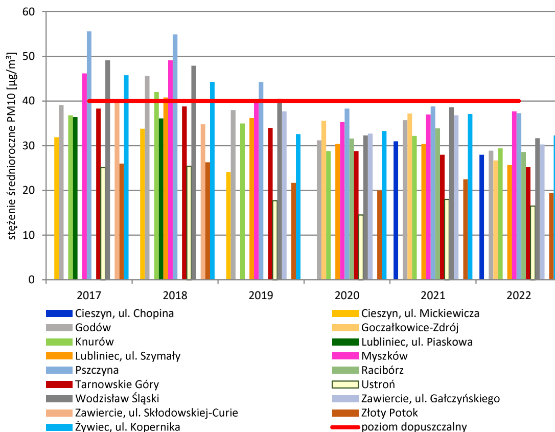
Rysunek 39. Wyniki pomiarów stężeń średniorocznych pyłu PM10 w latach 2017-2022 w strefie śląskiej 131
