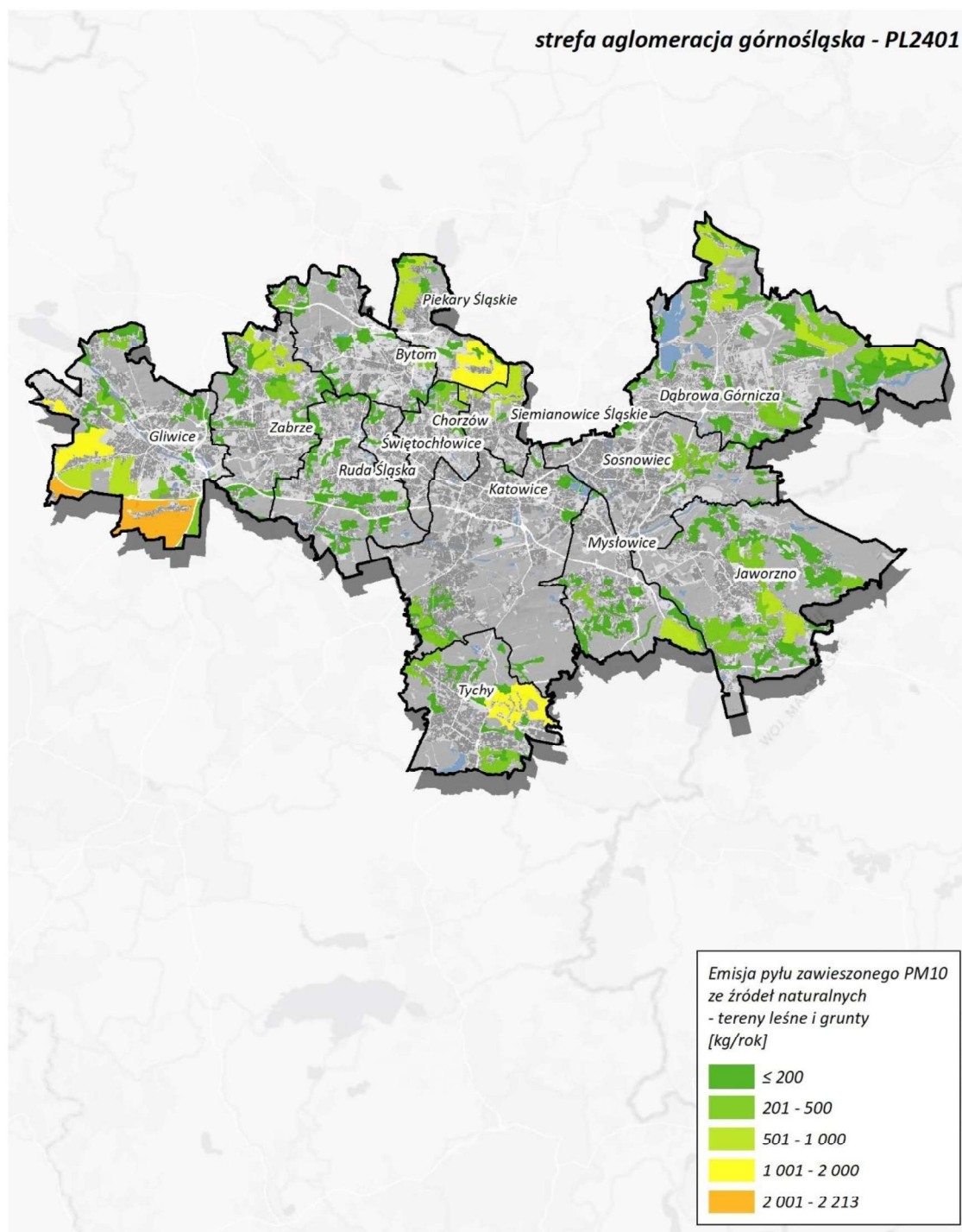
Rysunek 104. Lokalizacja i wielkość emisji pyłu PM10 ze źródeł naturalnych w aglomeracji górnośląskiej w roku bazowym 2022 276
