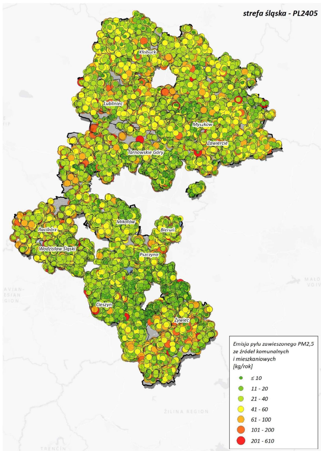
Rysunek 214. Lokalizacja i wielkość emisji pyłu PM 2,5 ze źródeł z sektora komunalno-bytowego w strefie śląskiej w roku bazowym 2022 386
