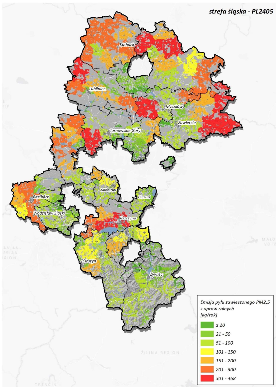
Rysunek 190. Lokalizacja i wielkość emisji pyłu PM 2,5 z upraw rolnych w strefie śląskiej w roku bazowym 2022 362
