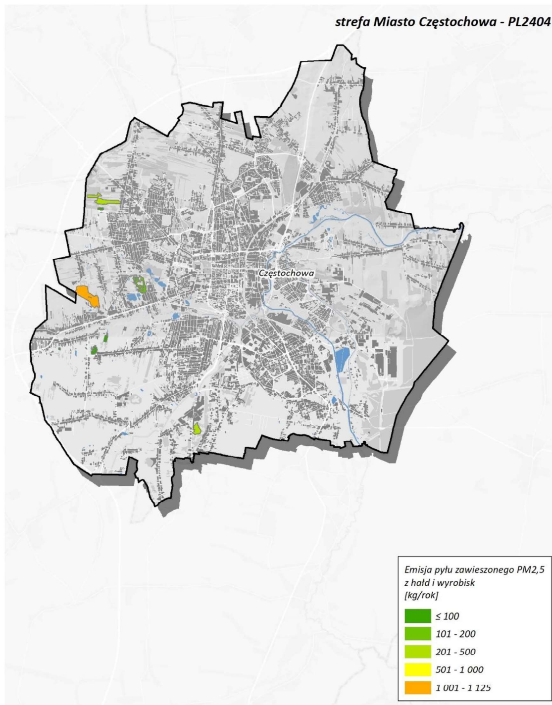
Rysunek 167. Lokalizacja i wielkość emisji pyłu PM 2,5 ze źródeł niezorganizowanych (hałdy i wyrobiska) w Częstochowie w roku bazowym 2022 339
