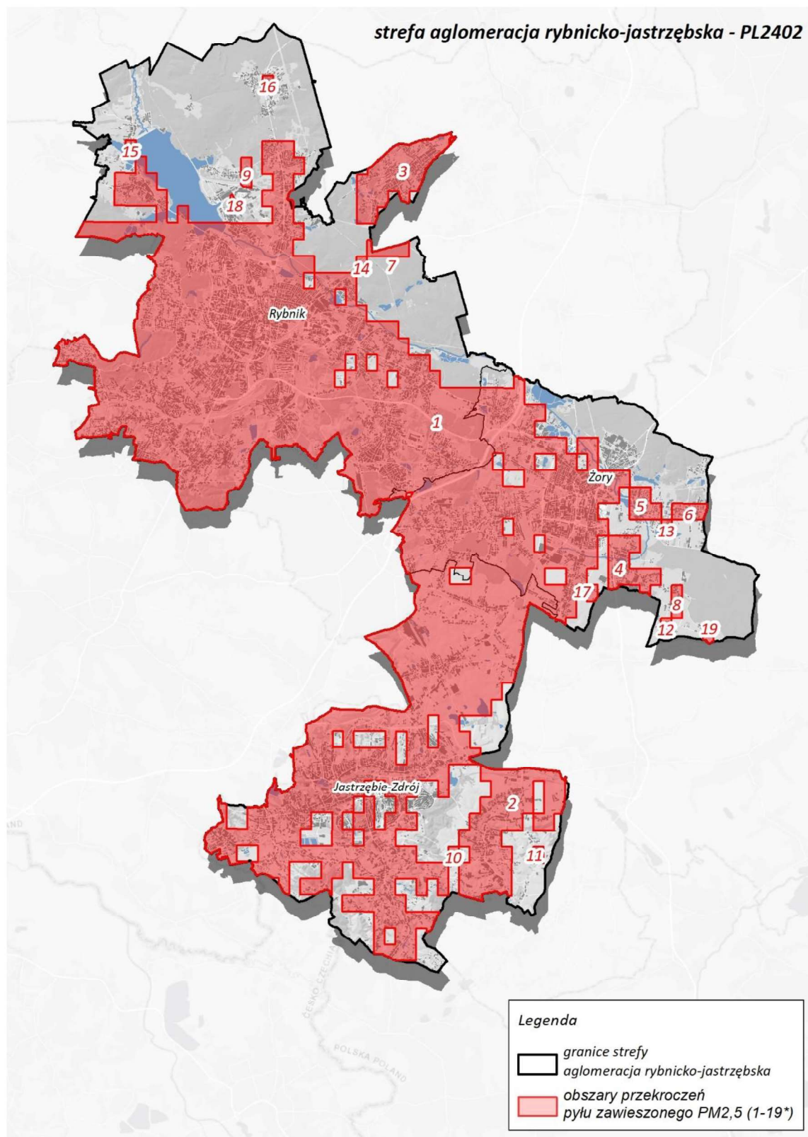
Rysunek 50. Obszary przekroczeń poziomu dopuszczalnego dla pyłu PM 2,5 na terenie aglomeracji rybnicko-jastrzębskiej w 2022 roku 149
