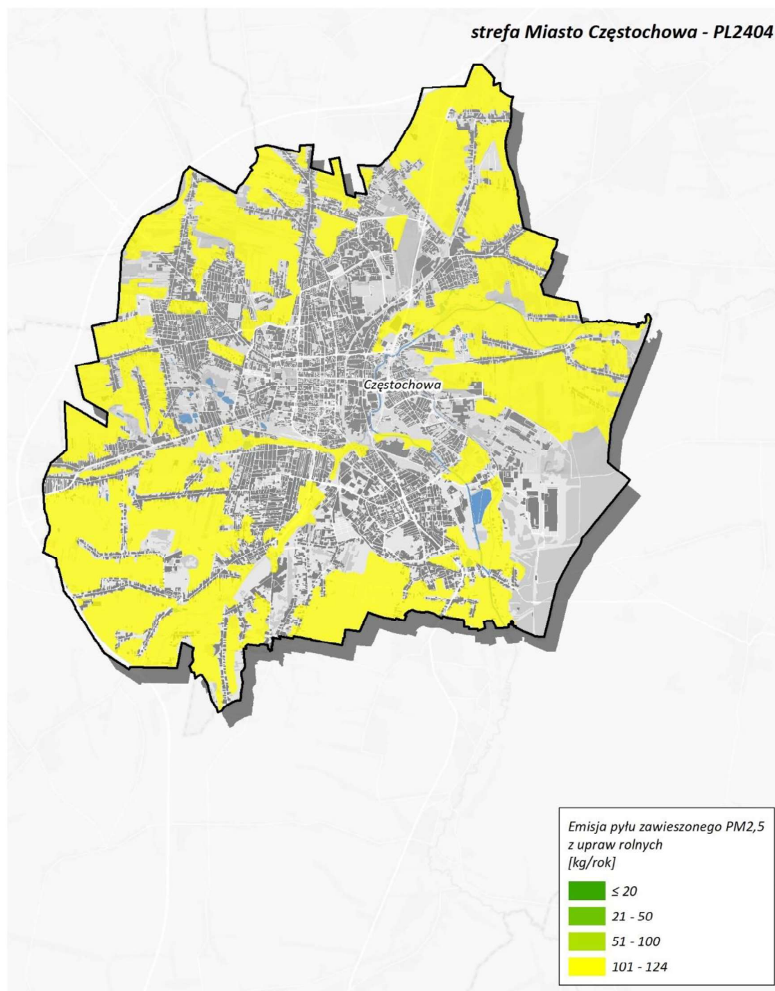
Rysunek 171. Lokalizacja i wielkość emisji pyłu PM 2,5 z upraw rolnych w Częstochowie w roku bazowym 2022 343
