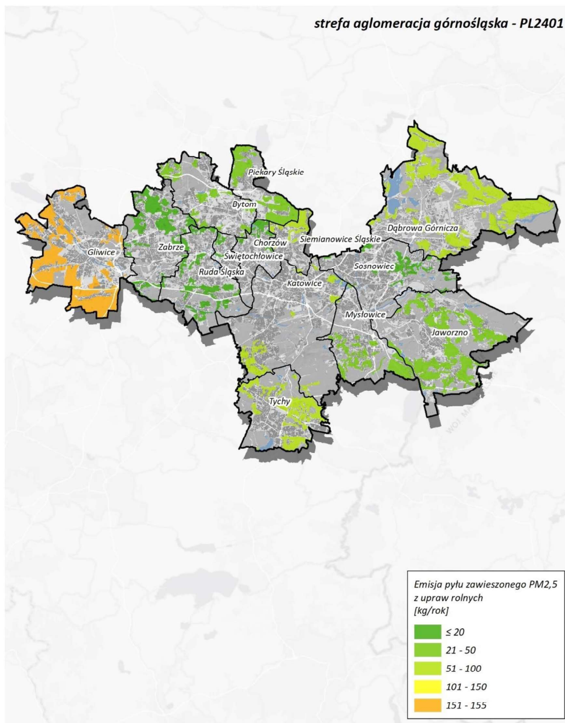
Rysunek 116. Lokalizacja i wielkość emisji pyłu PM 2,5 z upraw rolnych w aglomeracji górnośląskiej w roku bazowym 2022 288
