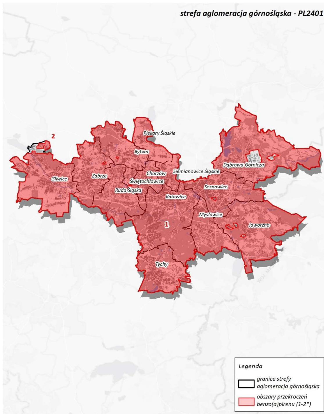
Rysunek 47. Obszary przekroczeń poziomu docelowego benzo(a)pirenu na terenie aglomeracji górnośląskiej w 2022 roku 142
