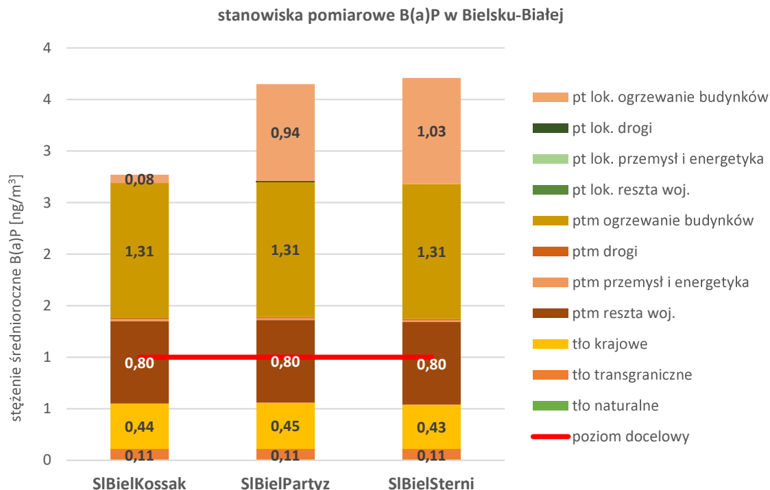
Rysunek 75. Prezentacja poziomów tła regionalnego, przyrostu tła miejskiego oraz lokalnego przyrostu stężeń na stanowiskach pomiarowych pomiarowych benzo(a)pirenu w Bielsku-Białej w 2022 roku 179
