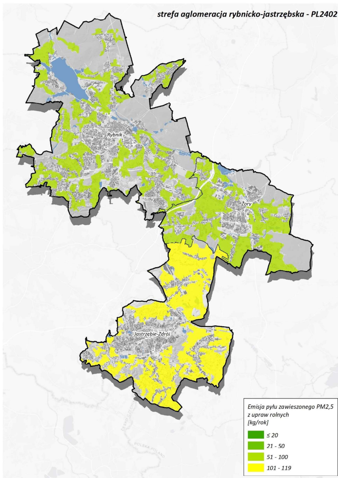
Rysunek 139. Lokalizacja i wielkość emisji pyłu PM 2,5 z upraw rolnych w aglomeracji rybnicko-jastrzębskiej w roku bazowym 2022 311
