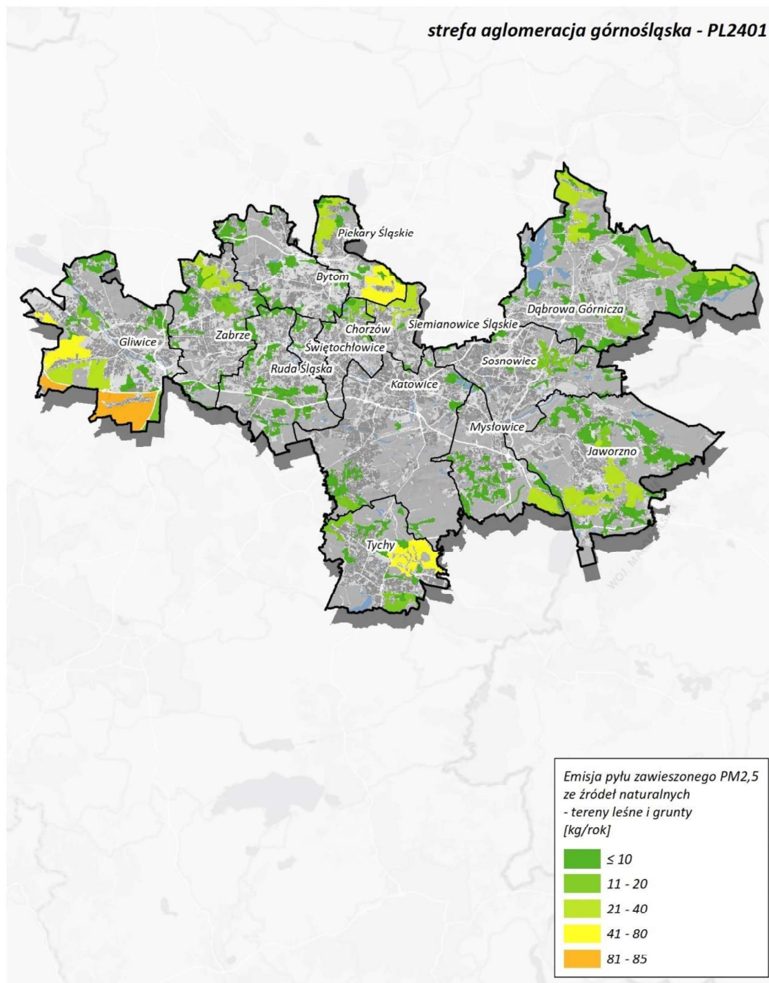
Rysunek 105. Lokalizacja i wielkość emisji pyłu PM 2,5 ze źródeł naturalnych w aglomeracji górnośląskiej w roku bazowym 2022 277
