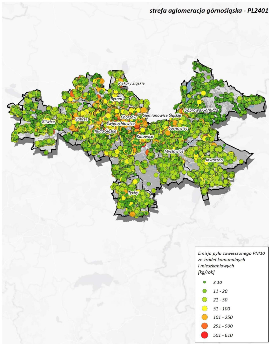
Rysunek 197. Lokalizacja i wielkość emisji pyłu PM10 ze źródeł z sektora komunalno-bytowego w aglomeracji górnośląskiej w roku bazowym 2022 369
