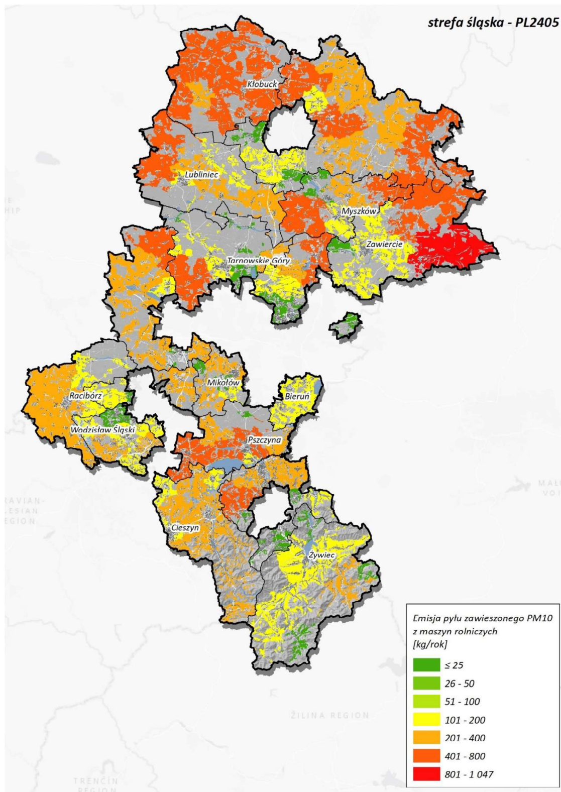
Rysunek 187. Lokalizacja i wielkość emisji pyłu PM10 z maszyn rolniczych w strefie śląskiej w roku bazowym 2022 359
