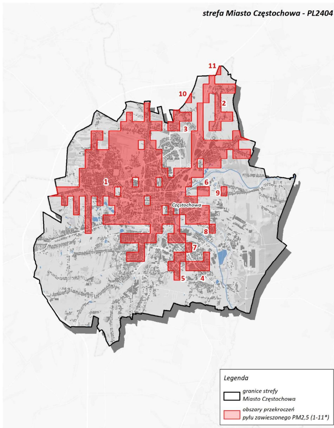
Rysunek 55. Obszary przekroczeń poziomu dopuszczalnego dla pyłu PM 2,5 na terenie strefy miasto Częstochowa w 2022 roku 159
