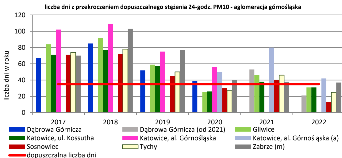
Rysunek 15. Liczba dni z przekroczeniem poziomu dopuszczalnego 24-godzinny pyłu zawieszony PM10 w latach 2017-2022 w punktach pomiarowych w strefie aglomeracja górnośląska 72
