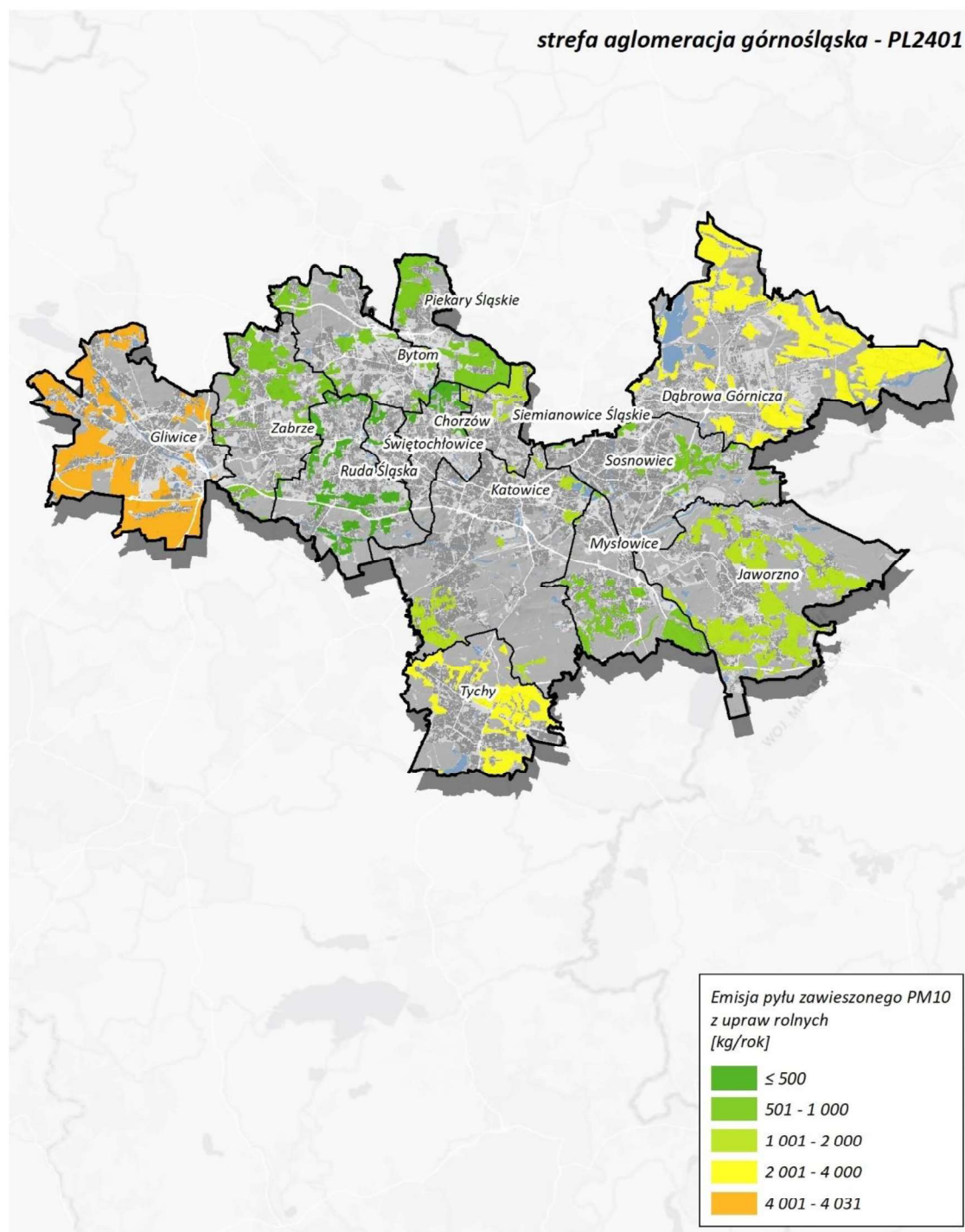
Rysunek 115. Lokalizacja i wielkość emisji pyłu PM10 z upraw rolnych w aglomeracji górnośląskiej w roku bazowym 2022 287
