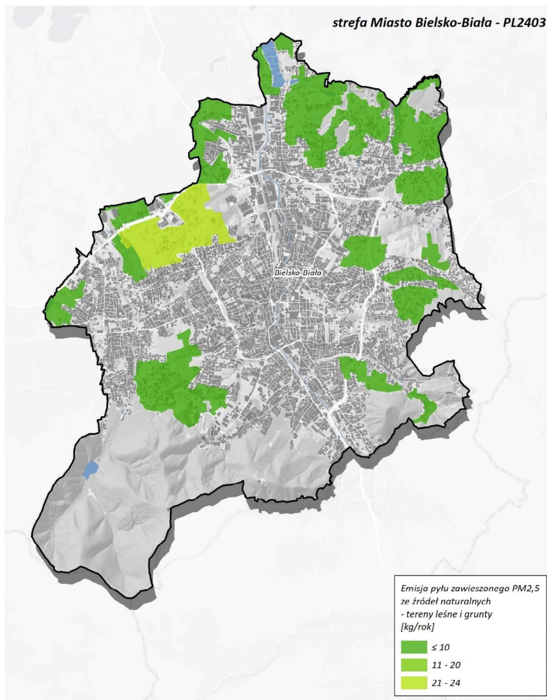
Rysunek 148. Lokalizacja i wielkość emisji pyłu PM 2,5 ze źródeł naturalnych (tereny leśne i grunty) w Bielsku-Białej w roku bazowym 2022 320
