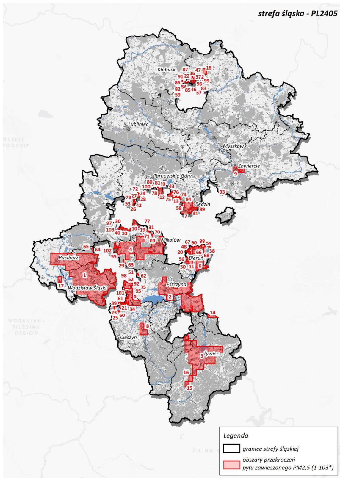
Rysunek 58. Obszary przekroczeń poziomu dopuszczalnego dla pyłu PM 2,5 na terenie strefy śląskiej w 2022 roku 165
