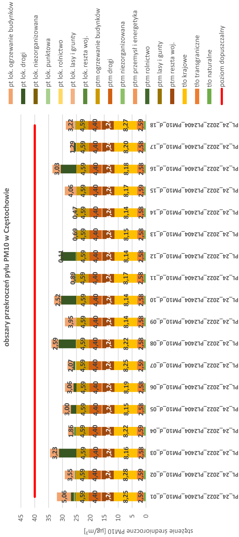
Rysunek 79. Prezentacja poziomów tła regionalnego, przyrostu tła miejskiego oraz lokalnego przyrostu stężeń dla pyłu PM10 w obszarach przekroczeń w Częstochowie w 2022 roku
