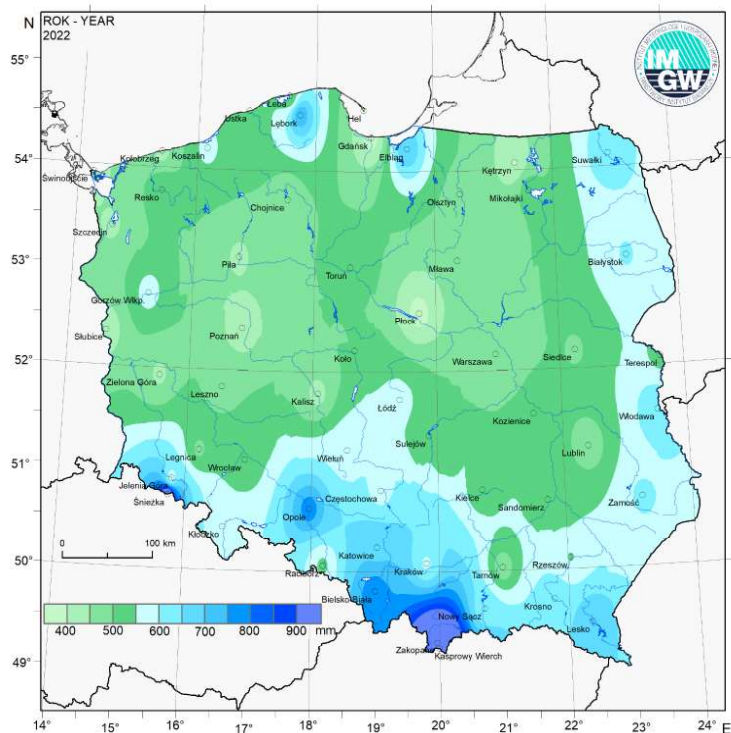
Rysunek 10. Roczne sumy opadów atmosferycznych w roku 2022 63
