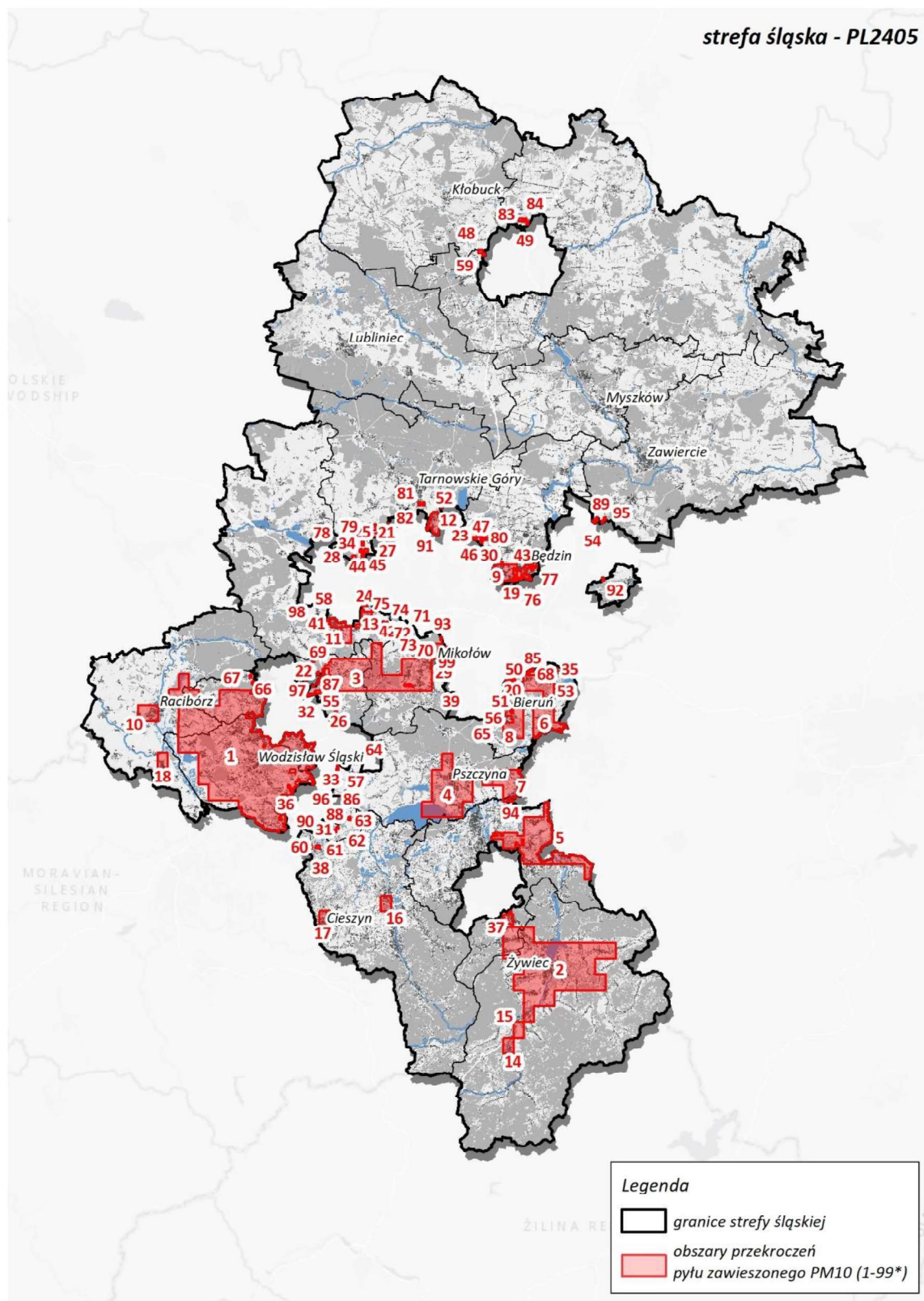
Rysunek 57. Obszary przekroczeń dobowego poziomu dopuszczalnego dla pyłu PM10 na terenie strefy śląskiej w 2022 roku 164
