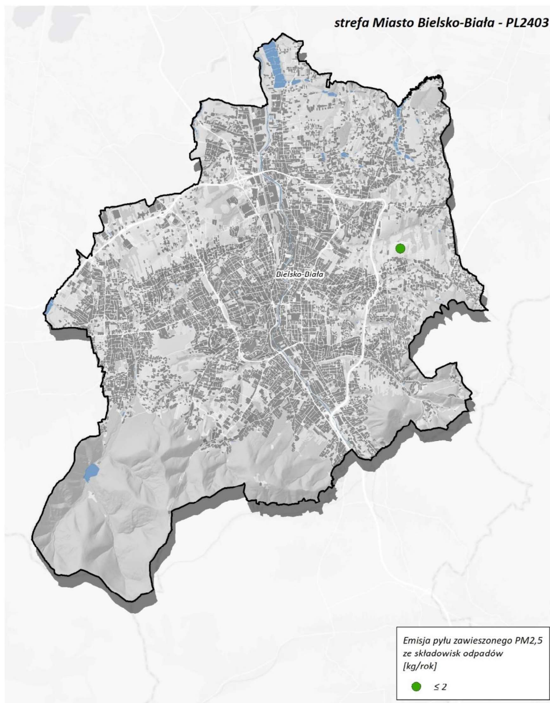
Rysunek 154. Lokalizacja i wielkość emisji pyłu PM 2,5 ze składowisk odpadów w Bielsku-Białej w roku bazowym 2022 326
