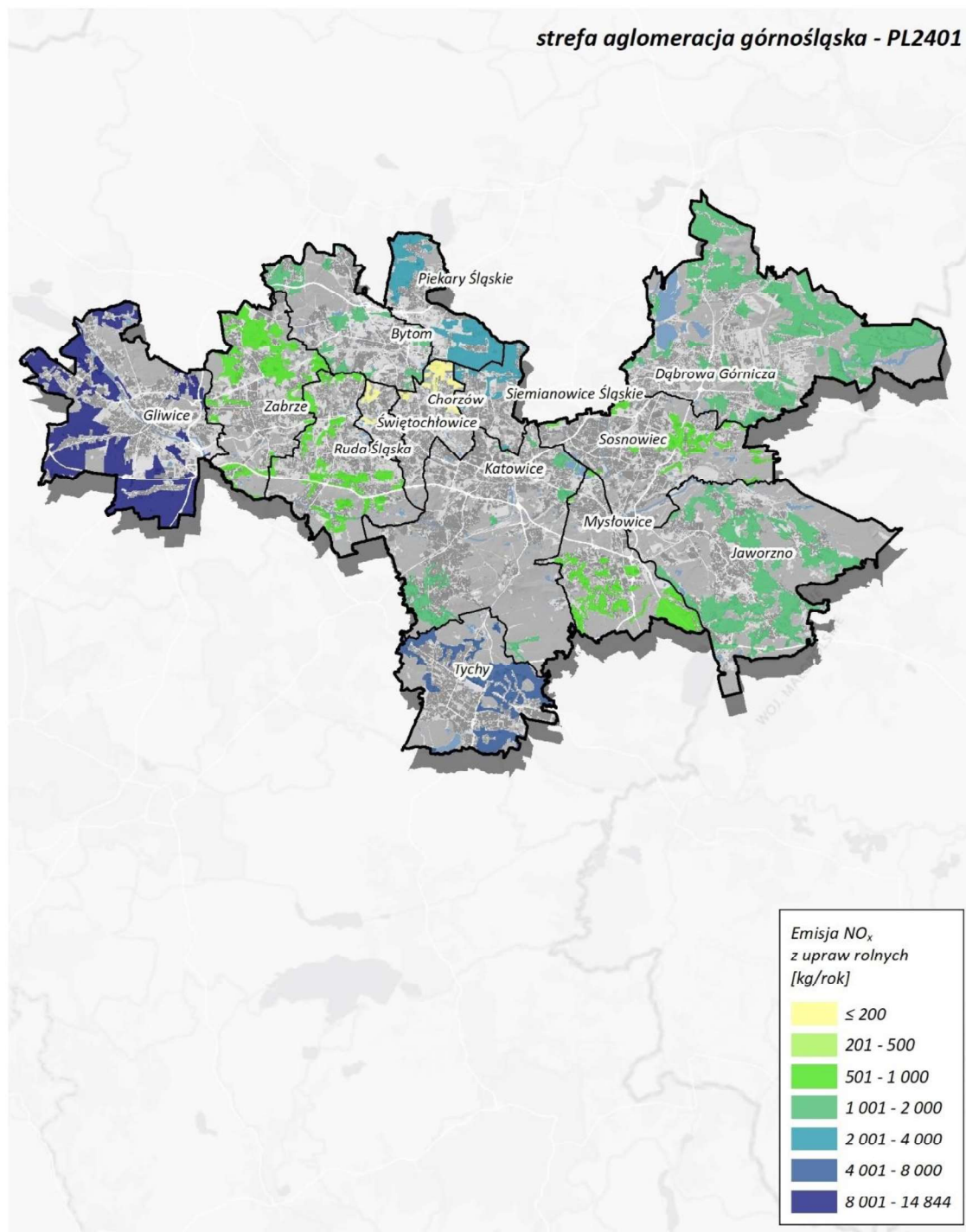
Rysunek 117. Lokalizacja i wielkość emisji NO x z upraw rolnych w aglomeracji górnośląskiej w roku bazowym 2022 289
