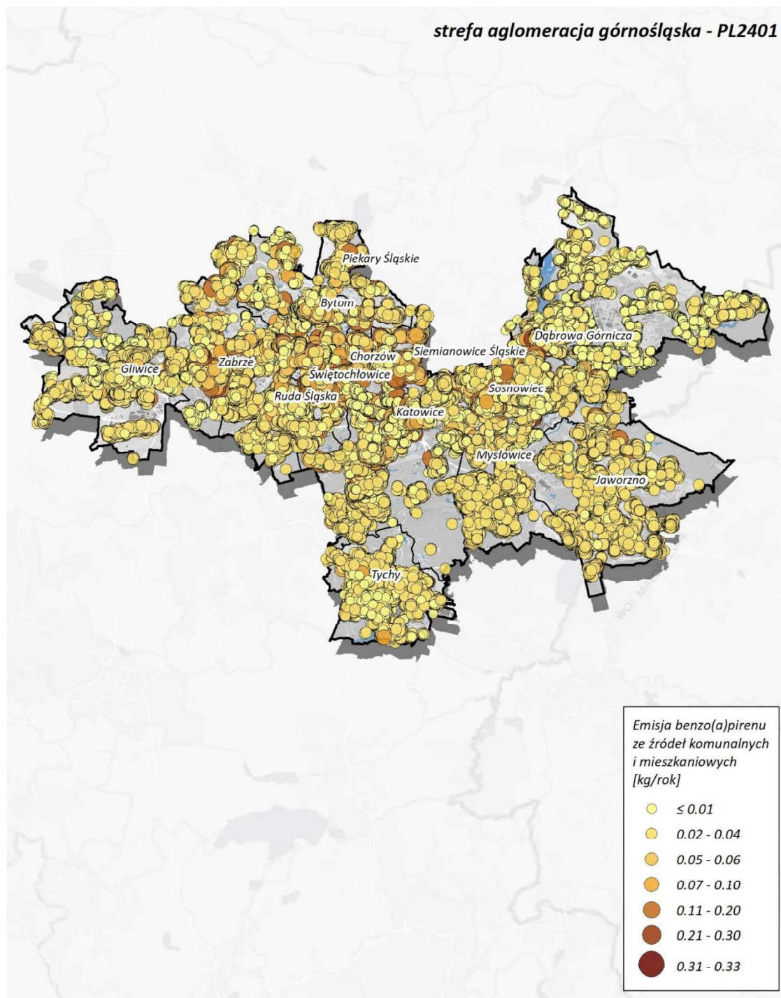
Rysunek 199. Lokalizacja i wielkość emisji B(a)P ze źródeł z sektora komunalno-bytowego w aglomeracji górnośląskiej w roku bazowym 2022 371
