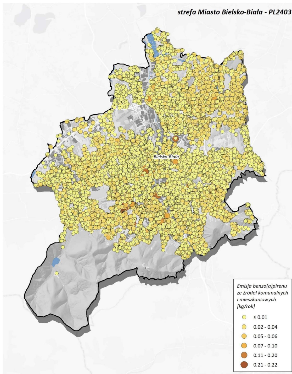
Rysunek 209. Lokalizacja i wielkość emisji B(a)P ze źródeł z sektora komunalno-bytowego w strefie miasto Bielsko-Biała w roku bazowym 2022 381
