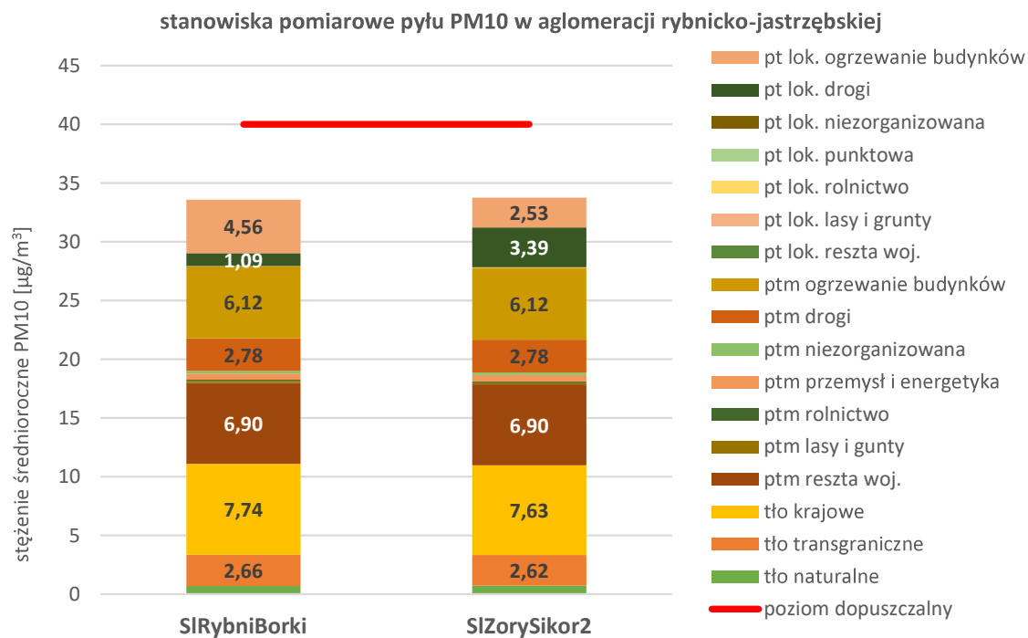
Rysunek 69. Prezentacja poziomów tła regionalnego, przyrostu tła miejskiego oraz lokalnego przyrostu stężeń dla pyłu PM10 na stanowiskach pomiarowych w aglomeracji rybnicko-jastrzębskiej w 2022 roku
