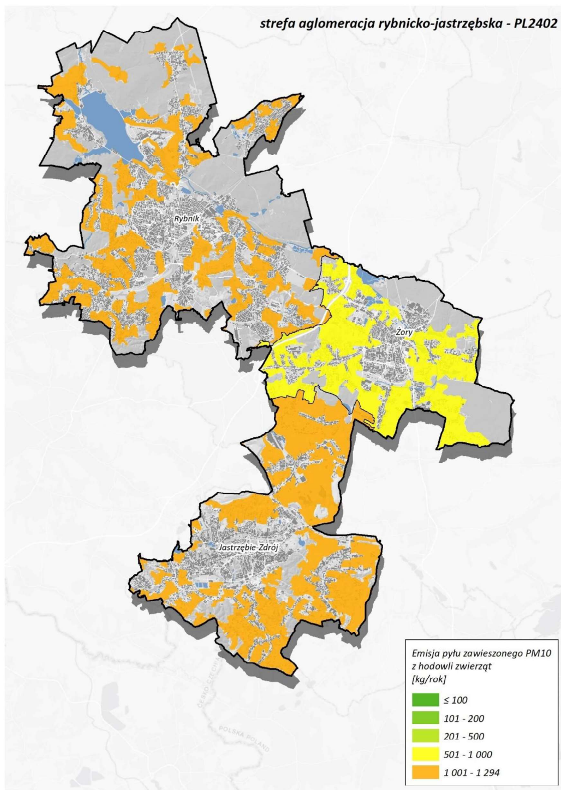
Rysunek 140. Lokalizacja i wielkość emisji pyłu PM10 z hodowli w aglomeracji rybnicko-jastrzębskiej w roku bazowym 2022 312
