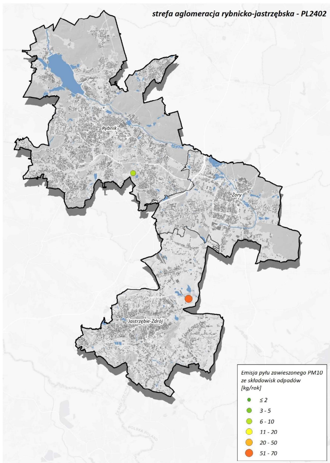
Rysunek 142. Lokalizacja i wielkość emisji pyłu PM10 ze składowisk odpadów w aglomeracji rybnicko-jastrzębskiej w roku bazowym 2022 314
