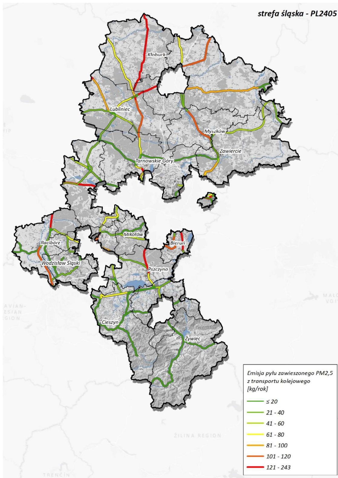
Rysunek 183. Lokalizacja i wielkość emisji pyłu PM 2,5 z kolei w strefie śląskiej w roku bazowym 2022 355
