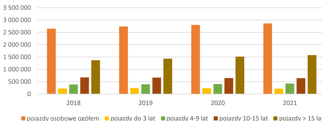
Rysunek 90. Liczba pojazdów osobowych w różnym wieku w województwie śląskim w latach 2018-2021 197
