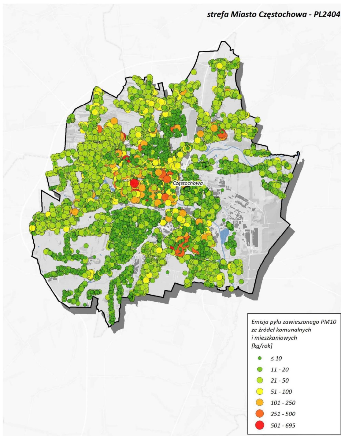
Rysunek 210. Lokalizacja i wielkość emisji pyłu PM10 ze źródeł z sektora komunalno-bytowego w strefie miasto Częstochowa w roku bazowym 2022 382
