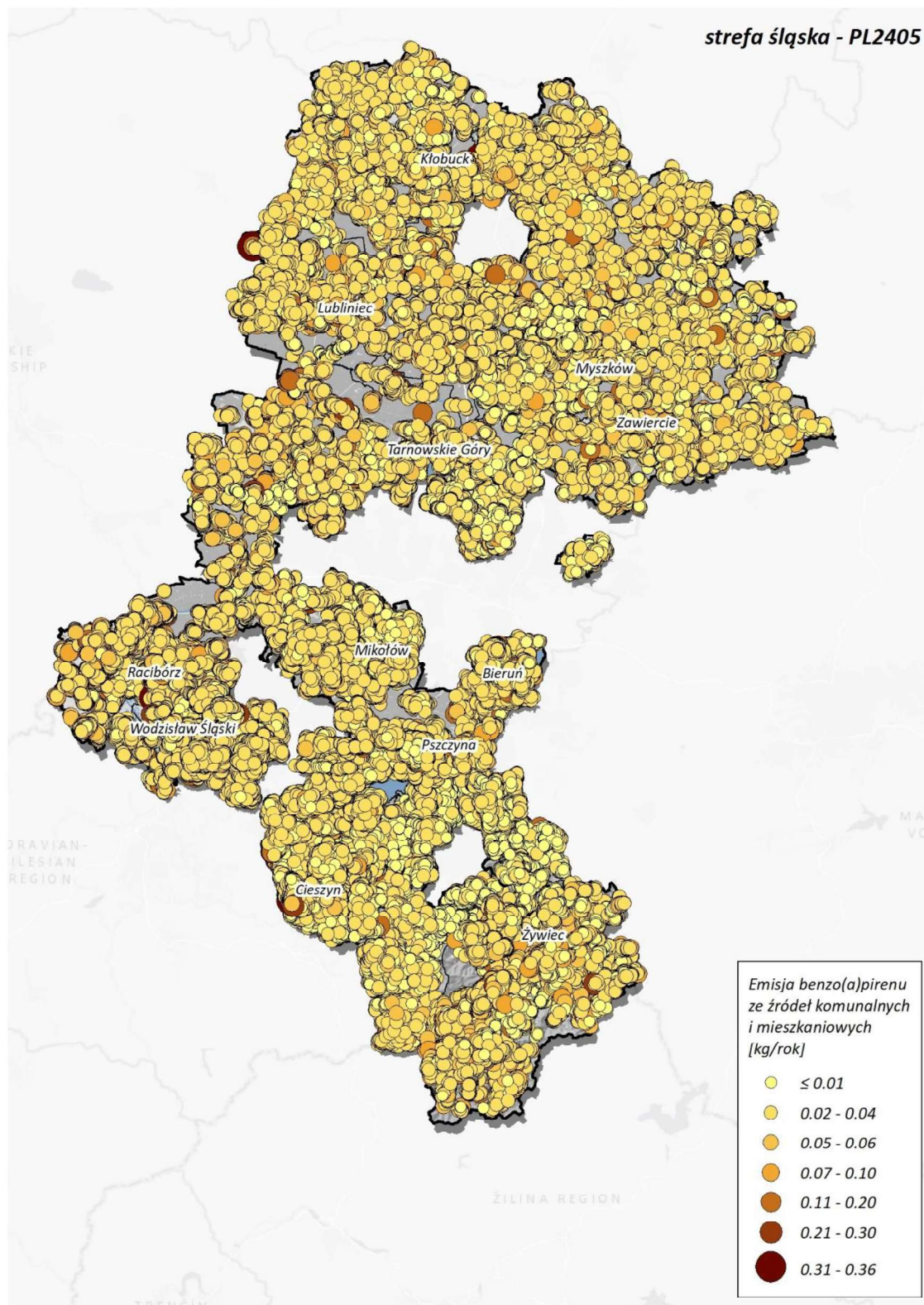
Rysunek 215. Lokalizacja i wielkość emisji B(a)P ze źródeł z sektora komunalno-bytowego w strefie śląskiej w roku bazowym 2022 387
