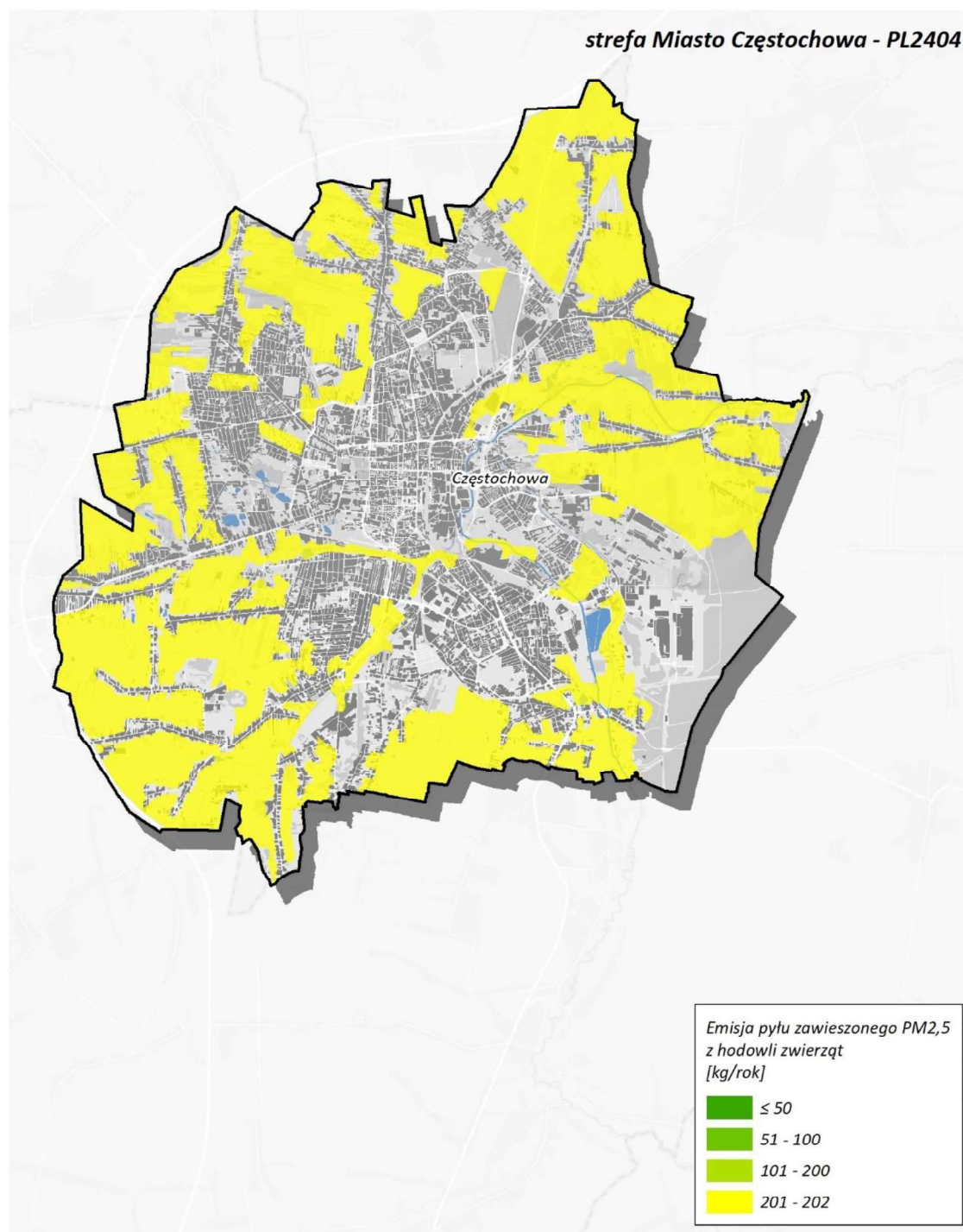
Rysunek 173. Lokalizacja i wielkość emisji pyłu PM 2,5 z hodowli w Częstochowie w roku bazowym 2022 345
