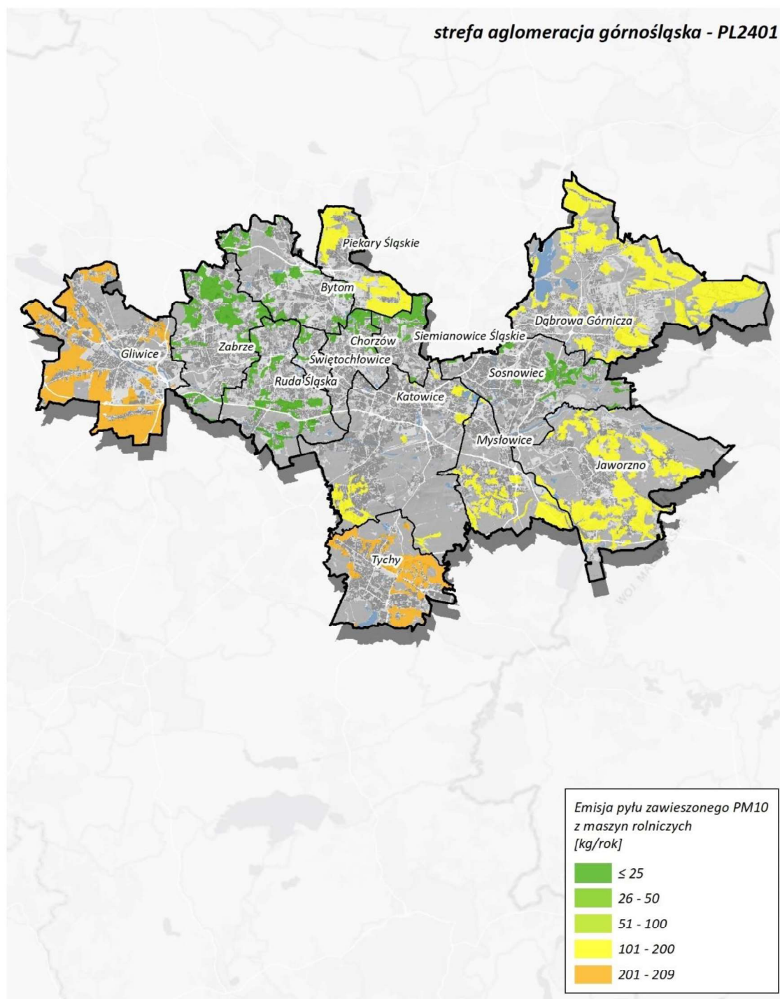
Rysunek 112. Lokalizacja i wielkość emisji pyłu PM10 z maszyn rolniczych w aglomeracji górnośląskiej w roku bazowym 2022 284
