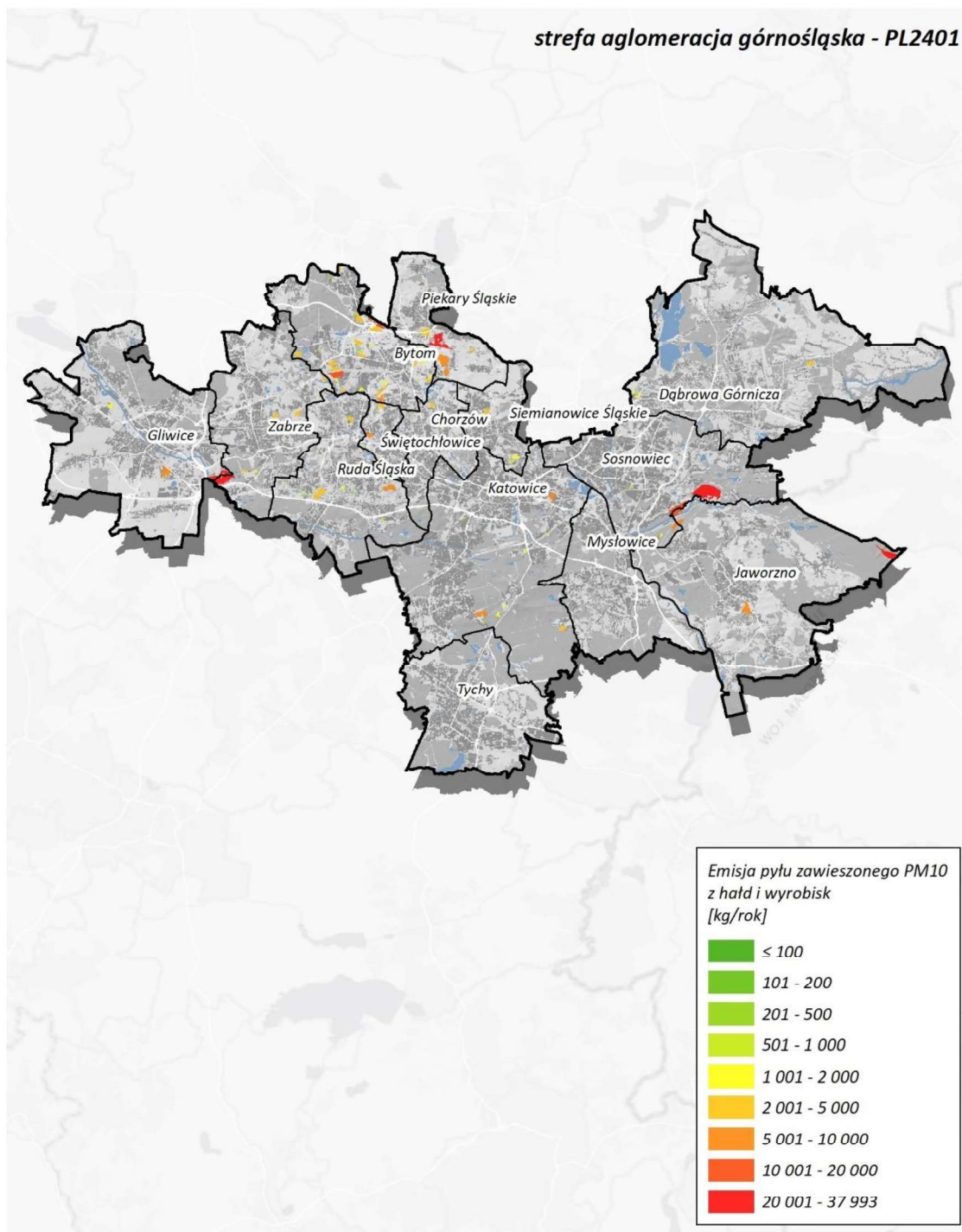
Rysunek 110. Lokalizacja i wielkość emisji pyłu PM10 ze źródeł niezorganizowanych (kopalnie odkrywkowe, hałdy i wyrobiska) w aglomeracji górnośląskiej w roku bazowym 2022 282
