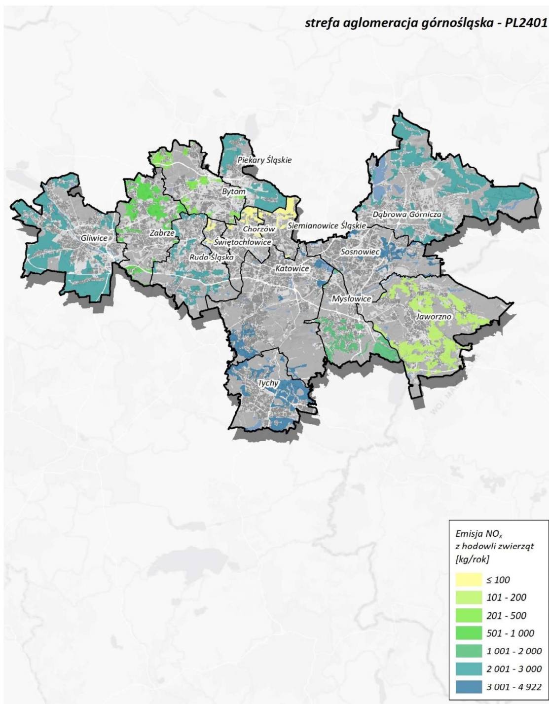
Rysunek 120. Lokalizacja i wielkość emisji NO x z hodowli w aglomeracji górnośląskiej w roku bazowym 2022 292
