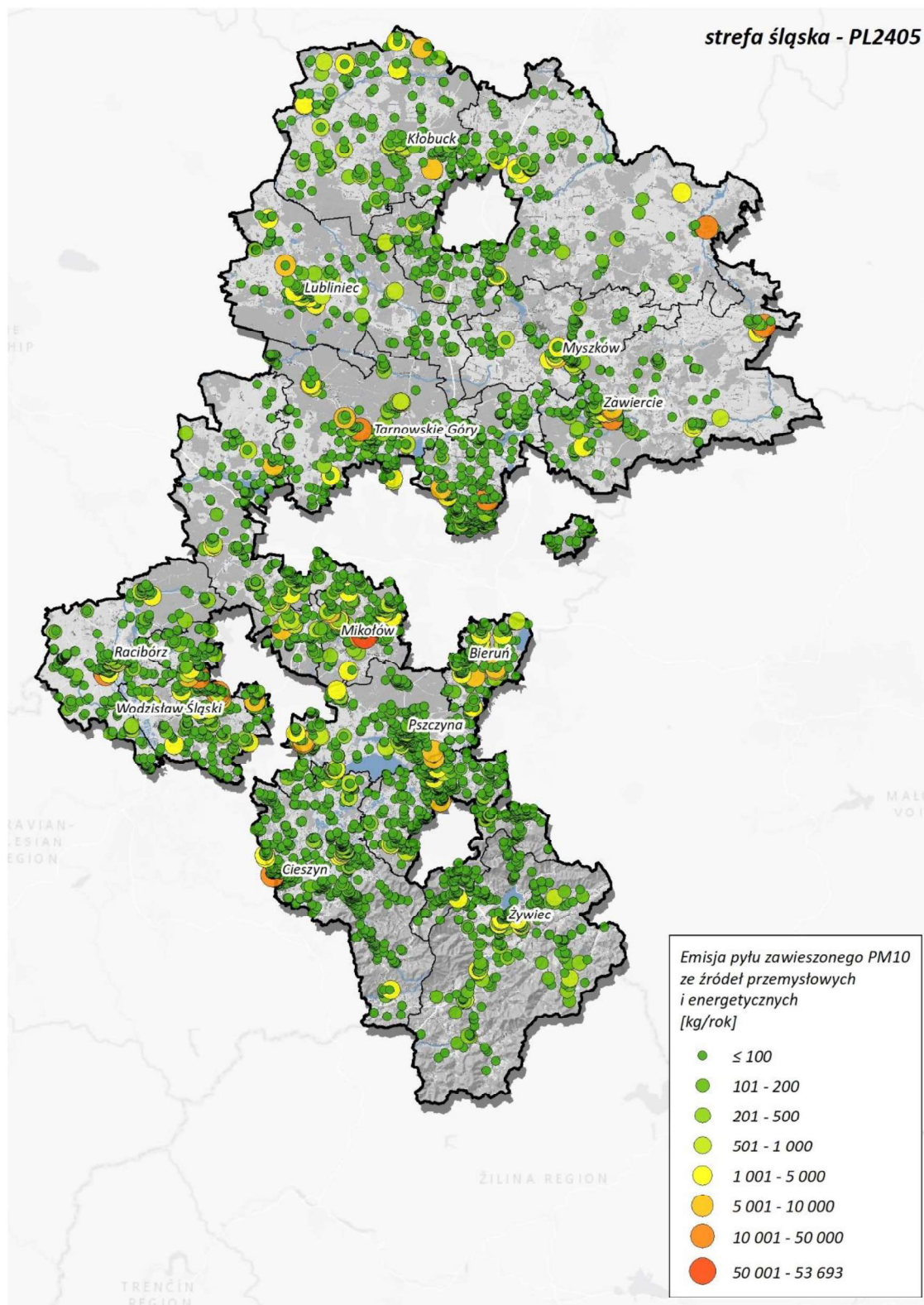
Rysunek 177. Lokalizacja i wielkość emisji pyłu PM10 z przemysłu i energetyki w strefie śląskiej w roku bazowym 2022 349
