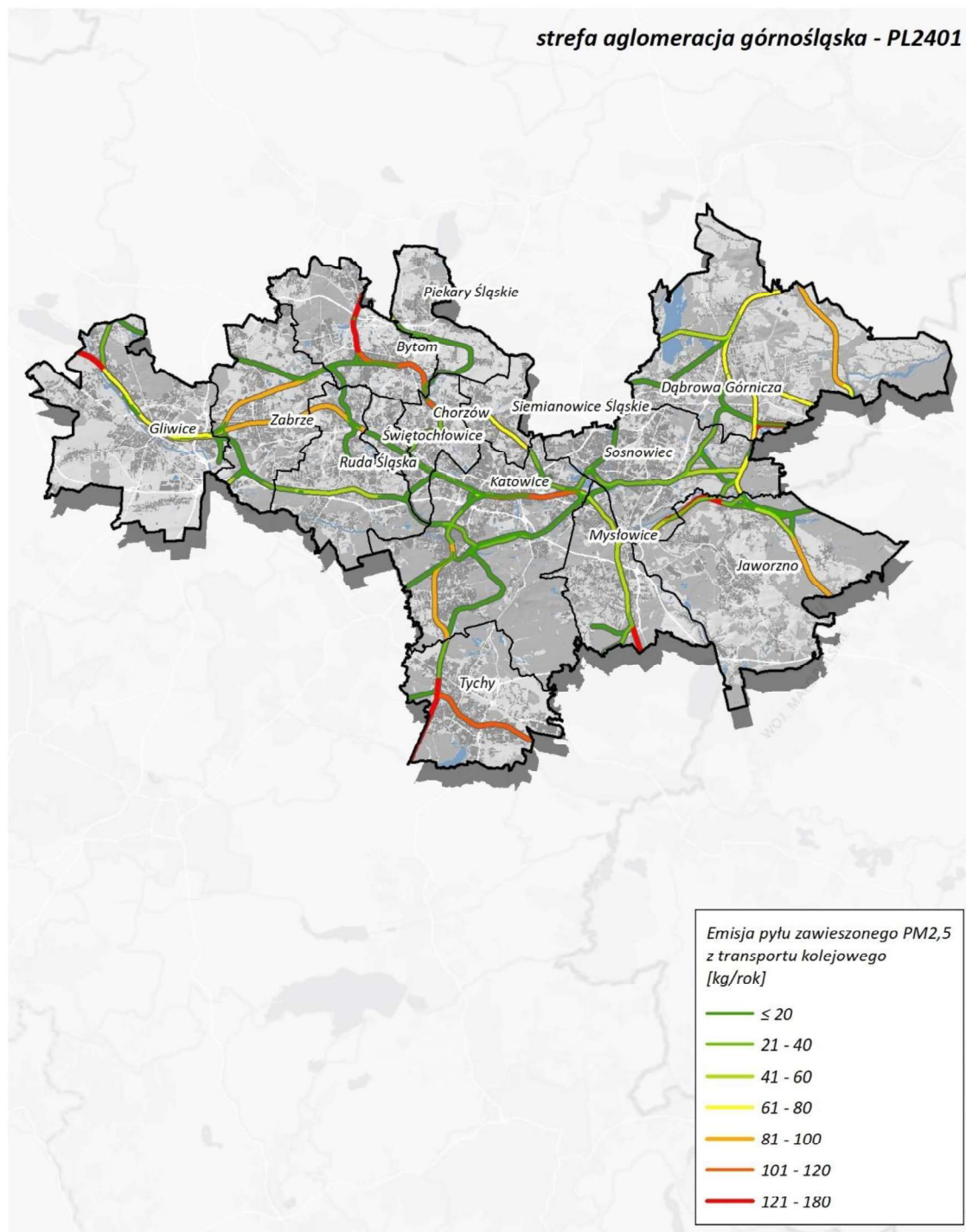
Rysunek 107. Lokalizacja i wielkość emisji pyłu PM 2,5 z kolei w aglomeracji górnośląskiej w roku bazowym 2022 279
