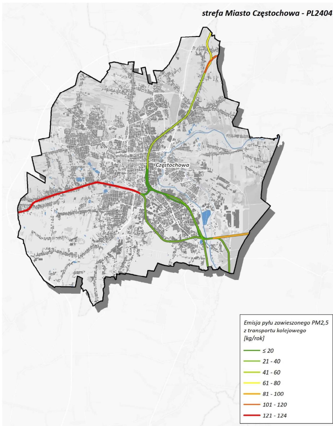
Rysunek 164. Lokalizacja i wielkość emisji pyłu PM 2,5 z kolei w Częstochowie w roku bazowym 2022 336
