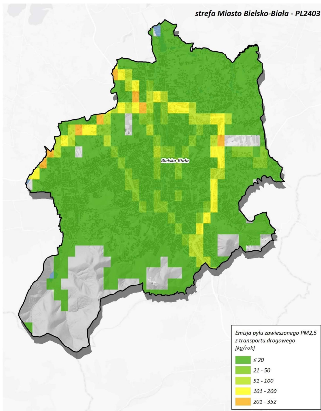
Rysunek 144. Lokalizacja i wielkość emisji pyłu PM 2,5 z sektora transportu drogowego w Bielsku-Białej w roku bazowym 2022 316
