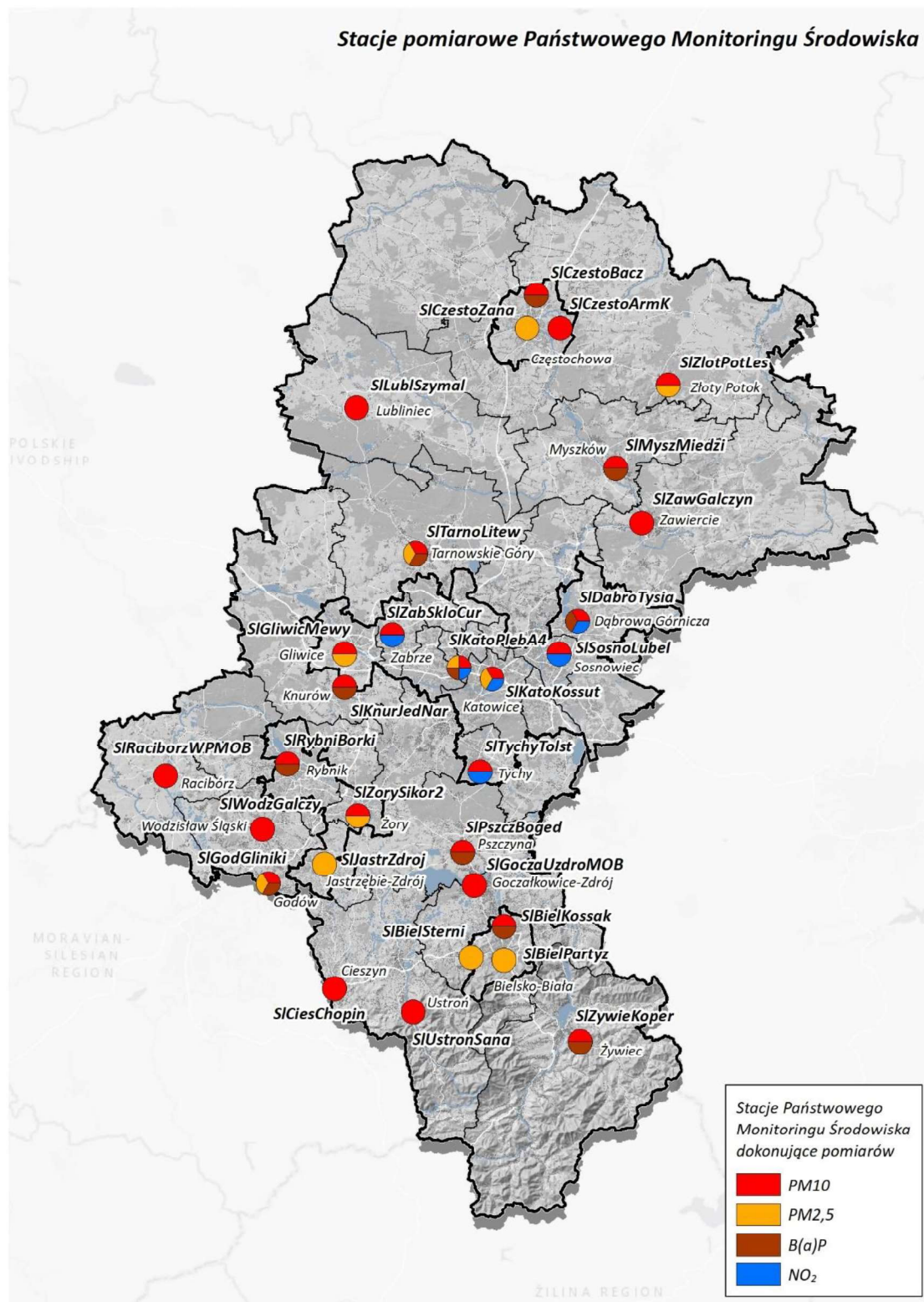
Rysunek 99. Lokalizacja punktów pomiarowych na terenie wszystkich stref w województwie śląskim 271
