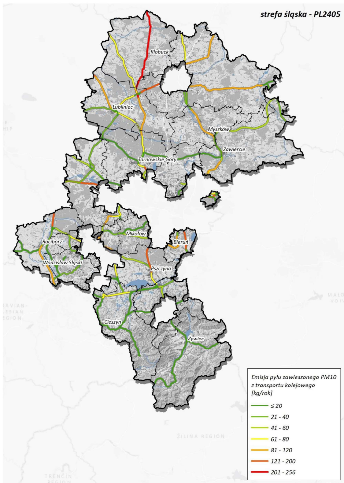
Rysunek 182. Lokalizacja i wielkość emisji pyłu PM10 z kolei w strefie śląskiej w roku bazowym 2022 354
