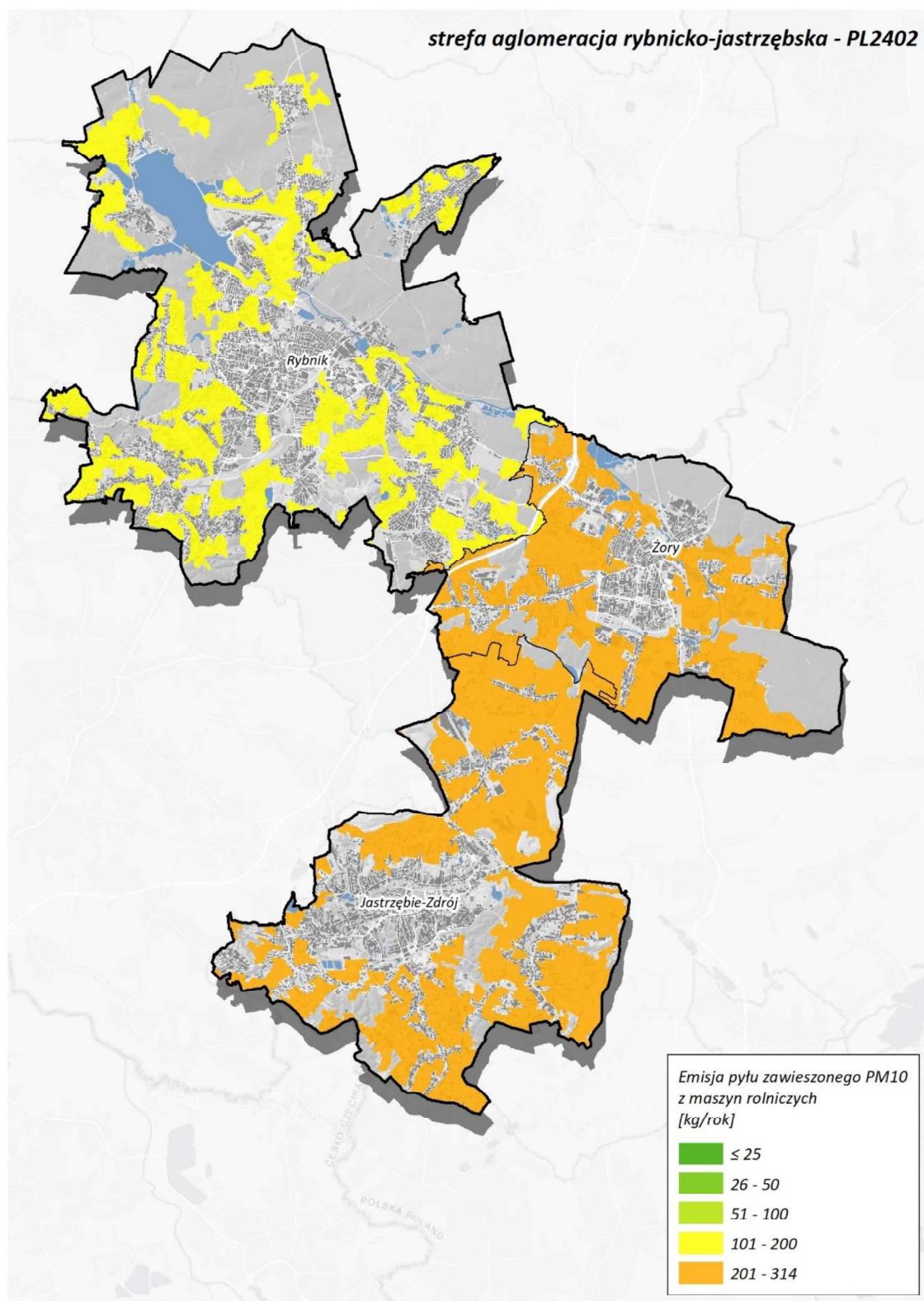
Rysunek 136. Lokalizacja i wielkość emisji pyłu PM10 z maszyn rolniczych w aglomeracji rybnicko-jastrzębskiej w roku bazowym 2022 308
