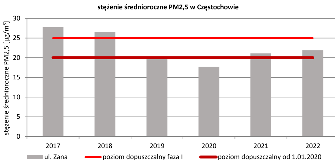
Rysunek 36. Wyniki pomiarów stężeń średniorocznych pyłu PM2,5 w latach 2017-2022 w strefie miasto Częstochowa 122
