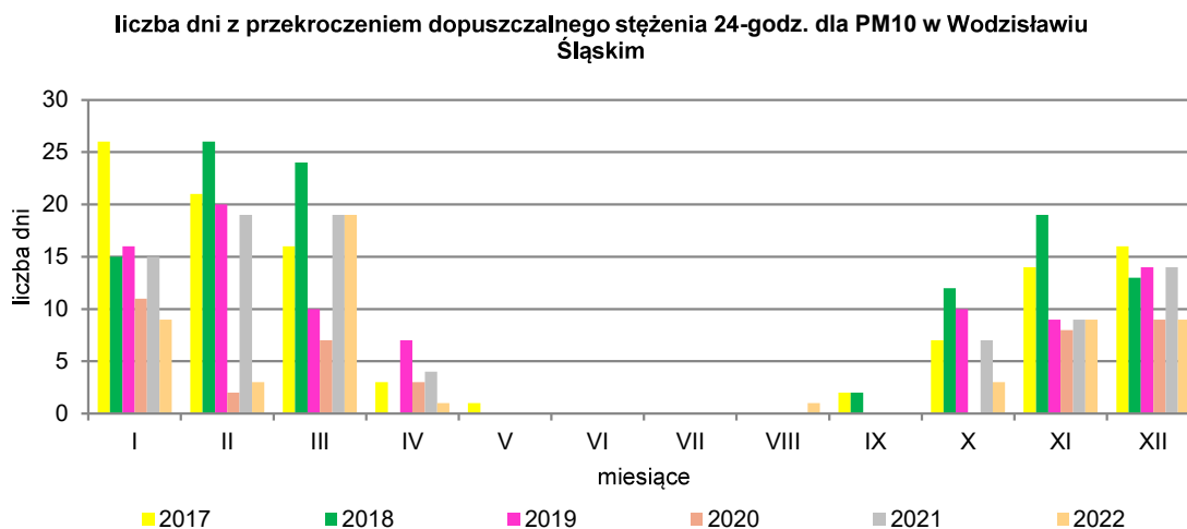
Rysunek 41. Liczba dni z przekroczeniem dopuszczalnego stężenia dobowego pyłu PM10 w ujęciu miesięcznym na stacji pomiarowej w Wodzisławiu Śląskim w latach 2017-2022
