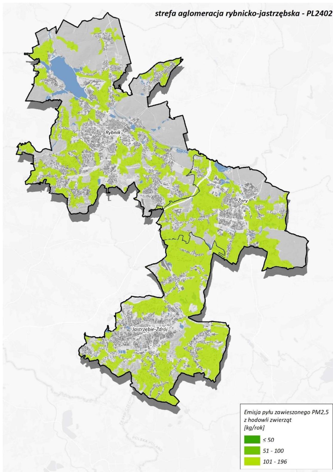
Rysunek 141. Lokalizacja i wielkość emisji pyłu PM 2,5 z hodowli w aglomeracji rybnicko-jastrzębskiej w roku bazowym 2022 313
