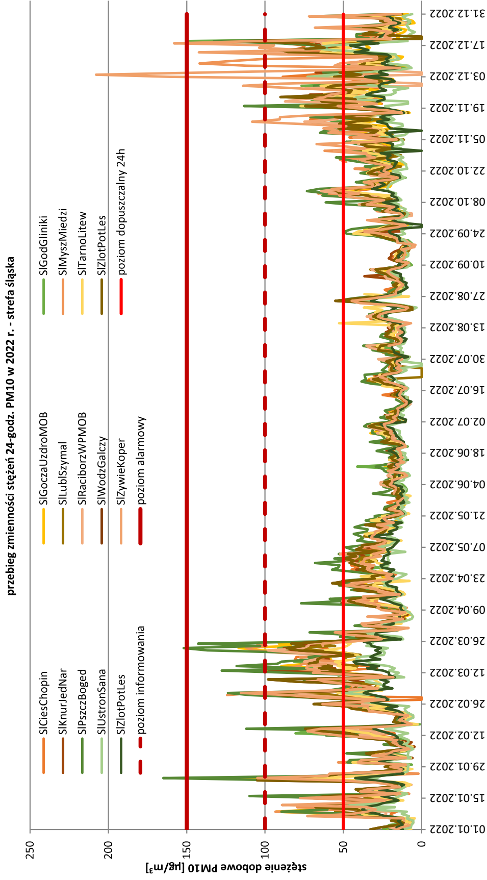
Rysunek 42. Przebieg zmienności stężeń 24-godzinnych w 2022 r. na stacjach pomiarowych w strefie śląskiej 134
