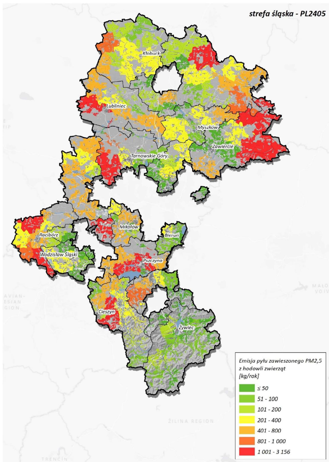
Rysunek 192. Lokalizacja i wielkość emisji pyłu PM 2,5 z hodowli w strefie śląskiej w roku bazowym 2022 364
