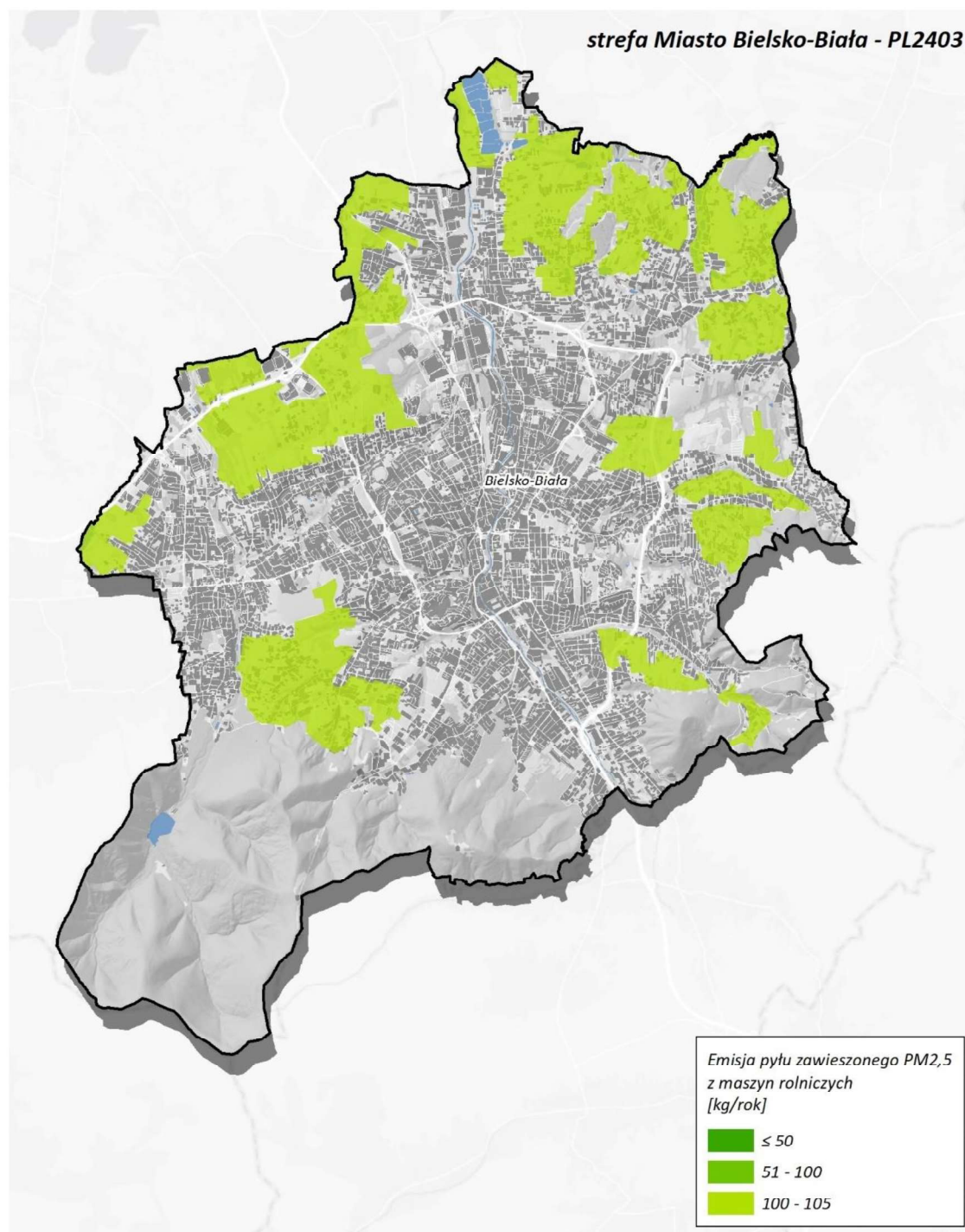
Rysunek 151. Lokalizacja i wielkość emisji pyłu PM 2,5 z maszyn rolniczych w Bielsku-Białej w roku bazowym 2022 323
