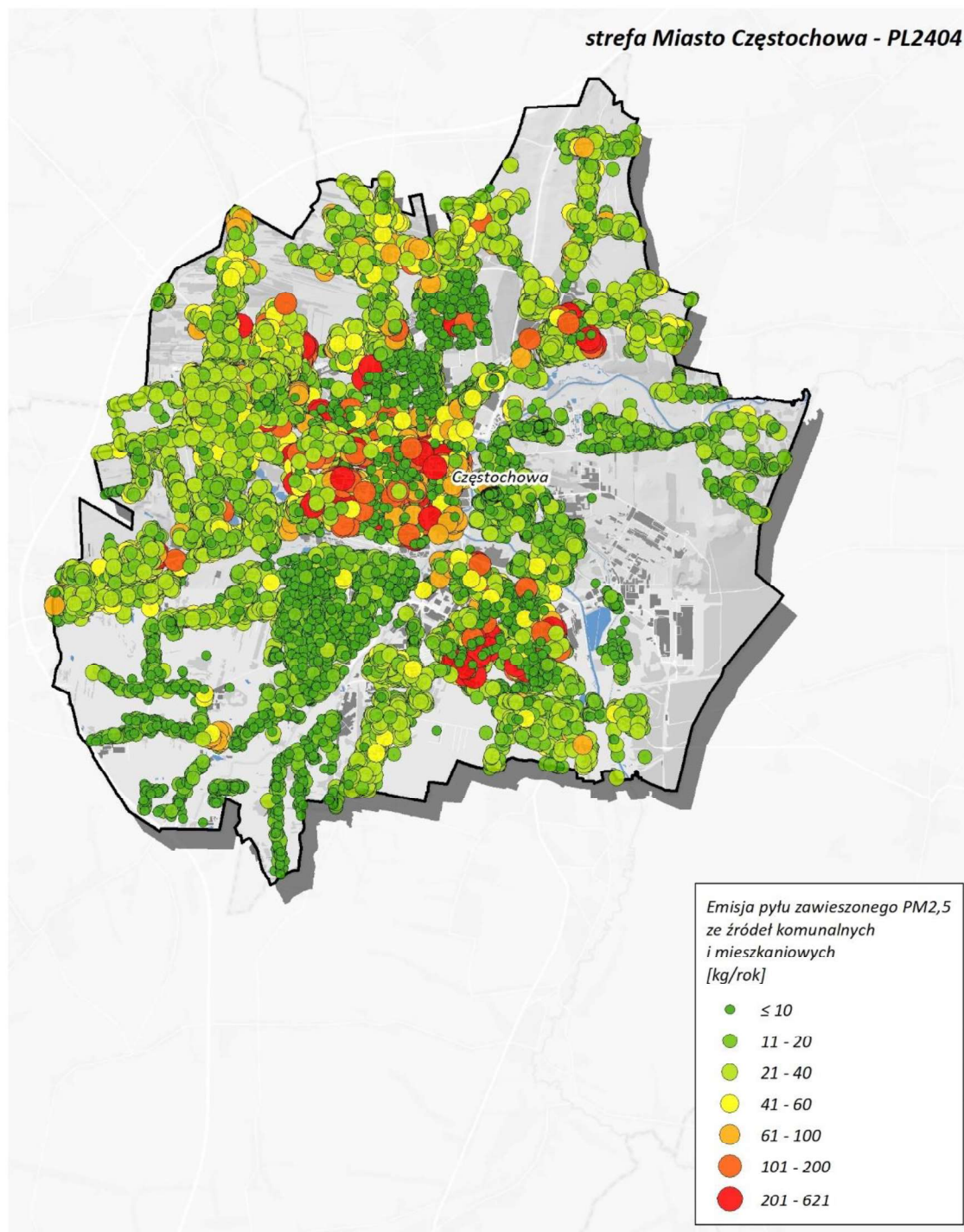
Rysunek 211. Lokalizacja i wielkość emisji pyłu PM 2,5 ze źródeł z sektora komunalno-bytowego w strefie miasto Częstochowa w roku bazowym 2022 383
