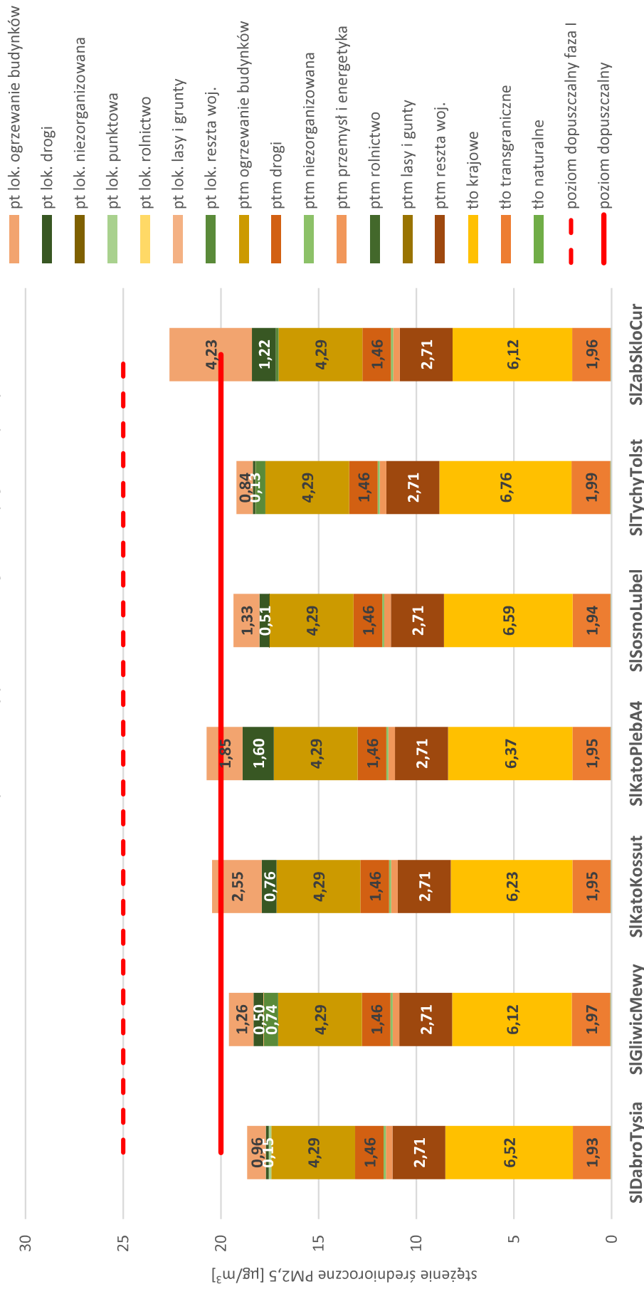
stanowiska pomiarowe pyłu PM2,5 w aglomeracji górnośląskiej
