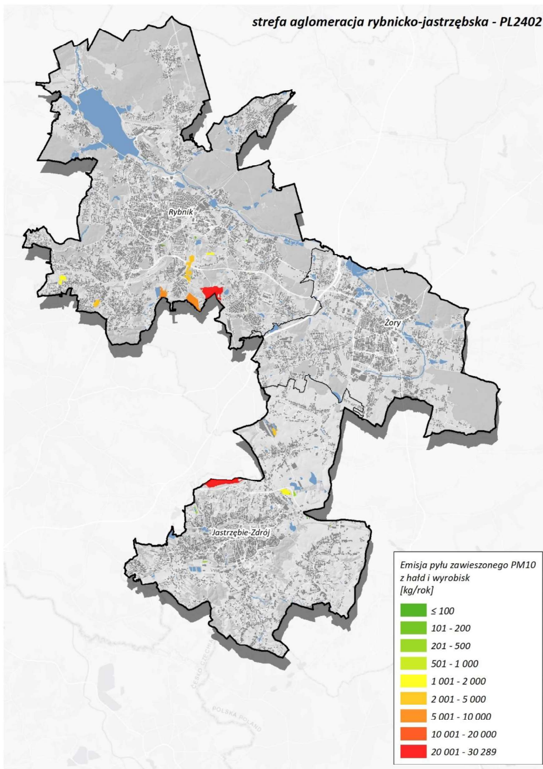
Rysunek 134. Lokalizacja i wielkość emisji pyłu PM10 ze źródeł niezorganizowanych (kopalnie odkrywkowe, hałdy i wyrobiska) w aglomeracji rybnicko-jastrzębskiej w roku bazowym 2022 306
