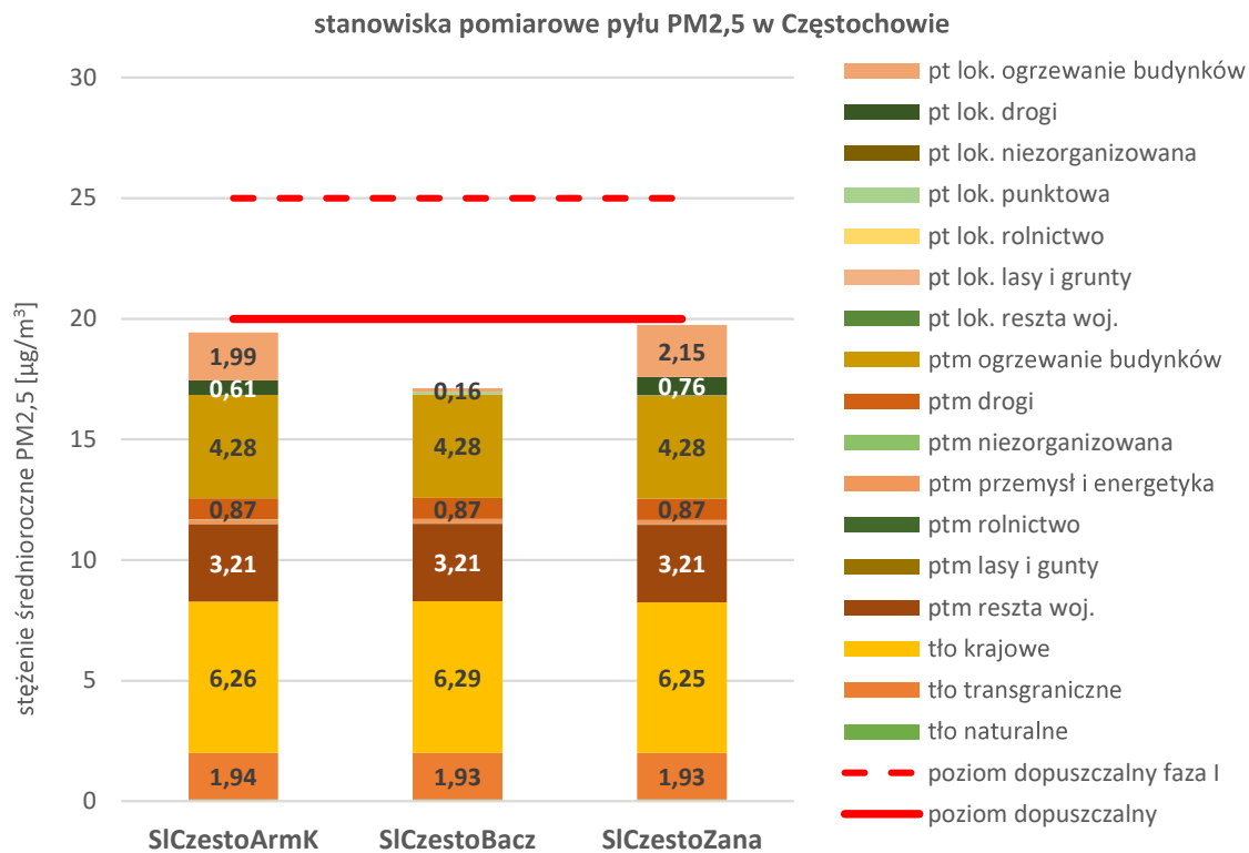
Rysunek 77. Prezentacja poziomów tła regionalnego, przyrostu tła miejskiego oraz lokalnego przyrostu stężeń pyłu PM 2,5 na stanowiskach pomiarowych w Częstochowie w 2022 roku 181
