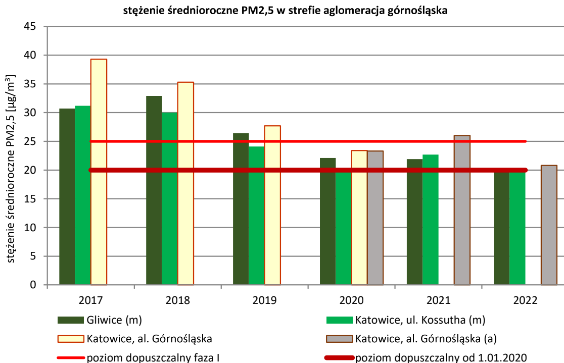
Rysunek 18. Wyniki pomiarów stężeń średniorocznych pyłu zawieszony PM 2,5 w latach 2017-2022 w strefie aglomeracja górnośląska 76
