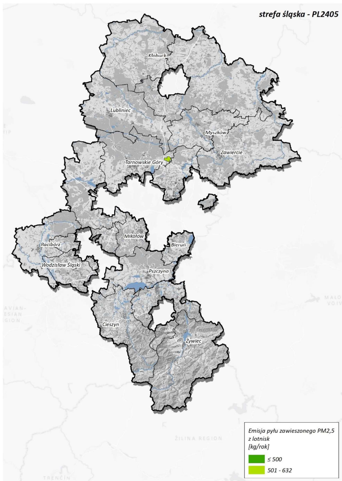
Rysunek 194. Lokalizacja i wielkość emisji pyłu PM2,5 z lotnisk w strefie śląskiej w roku bazowym 2022 366
