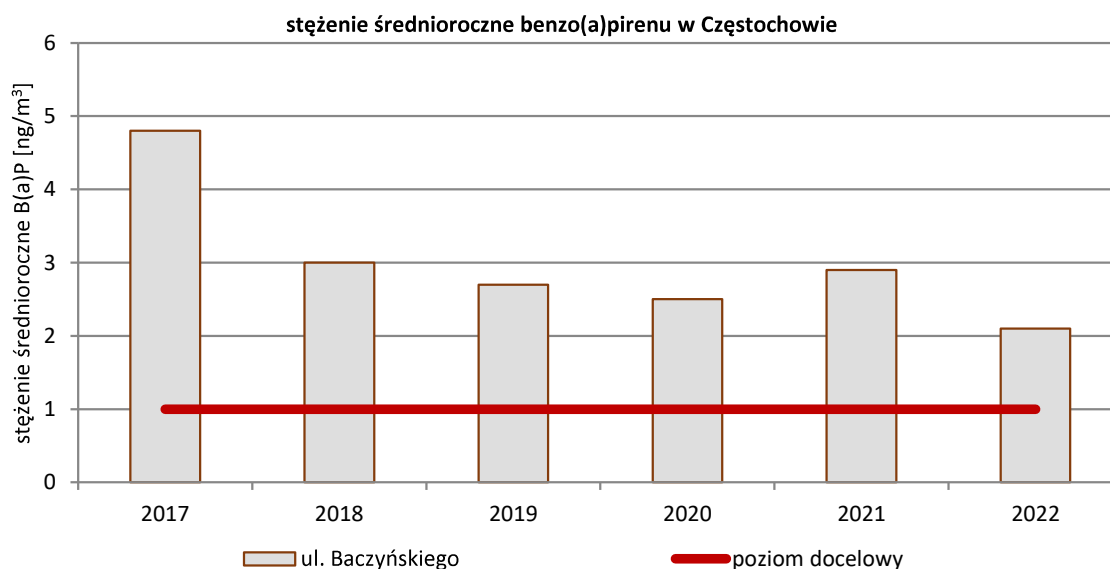
Rysunek 37. Wyniki pomiarów stężeń średniorocznych benzo(a)pirenu w latach 2017-2022 w strefie miasto Częstochowa 125
