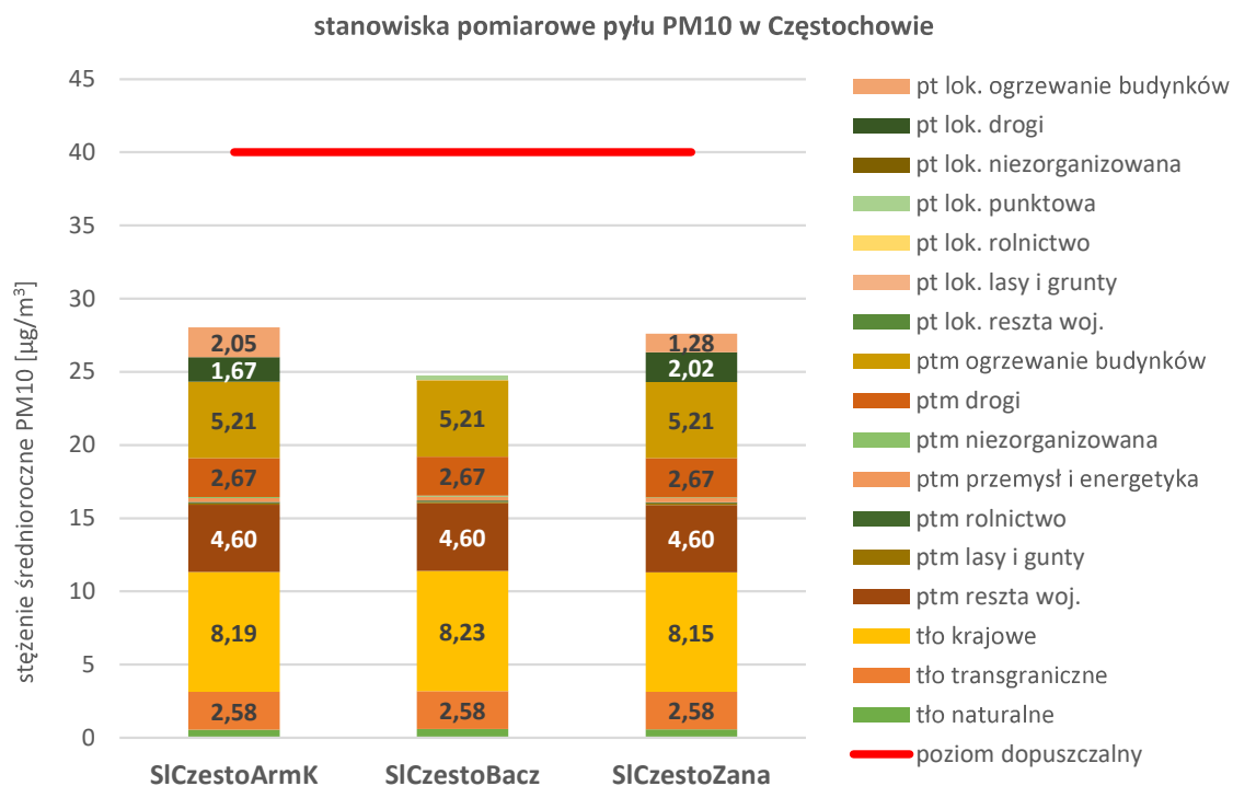
Rysunek 76. Prezentacja poziomów tła regionalnego, przyrostu tła miejskiego oraz lokalnego przyrostu stężeń dla pyłu PM10 na stanowiskach pomiarowych w Częstochowie w 2022 roku 180
