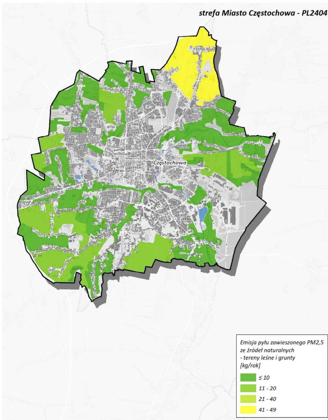
Rysunek 162. Lokalizacja i wielkość emisji pyłu PM 2,5 ze źródeł naturalnych w Częstochowie w roku bazowym 2022 334
