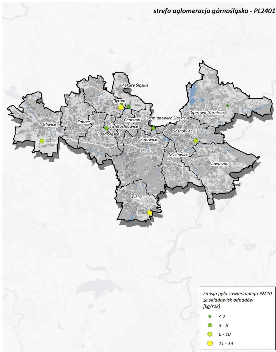
Rysunek 121. Lokalizacja i wielkość emisji pyłu PM10 ze składowisk odpadów w aglomeracji górnośląskiej w roku bazowym 2022 293
