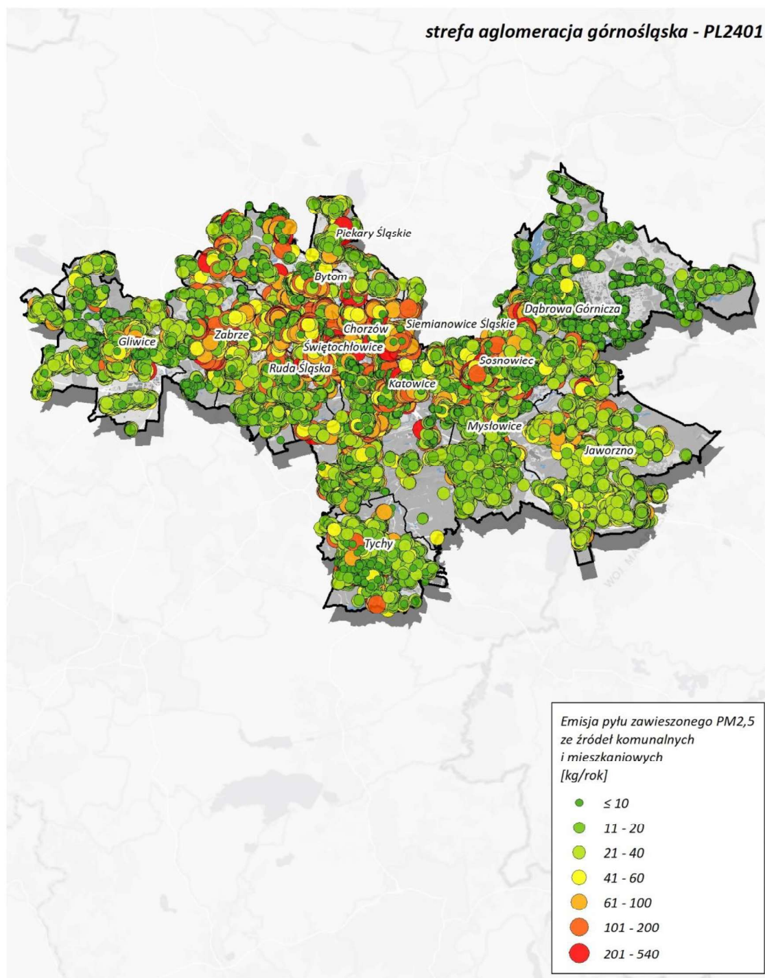
Rysunek 198. Lokalizacja i wielkość emisji pyłu PM 2,5 ze źródeł z sektora komunalno-bytowego w aglomeracji górnośląskiej w roku bazowym 2022 370
