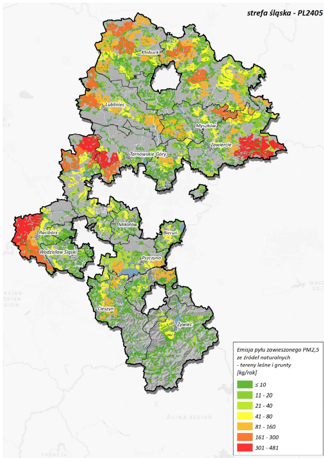
Rysunek 181. Lokalizacja i wielkość emisji pyłu PM 2,5 ze źródeł naturalnych w strefie śląskiej w roku bazowym 2022 353
