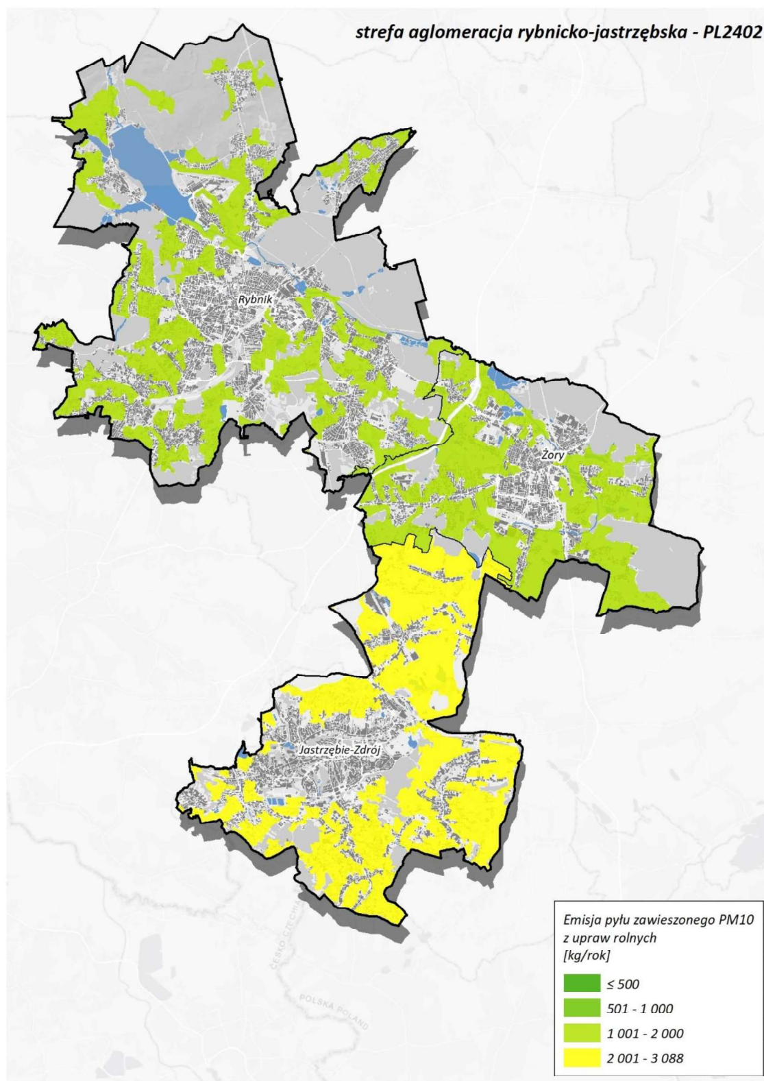
Rysunek 138. Lokalizacja i wielkość emisji pyłu PM10 z upraw rolnych w aglomeracji rybnicko-jastrzębskiej w roku bazowym 2022 310
