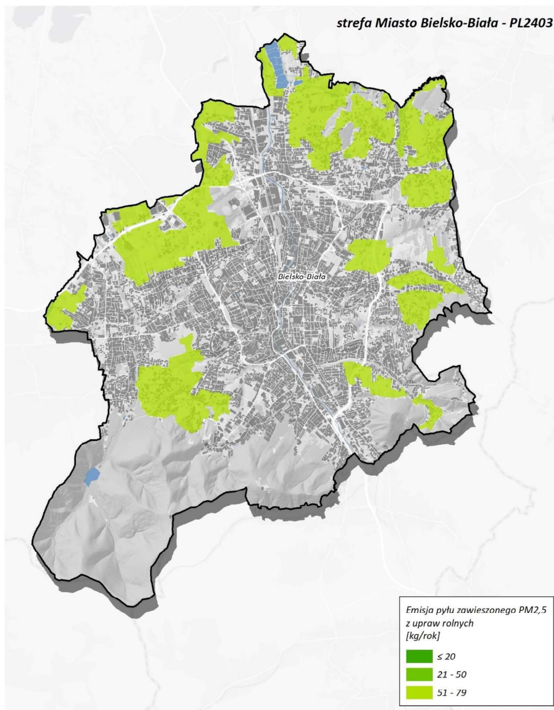
Rysunek 152. Lokalizacja i wielkość emisji pyłu PM 2,5 z upraw rolnych w Bielsku-Białej w roku bazowym 2022 324
