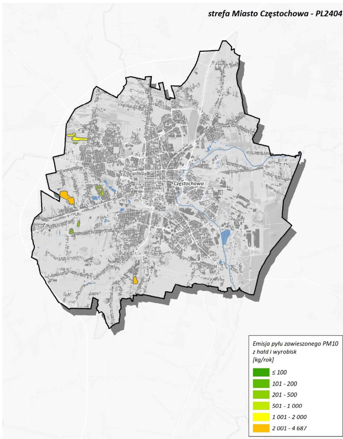
Rysunek 166. Lokalizacja i wielkość emisji pyłu PM10 ze źródeł niezorganizowanych (hałdy i wyrobiska) w Częstochowie w roku bazowym 2022 338
