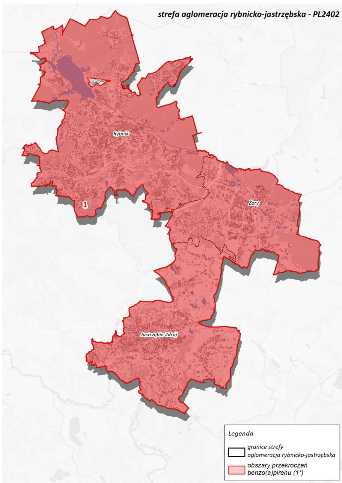
Rysunek 51. Obszary przekroczeń poziomu docelowego benzo(a)pirenu na terenie aglomeracji rybnicko-jastrzębskiej w 2022 roku 150
