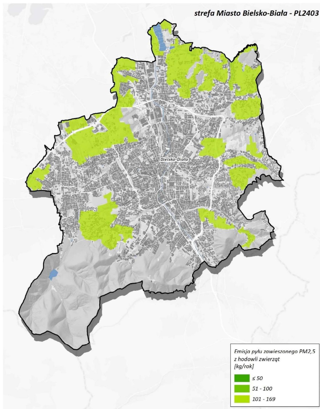
Rysunek 153. Lokalizacja i wielkość emisji pyłu PM 2,5 z hodowli w Bielsku-Białej w roku bazowym 2022 325
