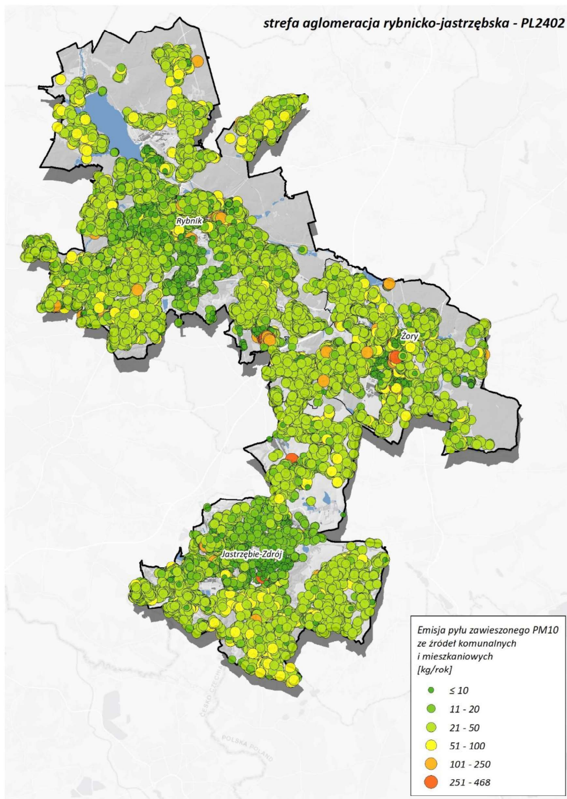
Rysunek 205. Lokalizacja i wielkość emisji pyłu PM10 ze źródeł z sektora komunalno-bytowego w aglomeracji rybnicko-jastrzębskiej w roku bazowym 2022 377
