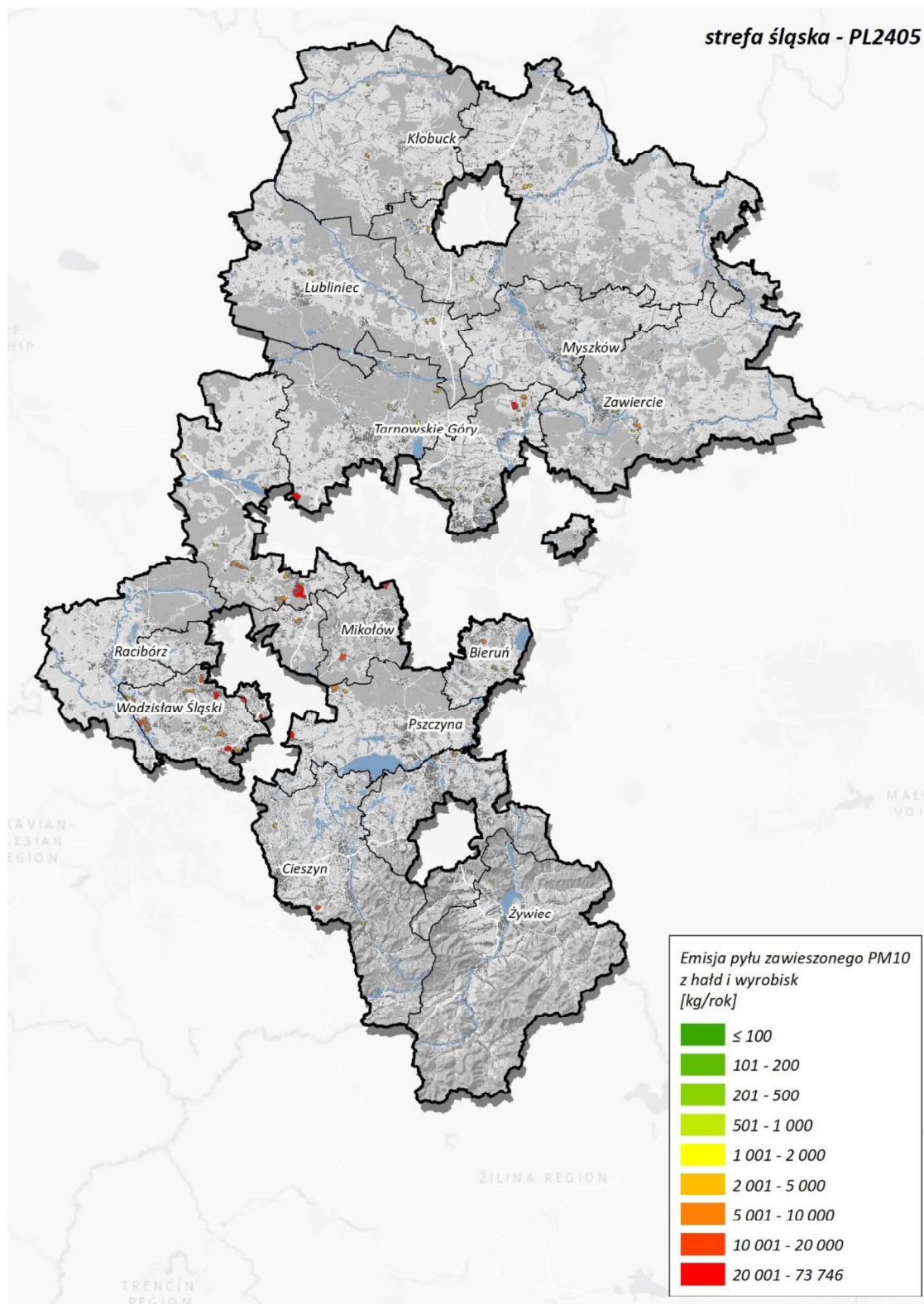
Rysunek 185. Lokalizacja i wielkość emisji pyłu PM10 ze źródeł niezorganizowanych (kopalnie odkrywkowe, hałdy i wyrobiska) w strefie śląskiej w roku bazowym 2022 357
