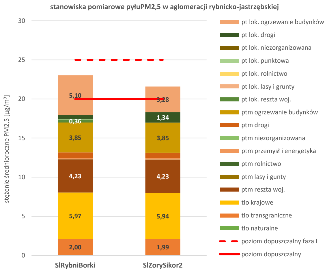
Rysunek 70. Prezentacja poziomów tła regionalnego, przyrostu tła miejskiego oraz lokalnego przyrostu stężeń na stanowiskach pomiarowych na terenie obszaru przekroczeń pyłu PM 2,5 w aglomeracji rybnicko-jastrzębskiej w 2022 roku 176
