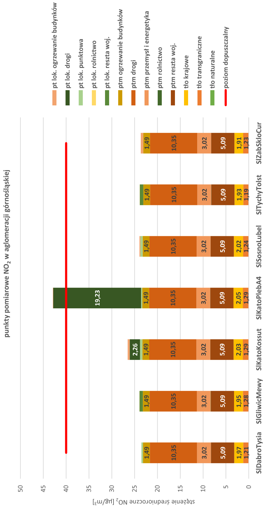
Rysunek 68. Prezentacja poziomów tła regionalnego, przyrostu tła miejskiego oraz lokalnego przyrostu stężeń w punktach pomiarowych NO 2 , w tym na terenie obszaru przekroczeń NO 2 w aglomeracji górnośląskiej w 2022 roku 175
