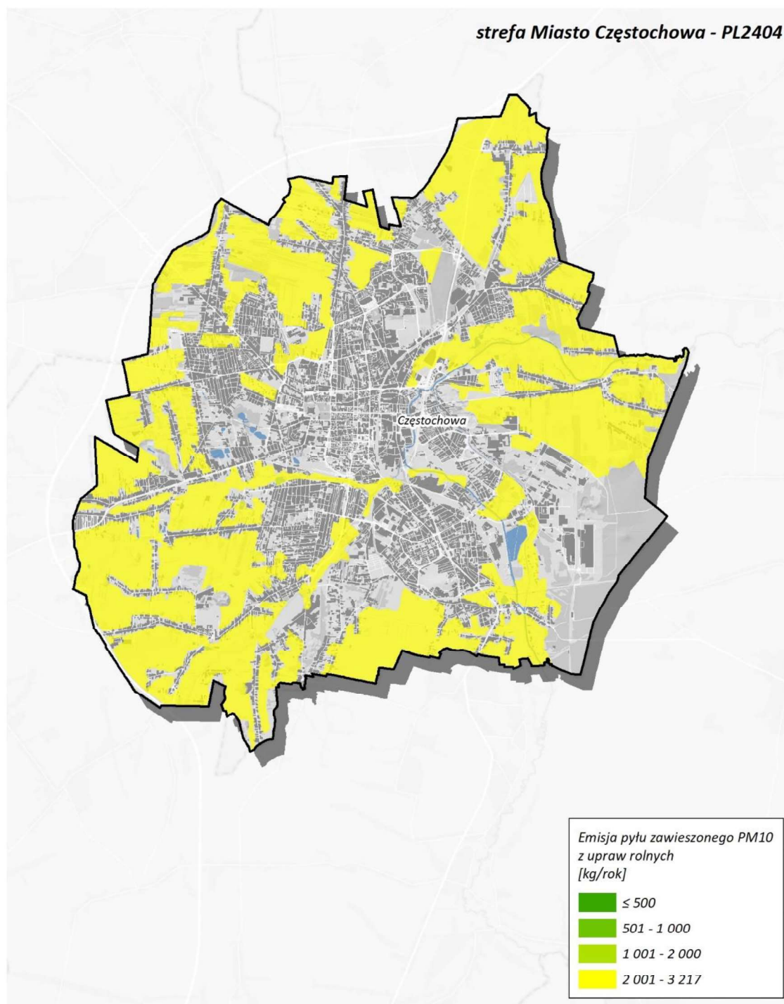
Rysunek 170. Lokalizacja i wielkość emisji pyłu PM10 z upraw rolnych w Częstochowie w roku bazowym 2022 342
