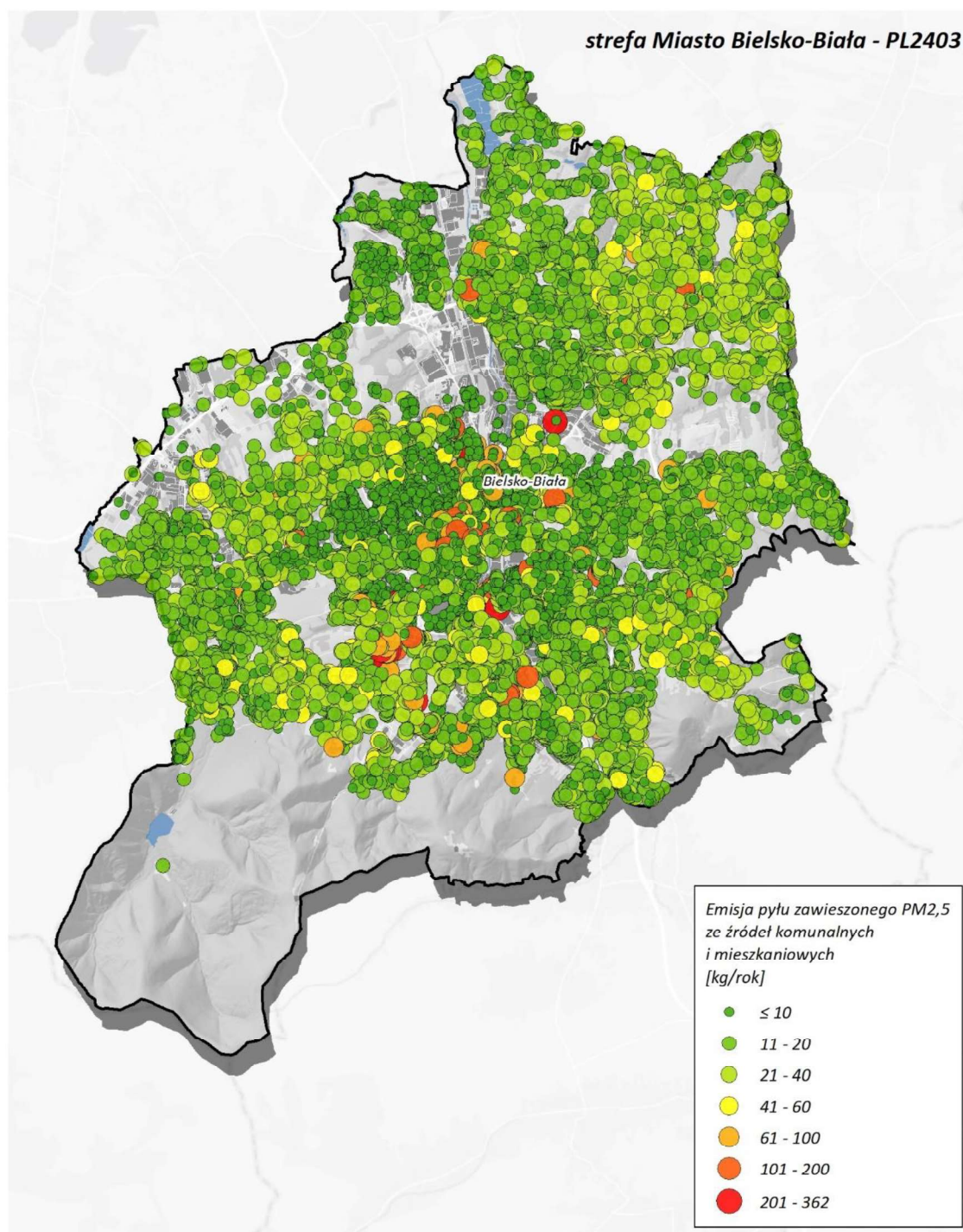
Rysunek 208. Lokalizacja i wielkość emisji pyłu PM 2,5 ze źródeł z sektora komunalno-bytowego w strefie miasto Bielsko-Biała w roku bazowym 2022 380
