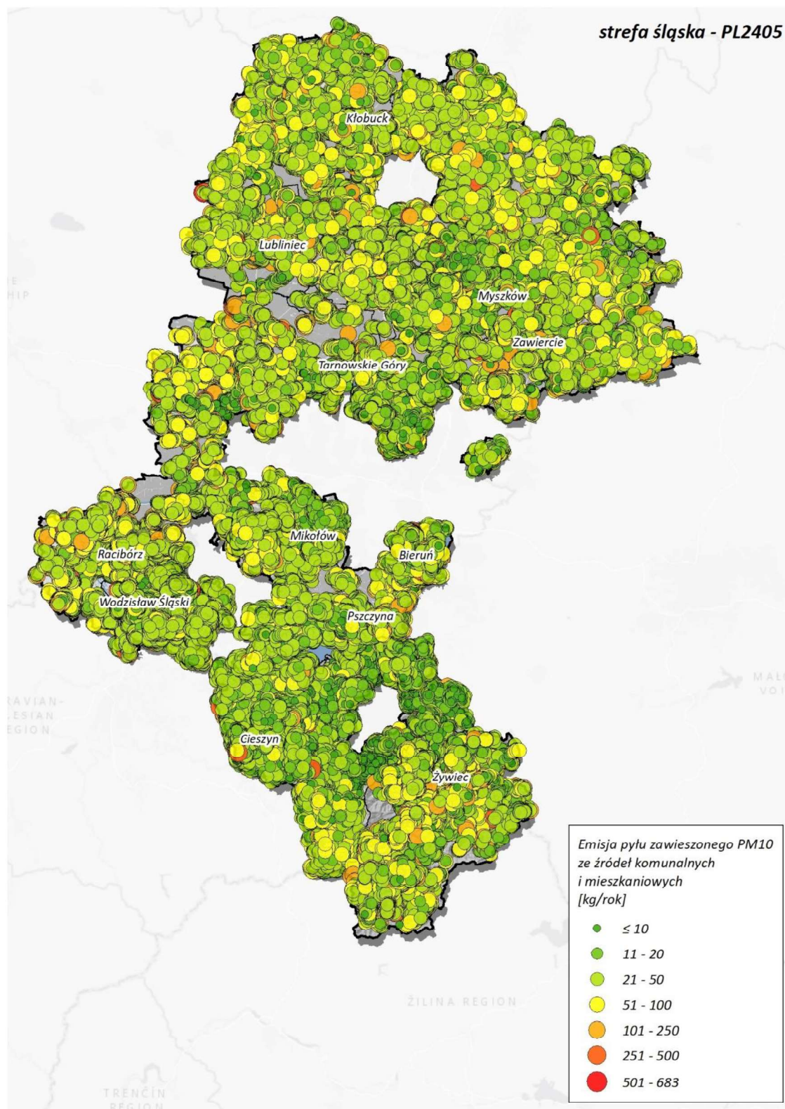
Rysunek 213. Lokalizacja i wielkość emisji pyłu PM10 ze źródeł z sektora komunalno-bytowego w strefie śląskiej w roku bazowym 2022 385
