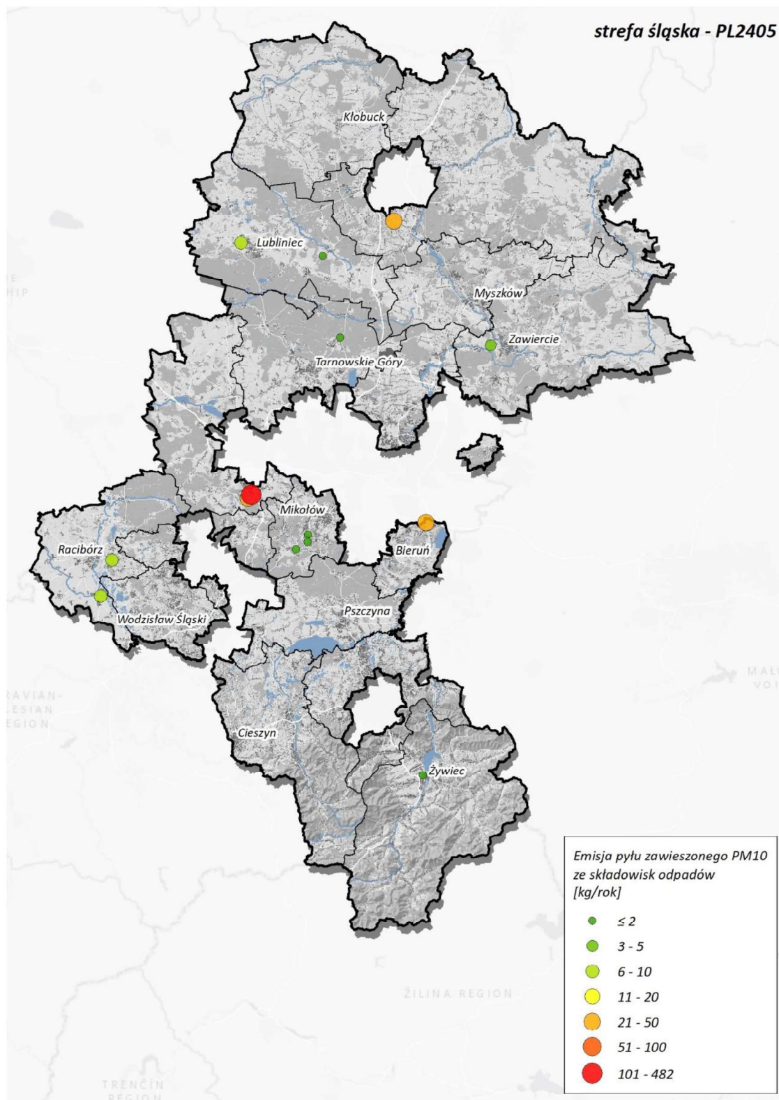
Rysunek 195. Lokalizacja i wielkość emisji pyłu PM10 ze składowisk odpadów w strefie śląskiej w roku bazowym 2022 367
