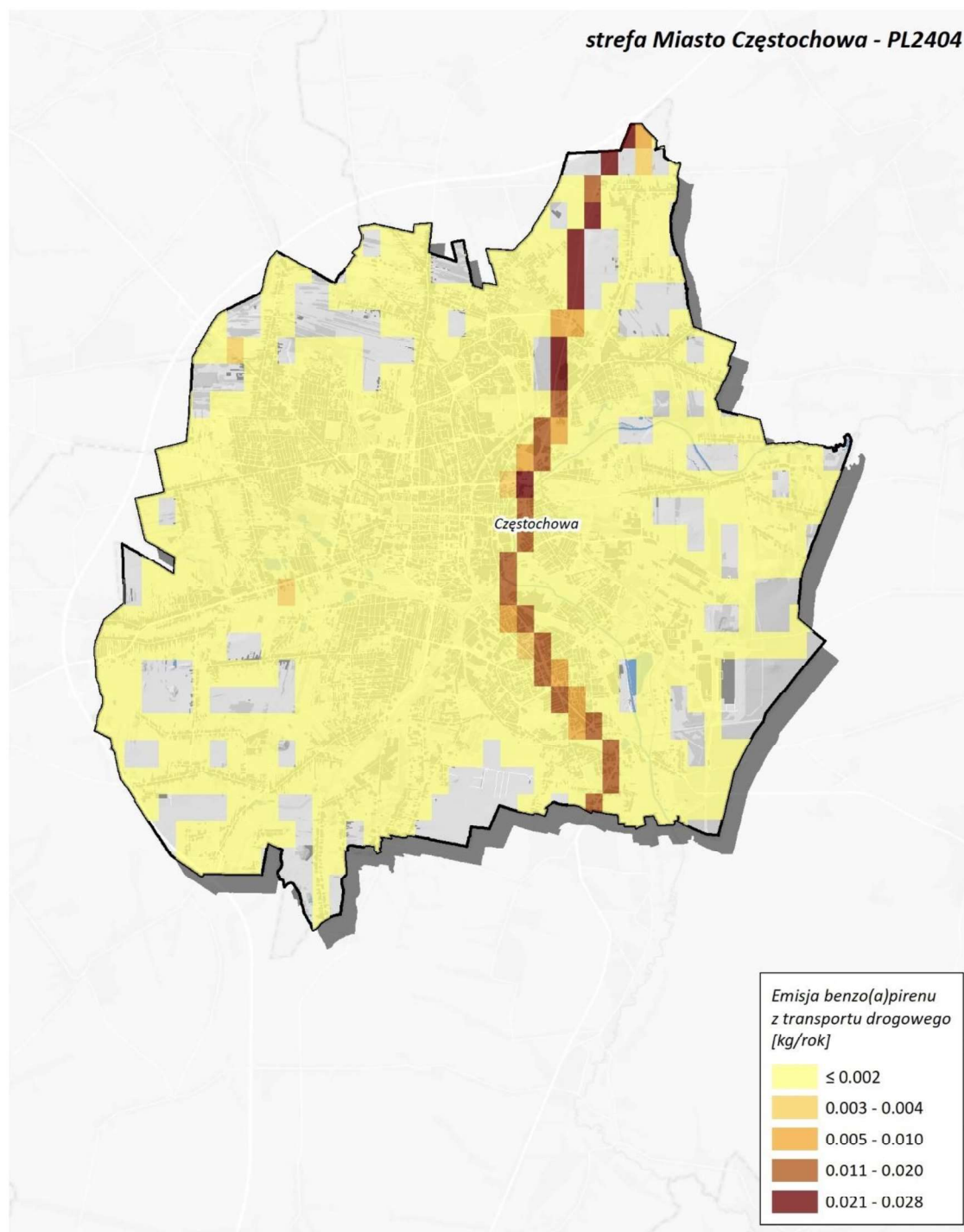
Rysunek 157. Lokalizacja i wielkość emisji B(a)P z sektora transportu drogowego w Częstochowie w roku bazowym 2022 329
