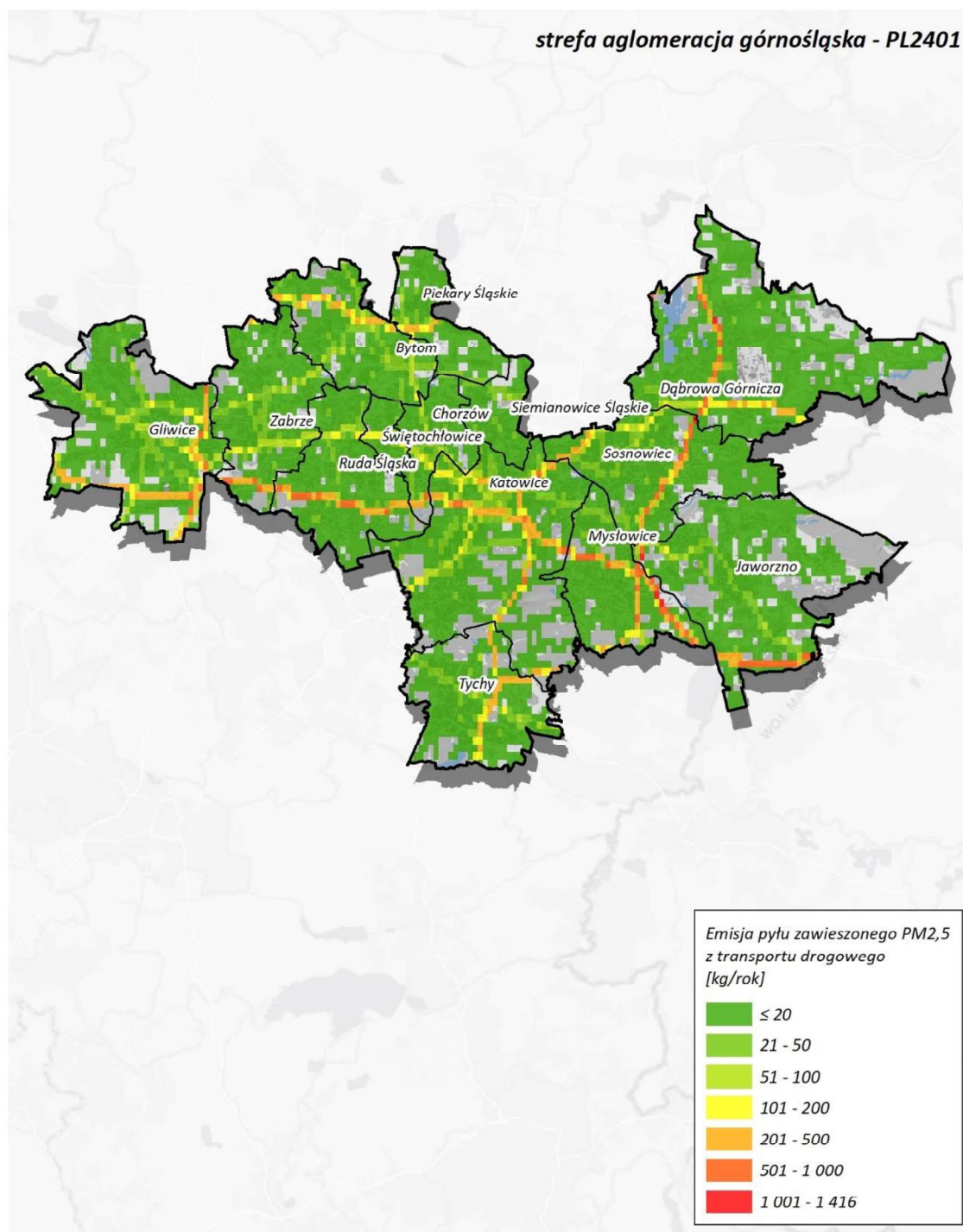
Rysunek 202. Lokalizacja i wielkość emisji pyłu PM 2,5 z sektora transportu drogowego w aglomeracji górnośląskiej w roku bazowym 2022 374
