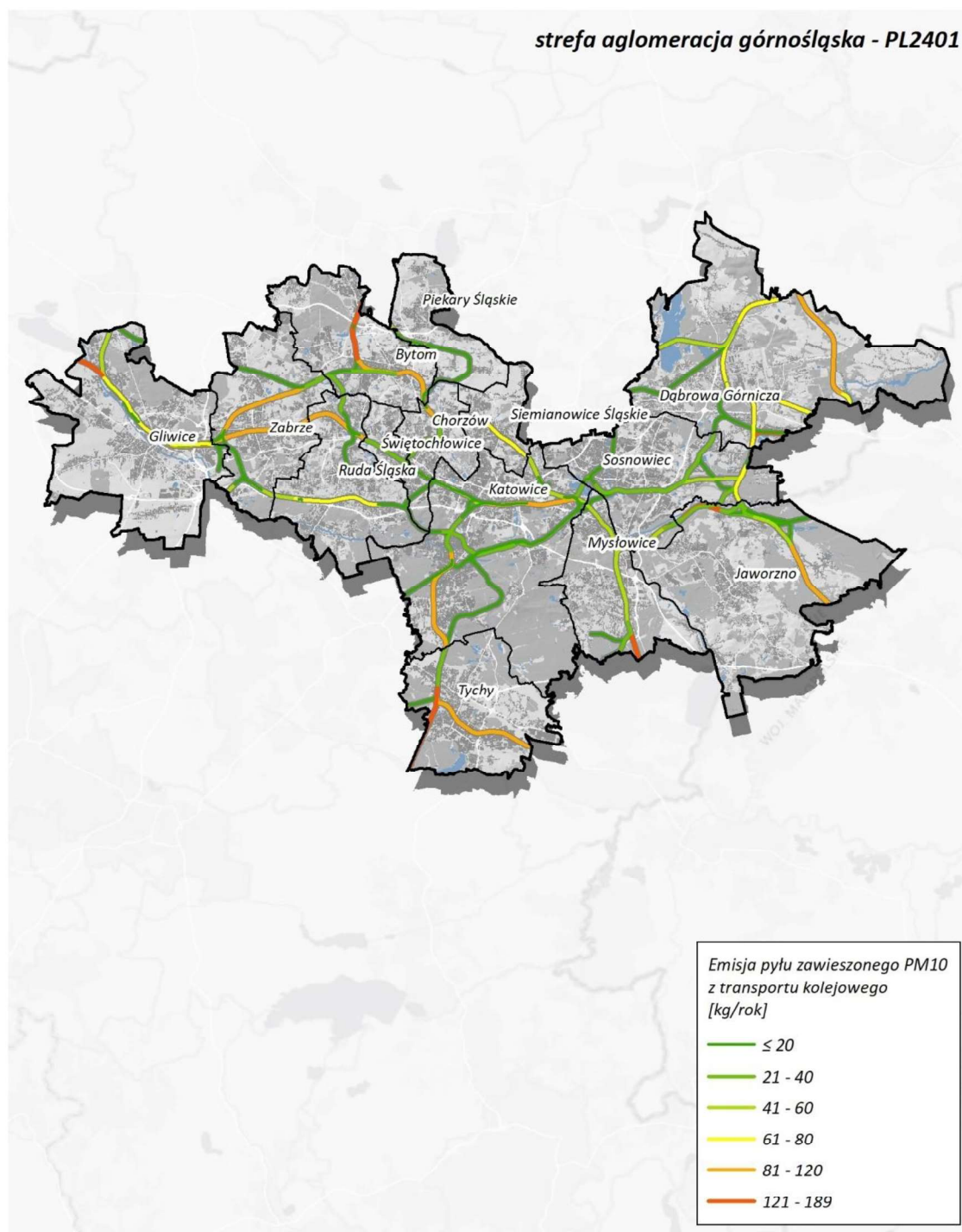
Rysunek 106. Lokalizacja i wielkość emisji pyłu PM10 z kolei w aglomeracji górnośląskiej w roku bazowym 2022 278
