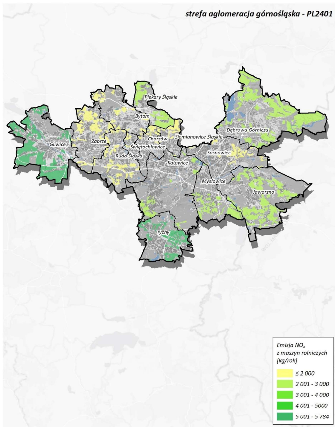
Rysunek 114. Lokalizacja i wielkość emisji NO x z maszyn rolniczych w aglomeracji górnośląskiej w roku bazowym 2022 286
