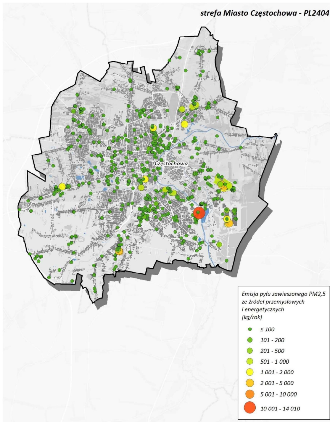
Rysunek 159. Lokalizacja i wielkość emisji pyłu PM 2,5 z przemysłu i energetyki w Częstochowie w roku bazowym 2022 331
