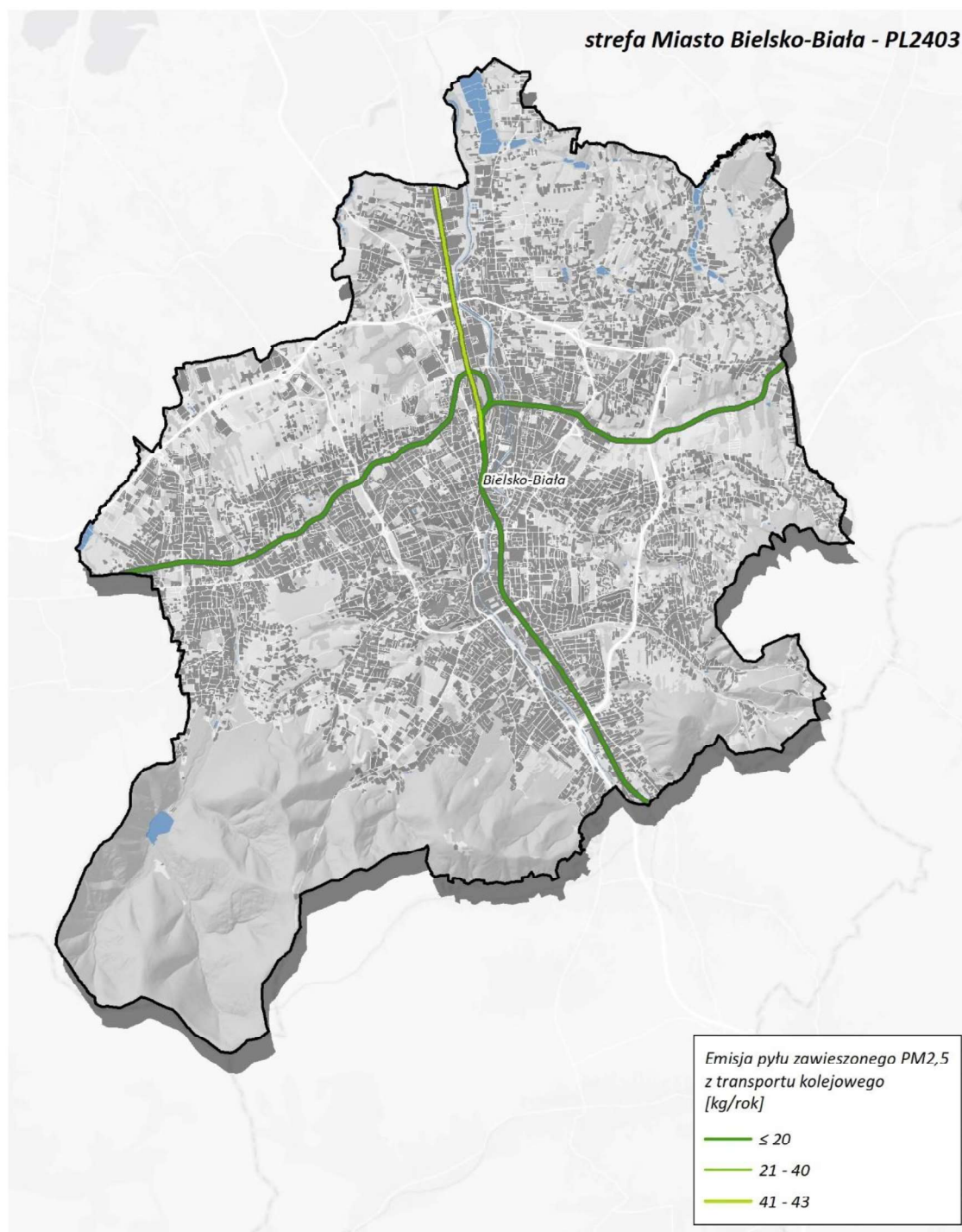
Rysunek 149. Lokalizacja i wielkość emisji pyłu PM 2,5 z kolei w Bielsku-Białej w roku bazowym 2022 321
