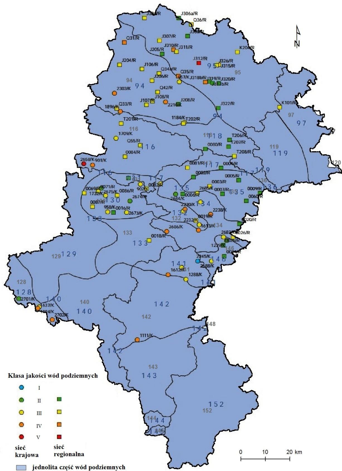
Ryc. 8. Jakość wód podziemnych województwa śląskiego w 2015 roku, w punktach monitoringu sieci regionalnej i krajowej, na tle jednolitych części wód podziemnych.
