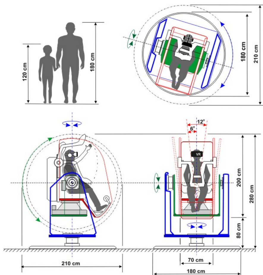
Rys. 3. Główne wymiary gabarytu oraz przestrzeni roboczej proponowanej konstrukcji stanowiska
