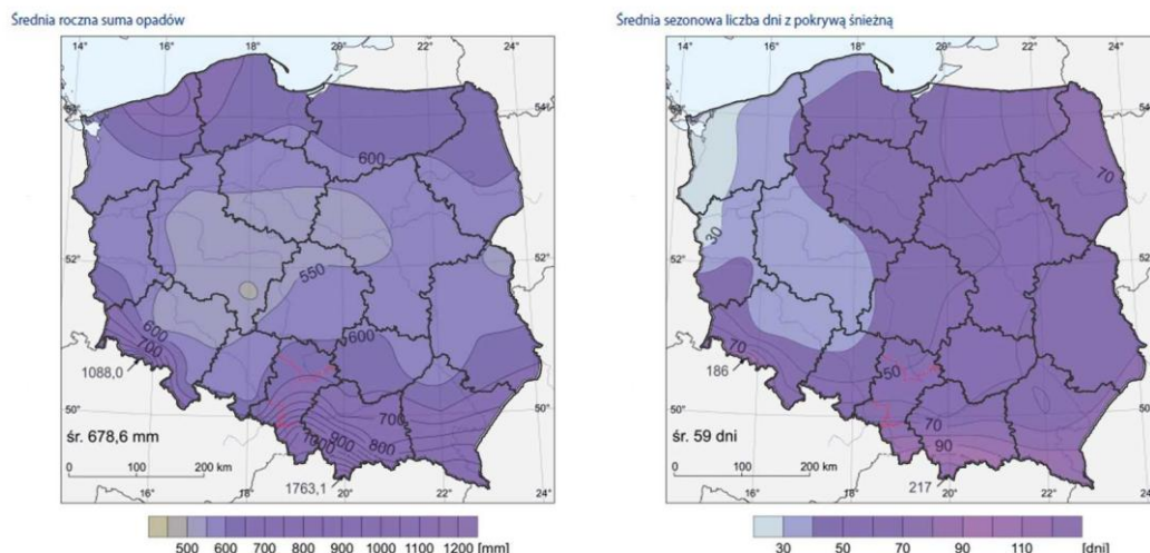
Rys. 7. Województwo na tle Polski. Średnia roczna suma opadów i średnia sezonowa liczba dni z pokrywą śnieżną
